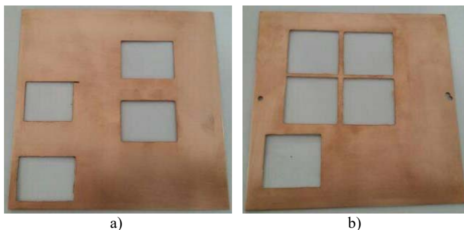
Figura 47: Placas do dielétrico após o corte das antenas em: a) h=0,64 mm b) h=1,27 mm. Fonte: Autoria Própria, 2016
