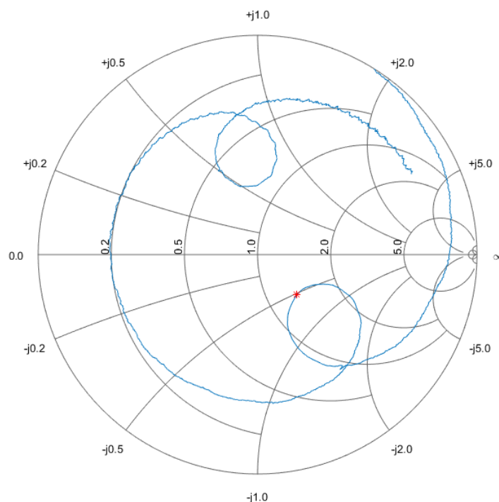
Figura 124: Curva de impedância de entrada para o dispositivo de Configuração 1, de RT/duroid 6006 h=0,64\text{ mm} , com variação no raio, em r=0,3\text{ mm} .
