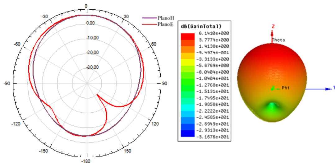
Figura 115: Diagramas de radiação 2D e 3D nos planos H e E para as configurações de RT/Duroid 6010 h=2,5 mm com variação no plano de terra em a) Sub, b) Sub+PT e c) PT. Fonte: Autoria Própria, 2015.
