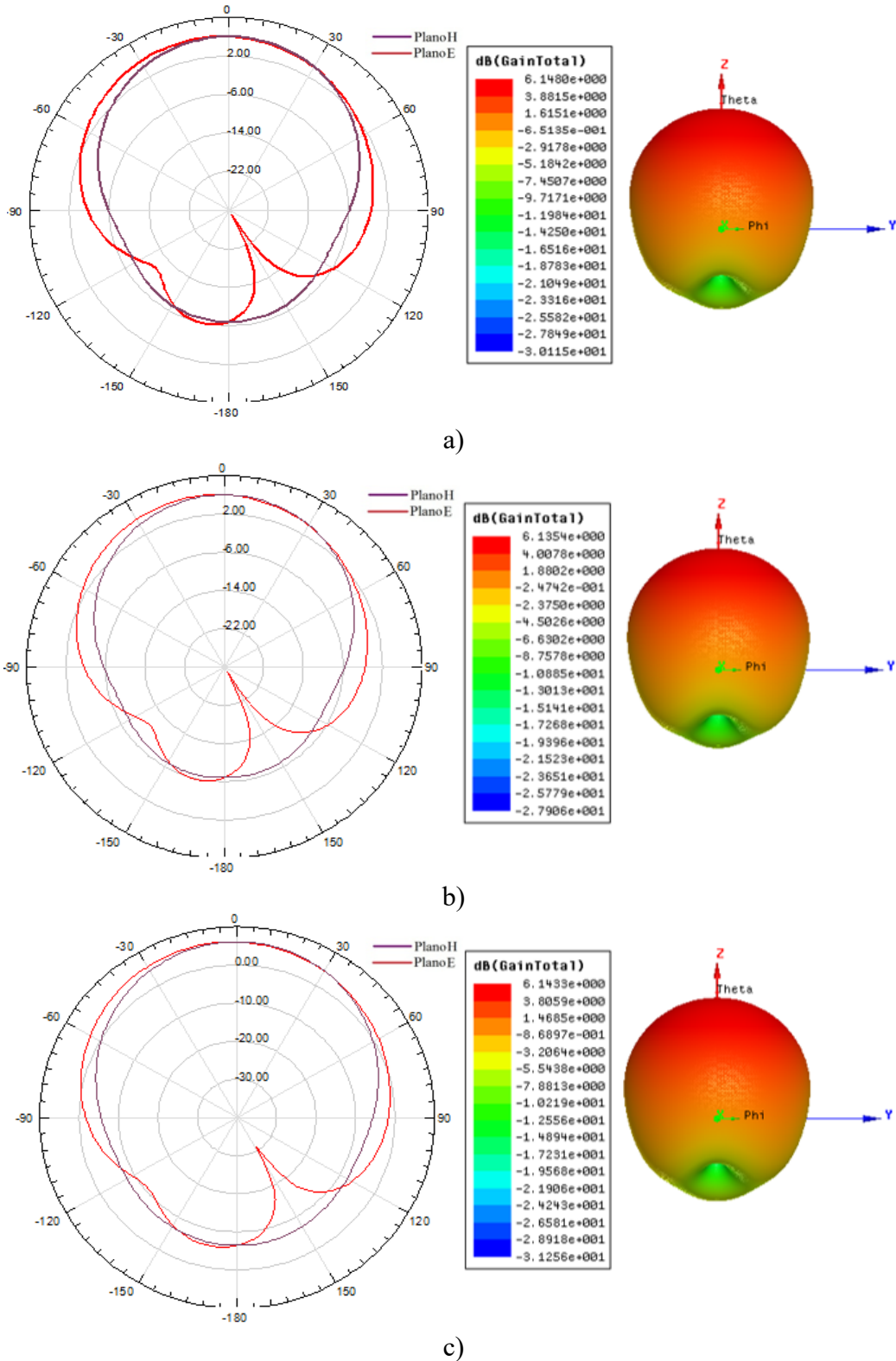
Figura 97: Diagramas de radiação 2D e 3D nos planos H e E, para substrato de RT/Duroid 6010 com h=2,5 mm por variação na altura em a) 75% b) 50% c) 25%.
