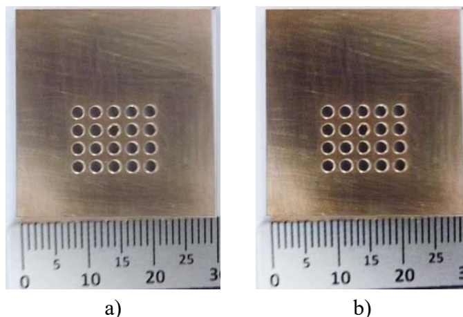
Figura 46: Estruturas perfuradas para variações nos planos de terra em: a) Configuração 3 e b) Configuração 4. Fonte: Autoria Própria, 2016.
