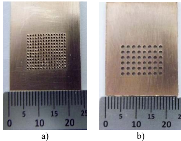
Figura 44: Estruturas perfuradas para variações no raio na: a) Configuração 1 e b) Configuração 2.
