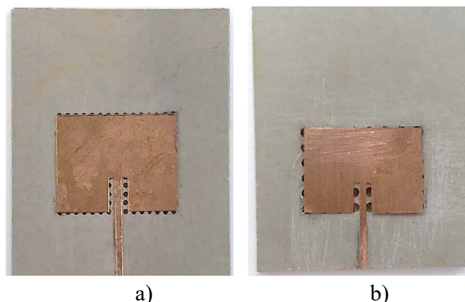
Figura 53: Estruturas com patches para as variações no raio em: a) Configuração 1 e b) Configuração 2.
