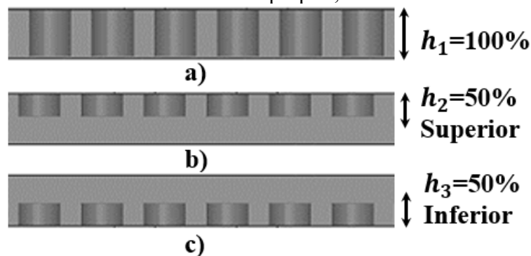
Figura 37: Variação da profundidade dos cilindros da estrutura EBG/PBG em a) 100% b) 50% Superior c) 50% Inferior.
