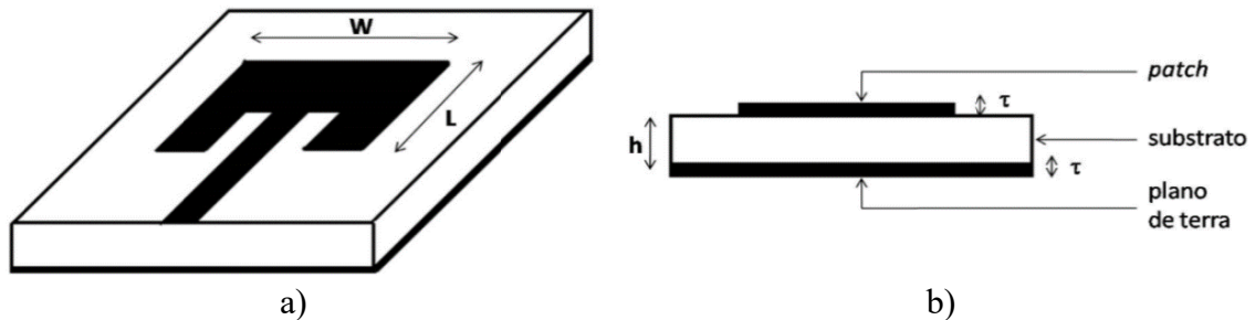
Figura 3: Antena alimentada por linha de microfita. Fonte: Adaptado do BALANIS, 2005.
