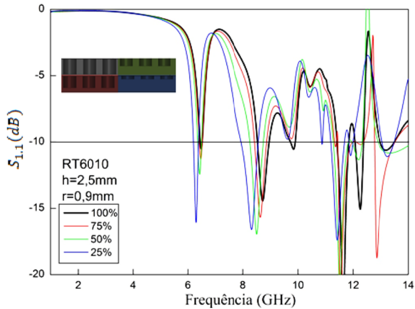
Figura 86: Perdas de retorno em função da frequência para as configurações com variação na altura em RT/Duroid 6010 com h=2,5 mm.
