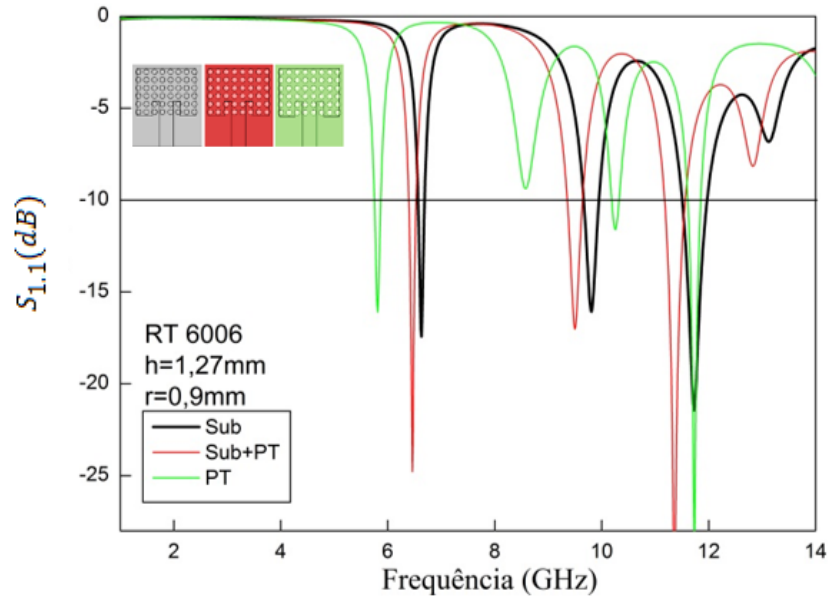
Figura 106: Perdas de retorno em função da frequência para as configurações com variação no plano de terra no dielétrico de RT/Duroid 6006 com h=1,27 mm.
