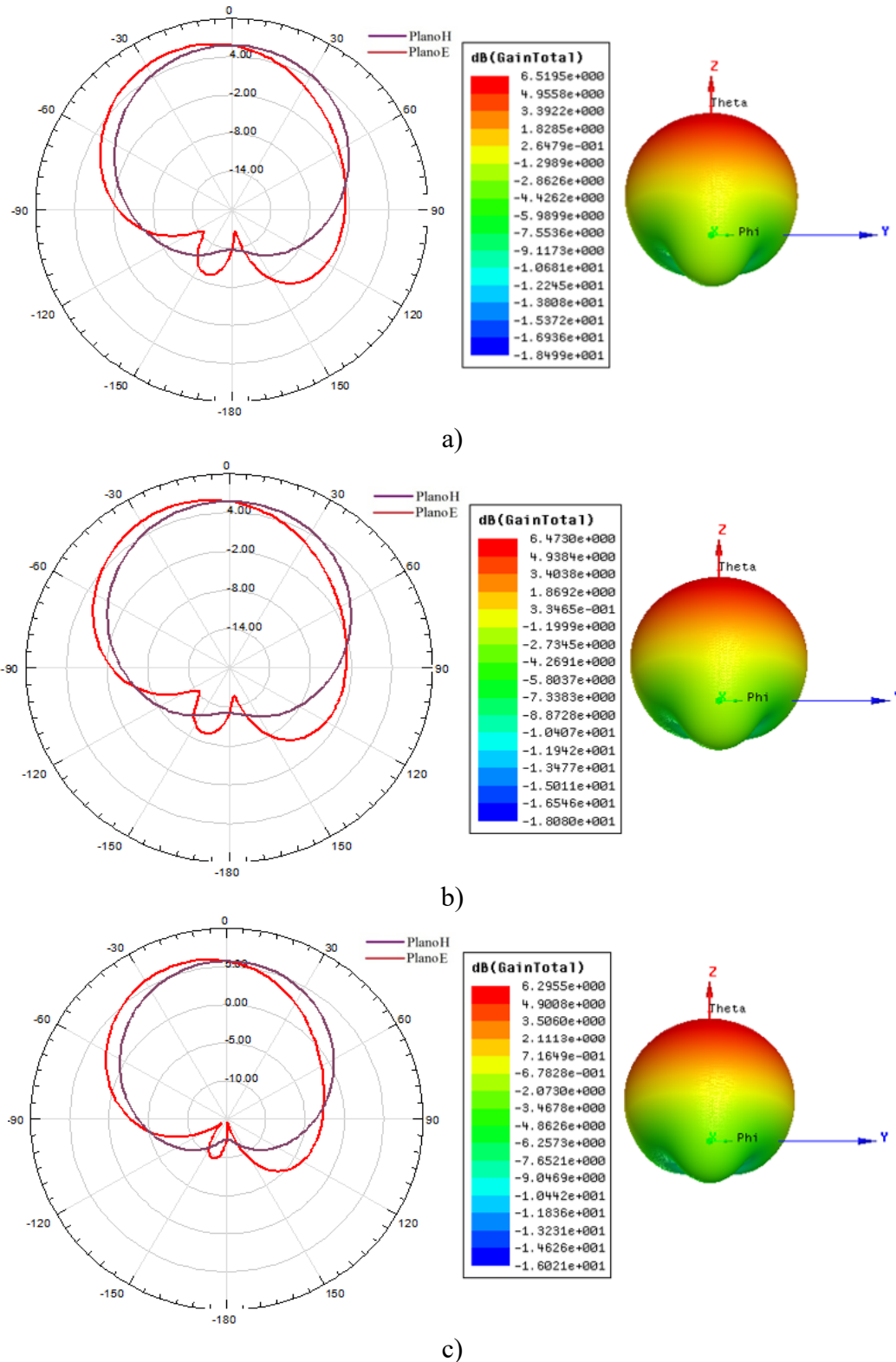
Figura 94: Diagramas de radiação 2D e 3D nos planos H e E, para o substrato de RT/Duroid 6006 com h=0,64 mm para variação na altura em a) 75% b) 50% c) 25%.
