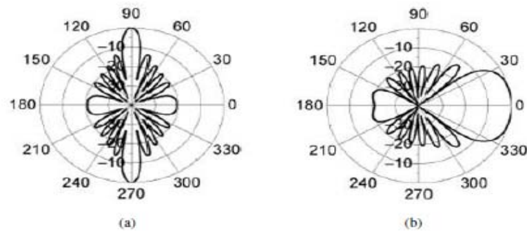
Figura 17: Diagrama de radiação a) Broadside b) end-fire.
