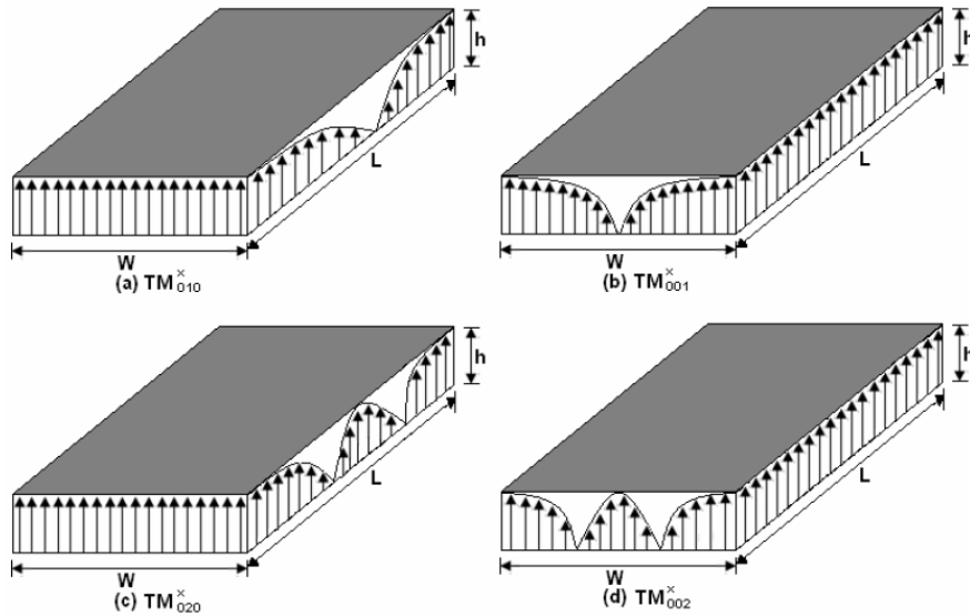
Figura 13: Configurações de campo (modos) para patch retangular de microfita.
