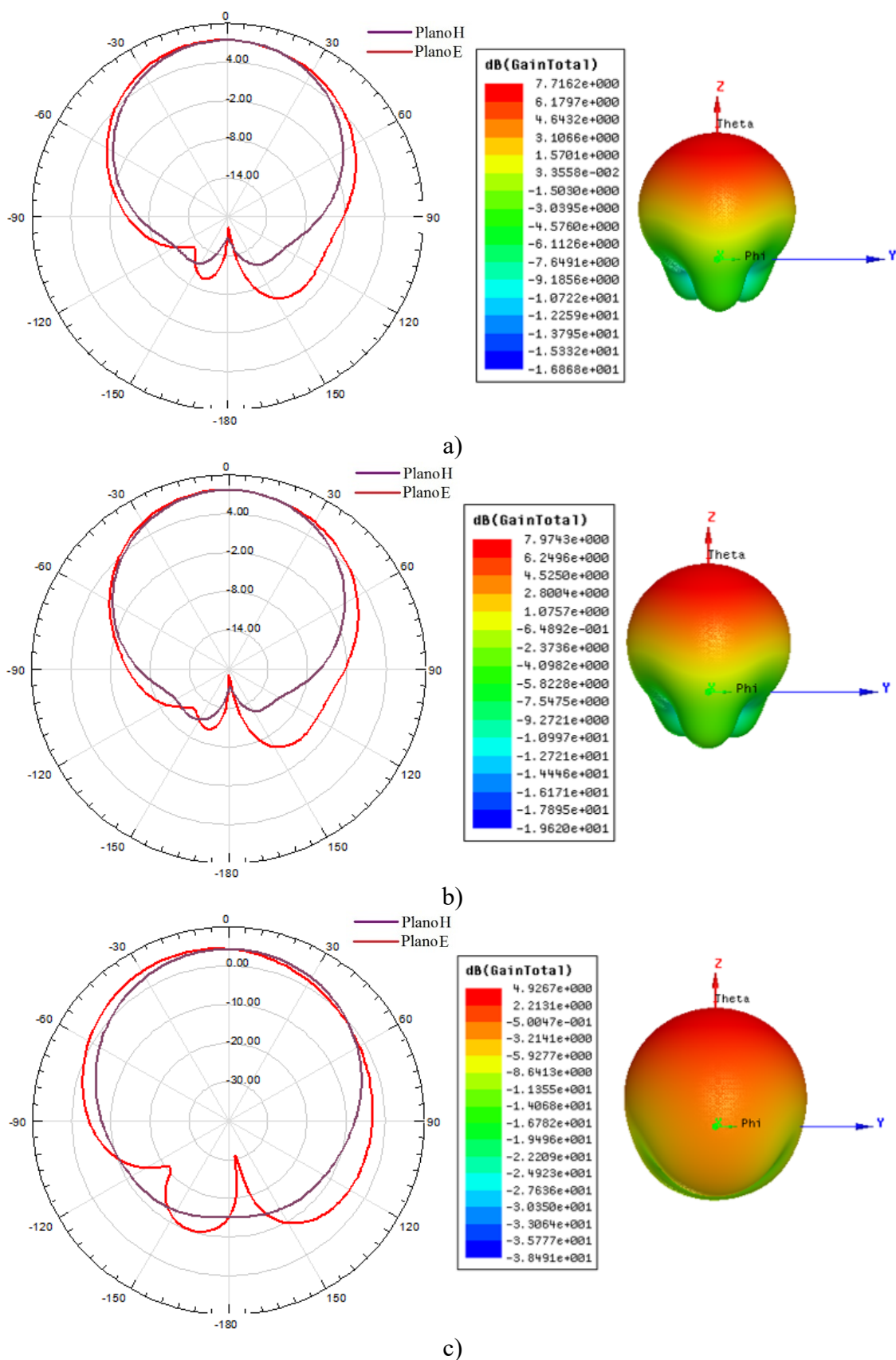
Figura 63: Diagramas de radiação 2D e 3D nos planos H e E, para as antenas padrão em: a) Configuração 1 b) Configuração 2 e c) Configuração 3.
