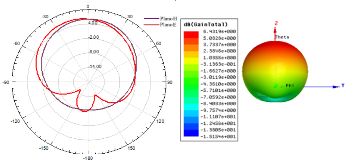
Figura 99: Diagramas de radiação 2D e 3D nos planos H e E, para as configurações com substrato de RT/Duroid 6006 com 2h=2,54 mm para variação na altura do cilindro em a) 100% b) 50% Superior c) 50% Inferior.
