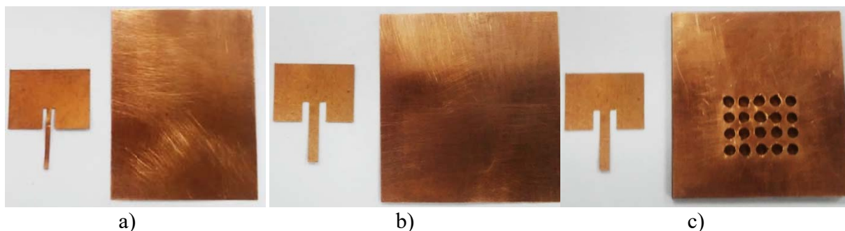
Figura 48: Configurações dos Patches e Planos de terra confeccionados para estruturas com variações em a) Raios b) Alturas c) Plano de terra.
