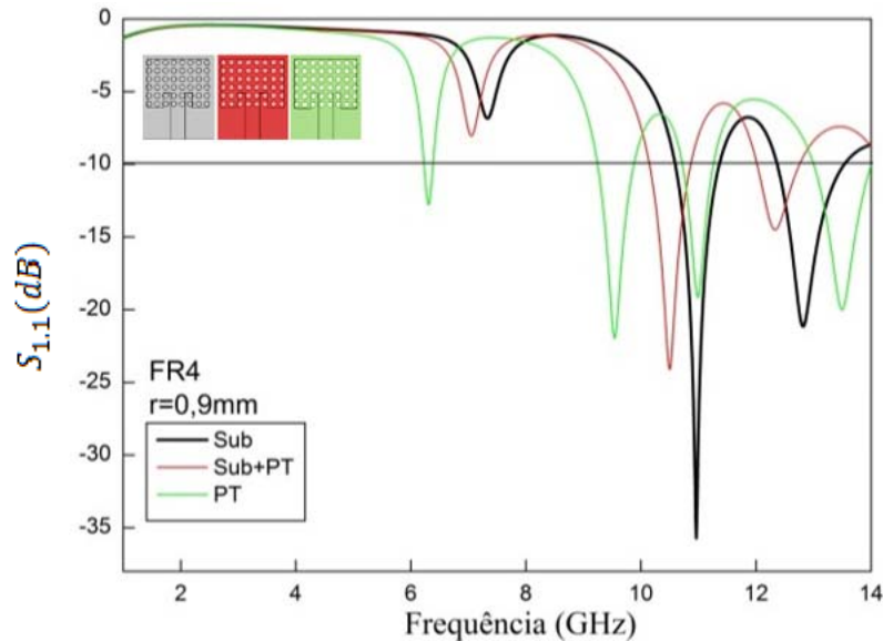
Figura 104: Perdas de retorno em função da frequência para as configurações com variação no plano de terra no dielétrico de FR4.
