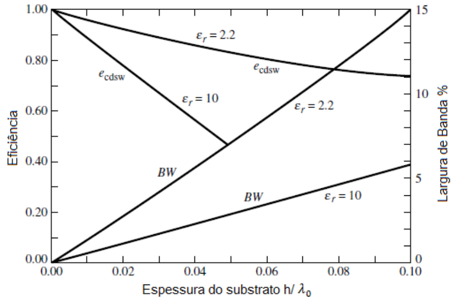
Figura 23: Efeitos da espessura do substrato e da constante dielétrica na largura de banda e eficiência para substratos diferentes de uma antena. Fonte: POZAR, 1992.
