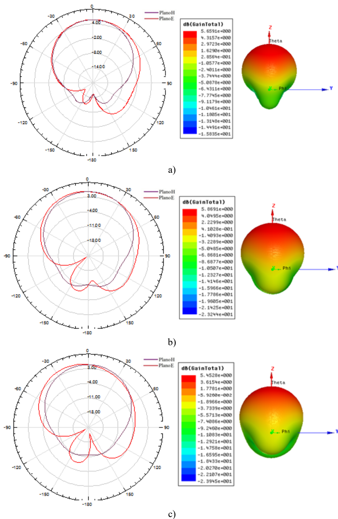
Figura 111: Diagramas de radiação 2D e 3D nos planos H e E para as configurações de FR4 com variação no plano de terra em a) Sub, b) Sub+PT e c) PT.
