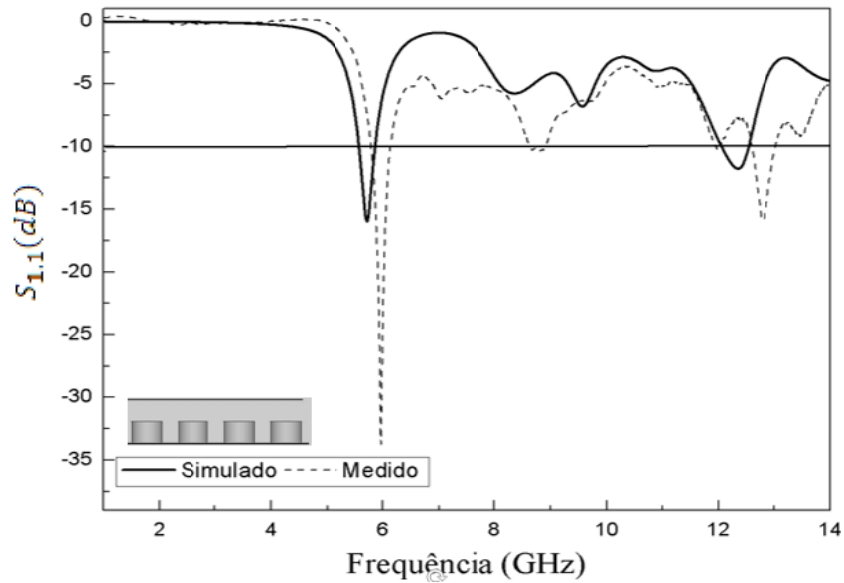
Figura 121: Comparação dos valores simulados e medidos para perda de retorno em função da frequência para a Configuração 3 de variação na altura em 50% Inferior.
