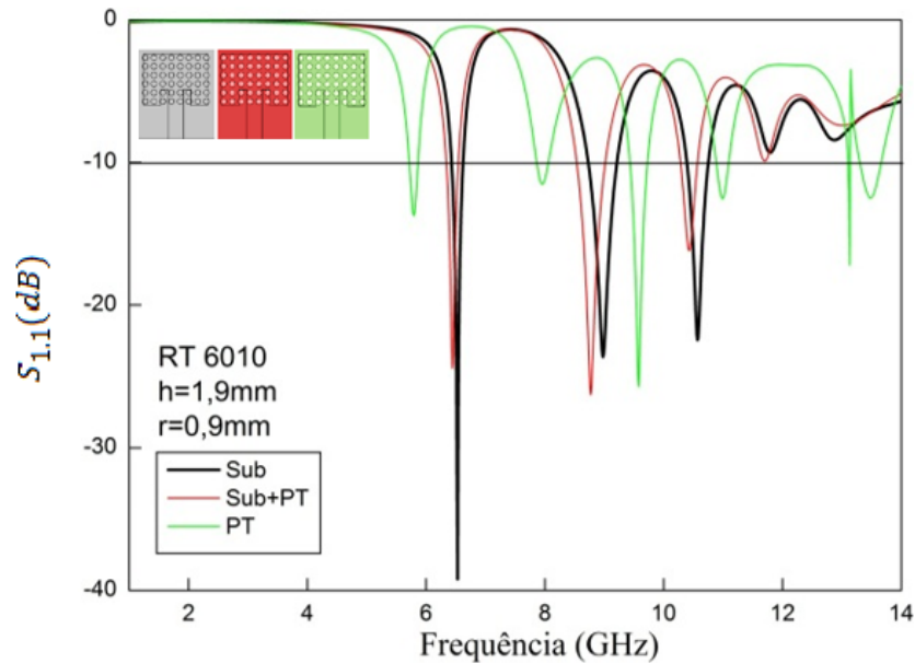
Figura 107: Perdas de retorno em função da frequência para as configurações com variação no plano de terra no dielétrico de RT/Duroid 6010 com h=1,9 mm.
