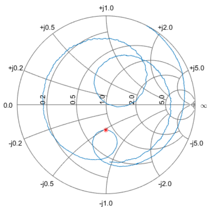
Figura 125: Curva de impedância de entrada para o dispositivo de Configuração 2, de RT/duroid 6006 h=0,64 mm, com variação no raio, em r=0,6 mm.
