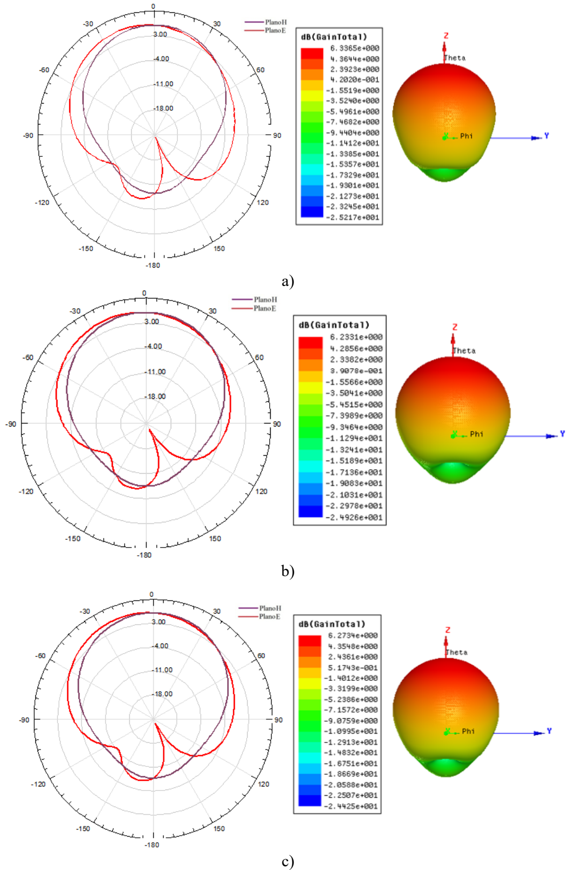
Figura 78: Diagramas de radiação 2D e 3D nos planos H e E, para o RT/Duroid 6010 com h=1.9 mm com variação no raio em a) r=0.3 mm b) r=0.6 mm c) r=0.9 mm.
