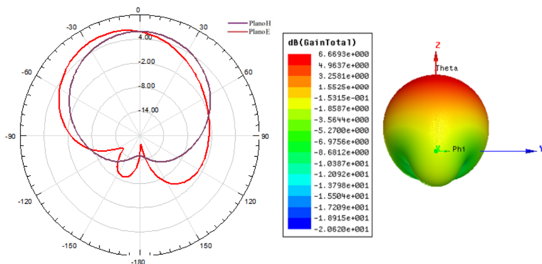
Figura 76: Diagramas de radiação 2D e 3D nos planos H e E, para oRT/Duroid 6006 com h=0,64 mm com variação no raio em a) r=0,3 mm b) r=0,6 mm c) r=0,9 mm.
