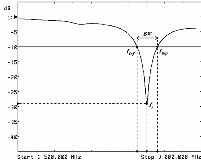
Figura 22: Gráfico da perda de retorno em função da frequência. Fonte: CARNEIRO, 2010.
