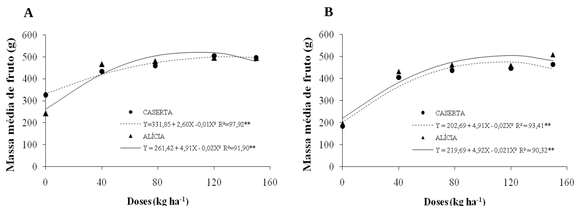
Figura 3 – Massa média de fruto de abobrinha italiana, em função de doses de fósforo, cultivo de agosto a novembro de 2015 (A) e de julho a setembro de 2016 (B), das cultivares Caserta (●) e Alícia (▲). Mossoró-RN, 2016.
