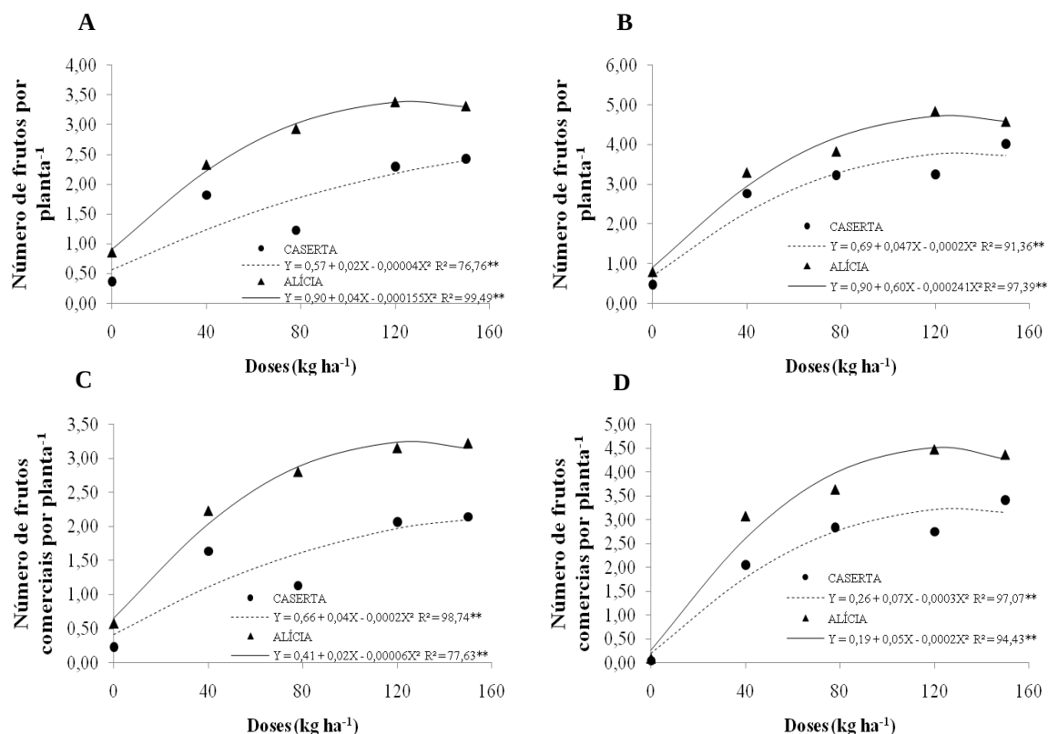
Figura 4 - Número de frutos por planta de abobrinha italiana, em função de doses de fósforo, cultivo de agosto a novembro de 2015 (A) e de julho a setembro de 2016 (B), e número de frutos comerciais por planta, cultivo de agosto a novembro de 2015 (C) e de julho a setembro de 2016, (D), das cultivares Caserta (●) e Alícia (▲). Mossoró-RN, 2016.
