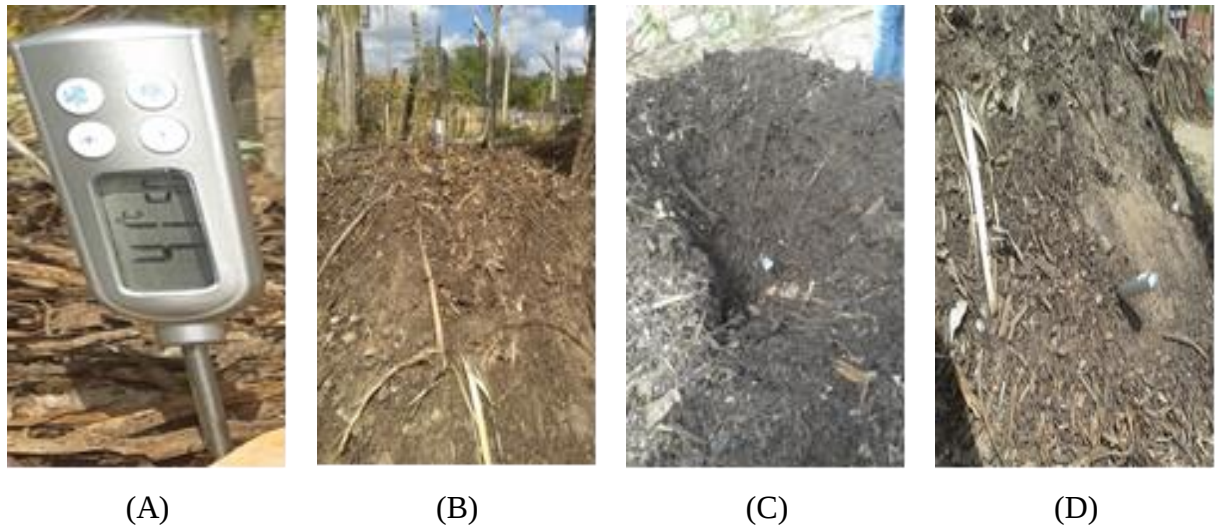
Figura 14 – Monitoramento da temperatura: termômetro digital (A); topo (B); centro (C); e base (D).
