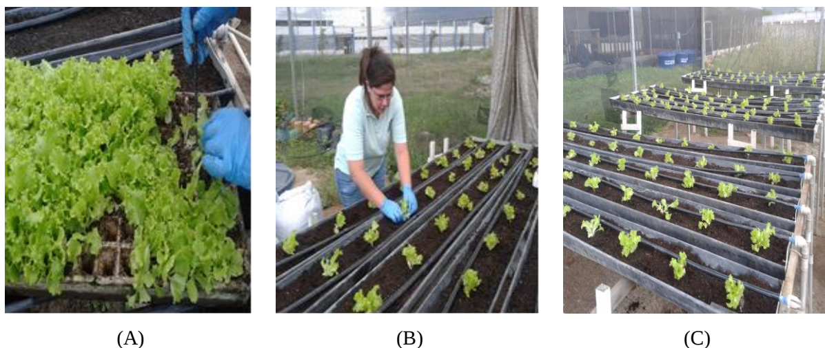
Figura 20 – Transplântio das mudas de alface nas canaletas de PVC.
