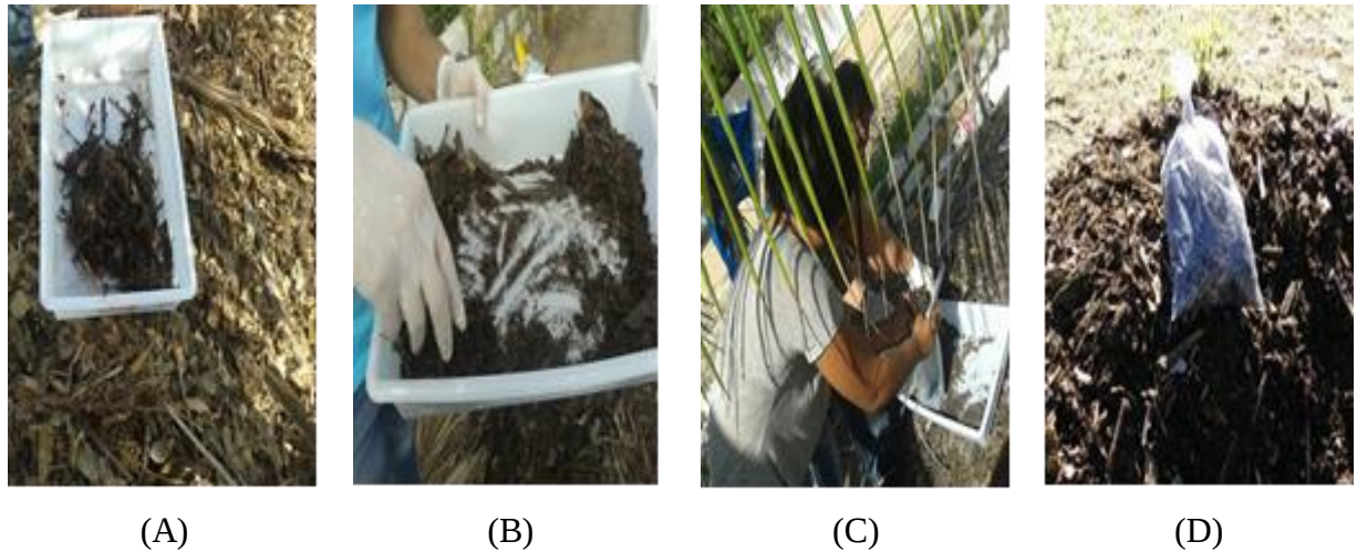
Figura 12 – Amostragem do composto pelo método de quartejamento da NBR10007/2004.
