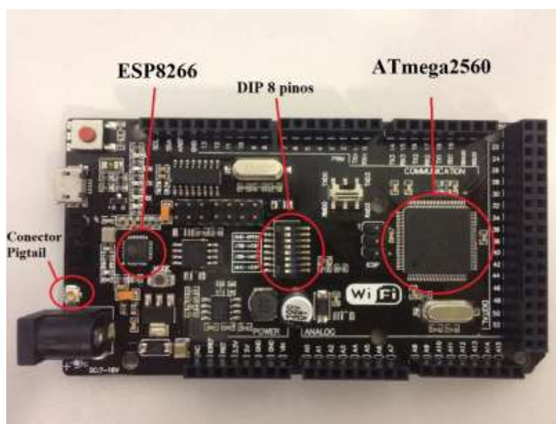
Figura 27: Placa wemos Atmega2560 wifi
