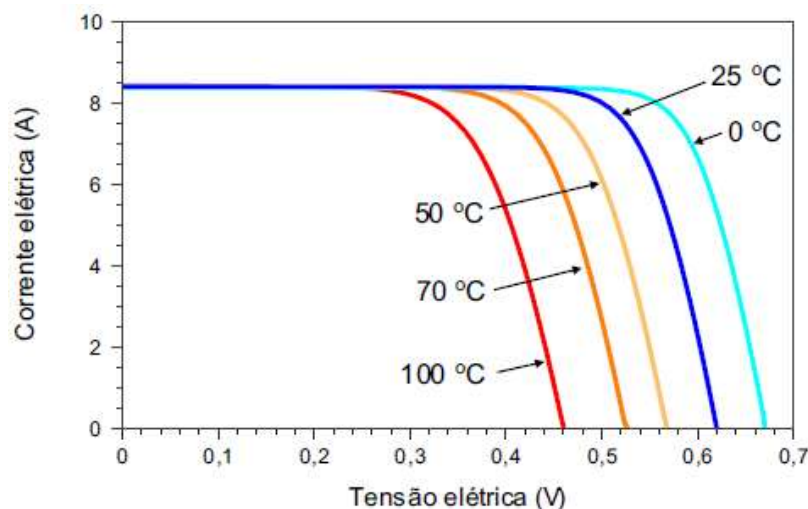
Figura 8: Influência da temperatura da célula fotovoltaica na curva I-V
