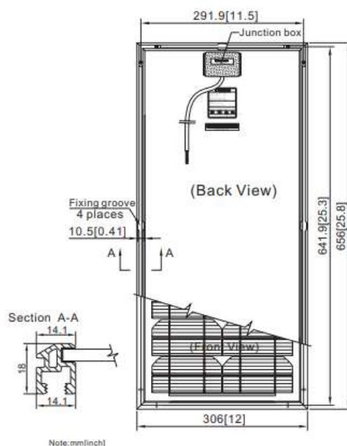
Figura 43: Dimensões do painel fotovoltaico
