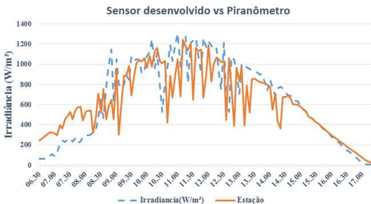
Figura 55: Comparativo entre a irradiância solar do sensor desenvolvido e o piranômetro
