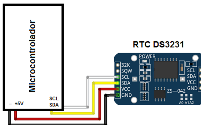
Figura 33: Montagem do módulo RTC DS3231
