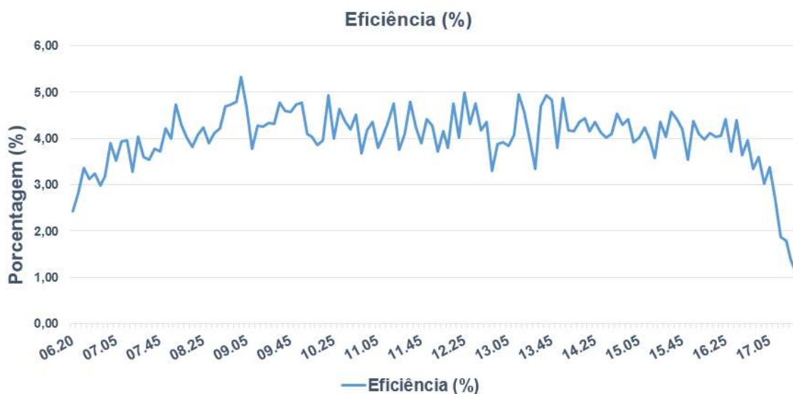
Figura 57: Eficiência obtida pelo dispositivo
