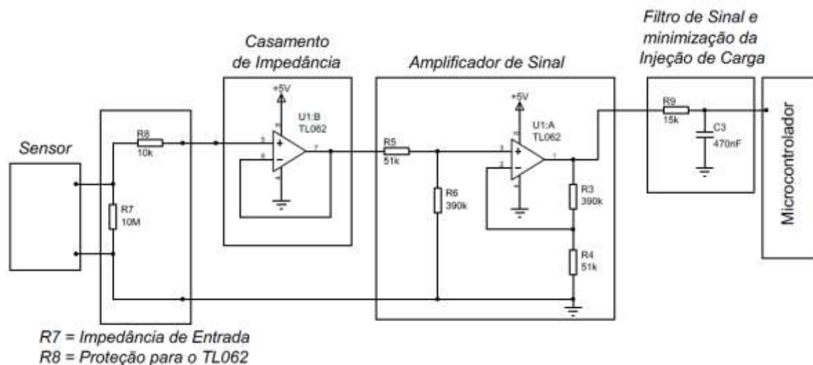
Figura 25: Circuito condicionador de sinal para linearização do sinal
