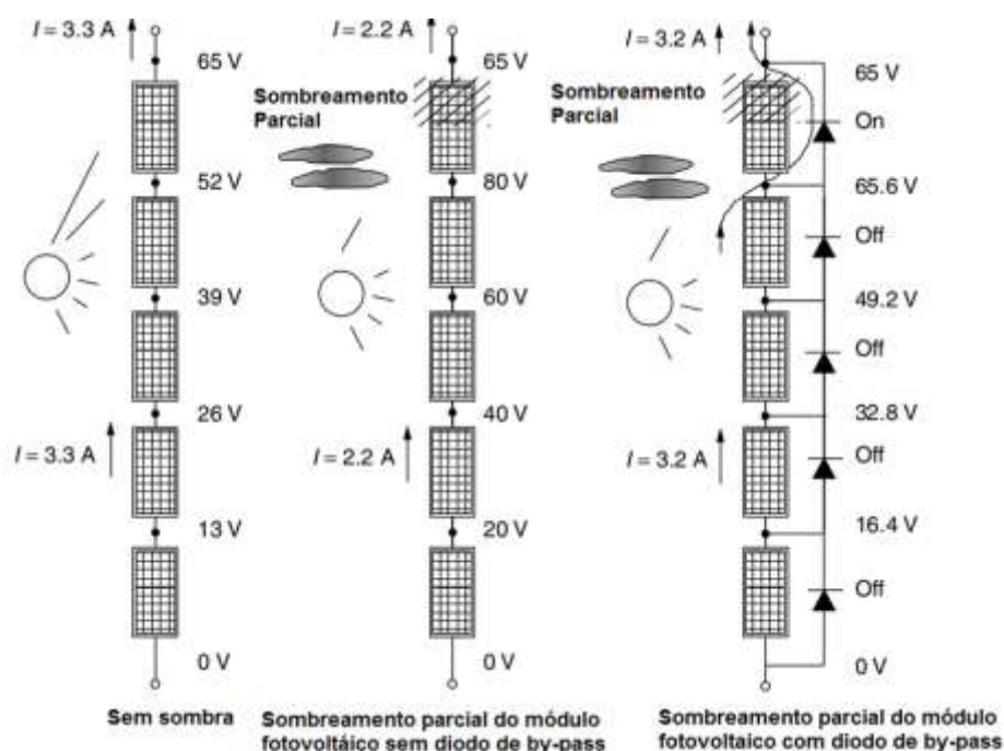
Figura 6: Proteção contra corrente reversa (diodo by-pass)
