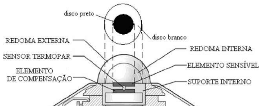
Figura 21: Esboço de um piranômetro
