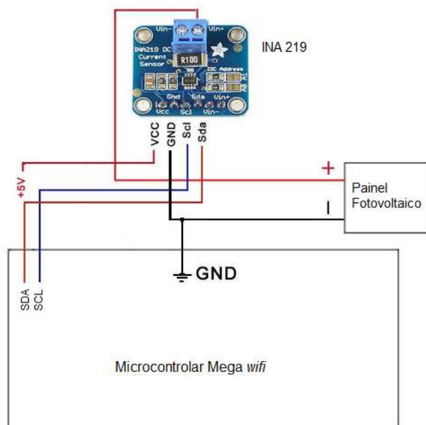
Figura 29: Ligação do sensor INA219
