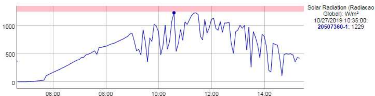
Figura 23: Representação de um dia de irradiância solar acima do normal
