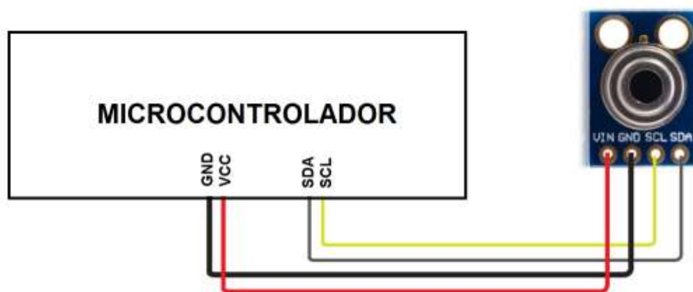
Figura 31: Sensor de temperatura infravermelho mlx90614
