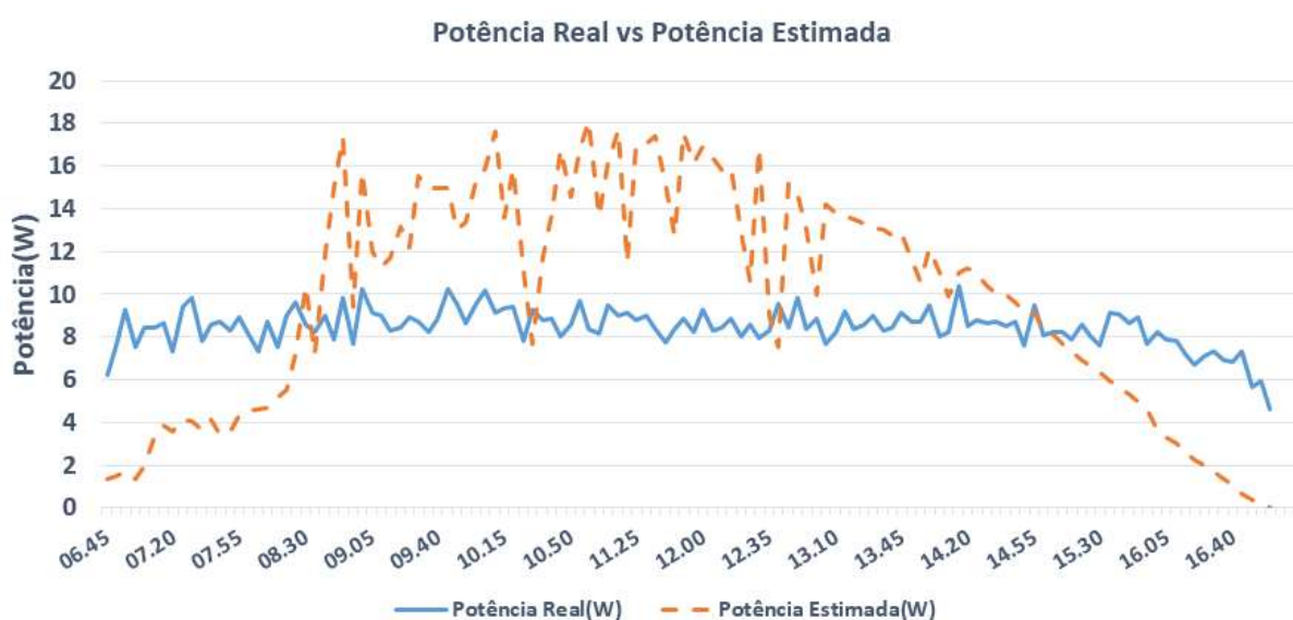
Figura 62: Comparação entre a potência estimada e a potência real
