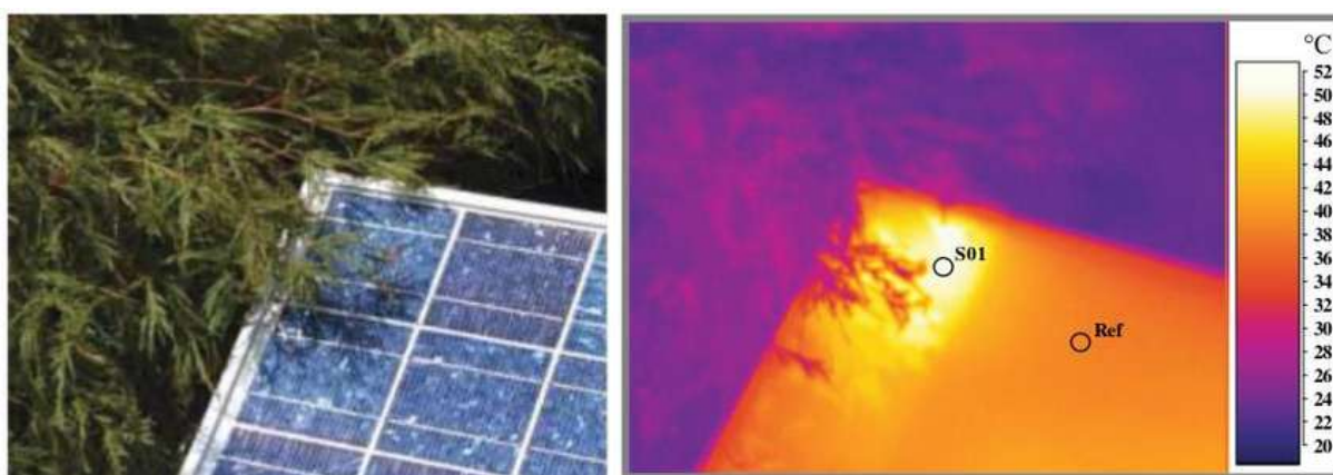
Figura 5: Efeito do Sombreamento
