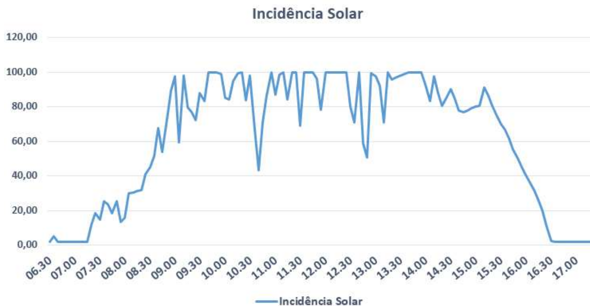
Figura 60: Incidência solar sobre a superfície do painel
