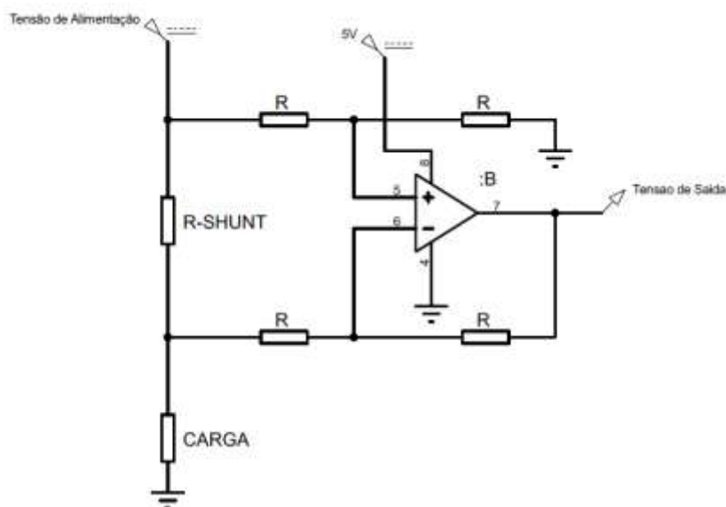
Figura 28: Método de medição High-side
