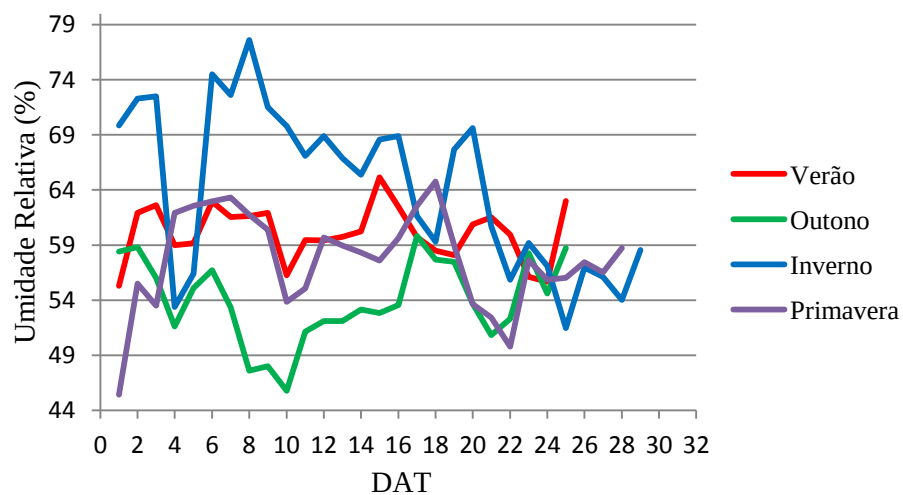
Figura 4 – Umidade Relativa média do ar durante a condução do experimento, dias após o transplântio (DAT), nas quatro épocas de plantio. Mossoró-RN, 2013.
