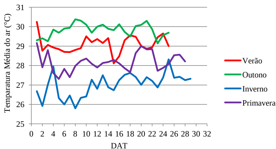
Figura 2- Temperatura média do ar durante a condução do experimento, dias após o transplântio (DAT), nas quatro épocas de plantio. Mossoró-RN, 2013.
