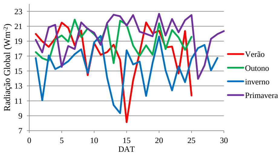
Figura 5 – Radiação Global (Wm -2 ) durante a condução do experimento, dias após o transplântio (DAT), nas quatro épocas de plantio. Mossoró-RN, 2013.
