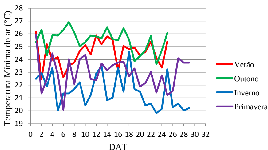
Figura 1- Temperatura mínima do ar durante a condução do experimento, dias após o transplântio (DAT), nas quatro épocas de plantio. Mossoró-RN, 2013.
