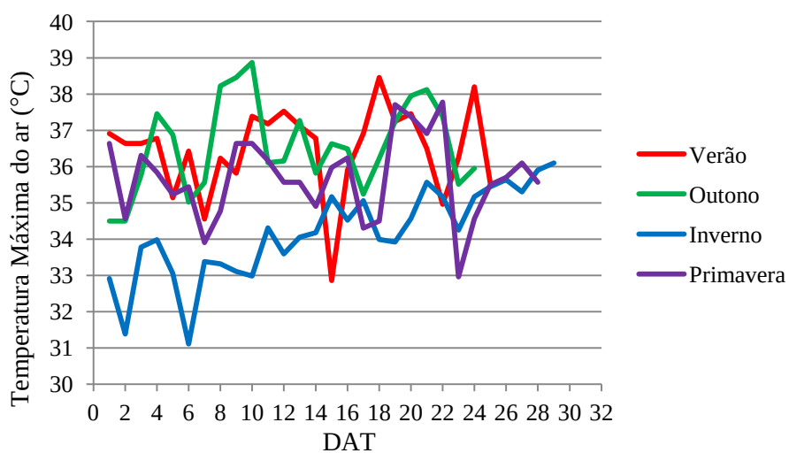
Figura 3- Temperatura máxima do ar durante a condução do experimento, dias após o transplântio (DAT), nas quatro épocas de plantio. Mossoró-RN, 2013.
