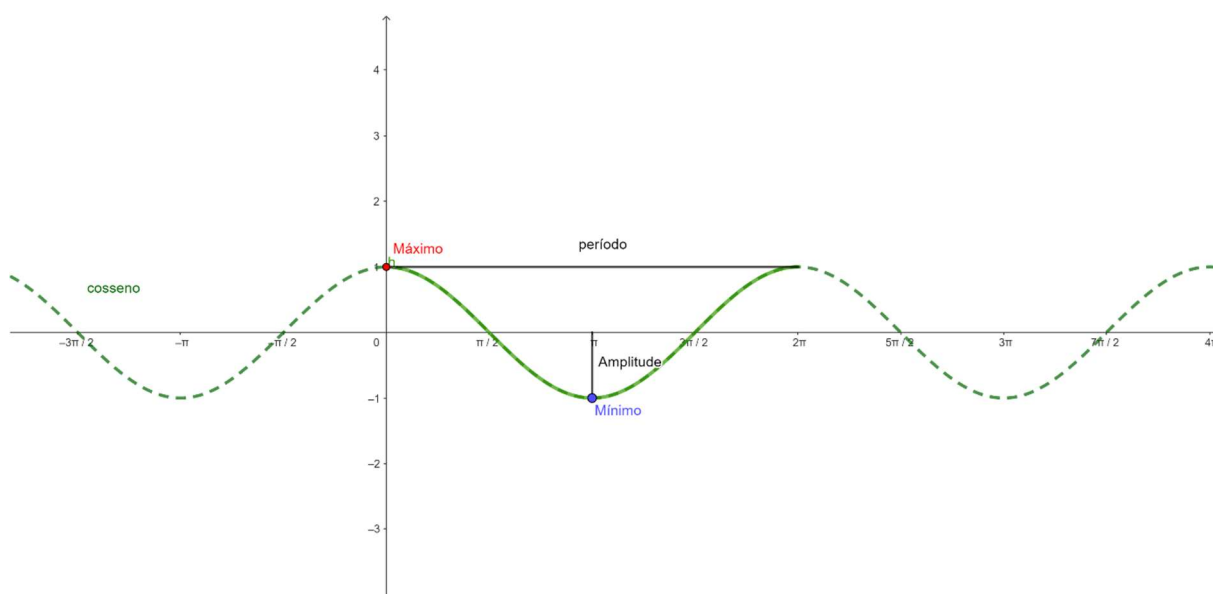
Gráfico 3. Função cosseno.
