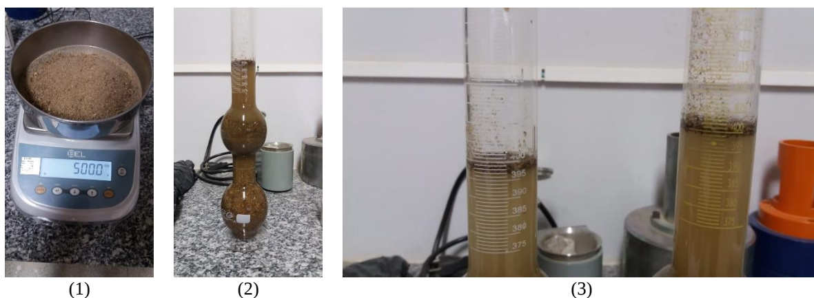
Figura 6 – Massa espec3fica por meio do frasco de Chapman: (1) Amostra de 500 gramas; (2) Frasco contendo 3gua (200 ml) e agregado mi3do e (3) faz-se a leitura.
