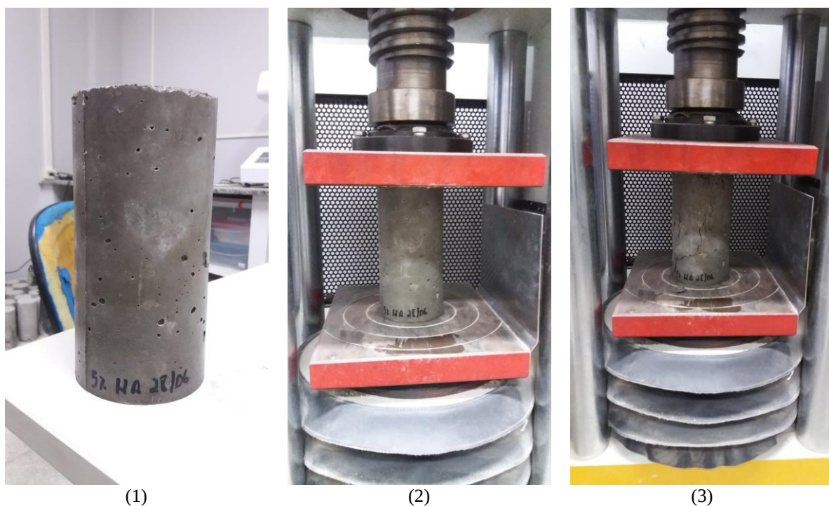
Figura 12 – Ensaio de resistência à compressão.
