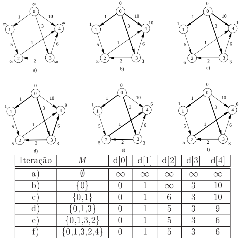
Figura 1.8: Exemplo de execução do algoritmo de Dijkstra Fonte: (ALMEIDA; ZIVIANI, 2004)
