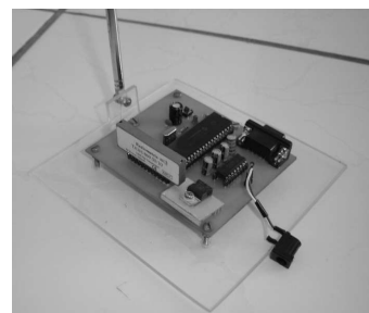
b)Placa transmissora
