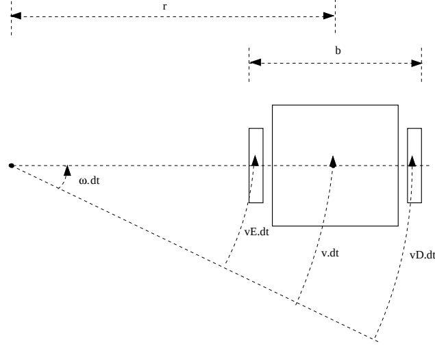
Figura B.2: Velocidades para movimentos infinitesimais Fonte: (ALSINA, 2001)
