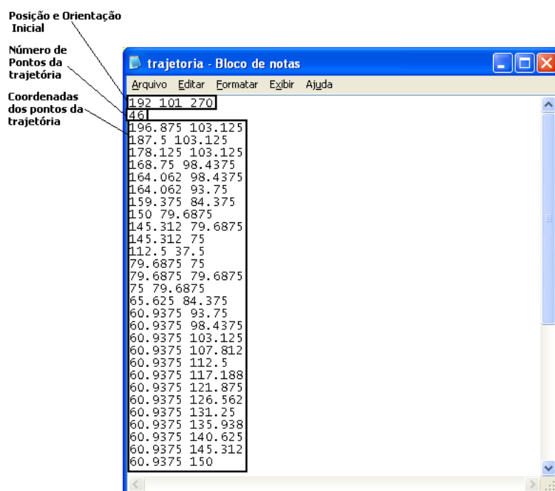
Figura 2.19: Detalhe do arquivo de saída “Trajetoria.txt”
