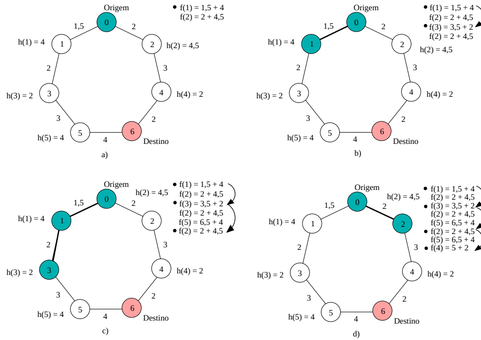
Figura 1.9: Exemplo de execução do algoritmo A-Estrela
