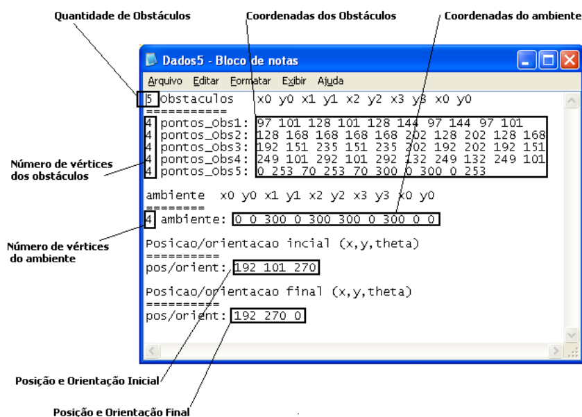
Figura 2.18: Detalhe do arquivo de entrada “Dados.txt”
