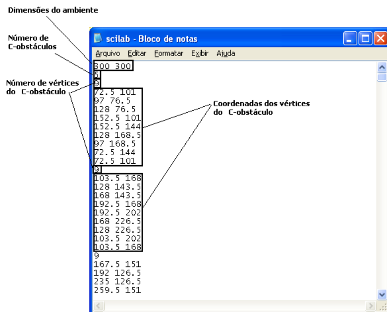
Figura 2.20: Detalhe do arquivo de saída “Scilab.txt”
