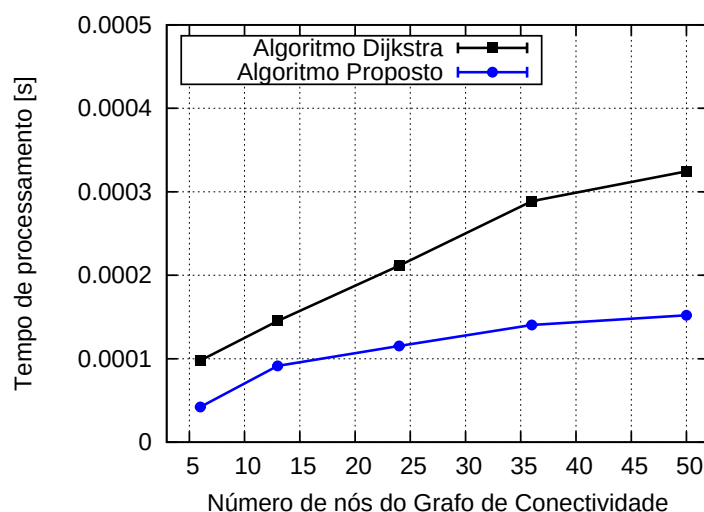
Figura 3.5: Comparativo para o tempo de processamento versus número de nós do grafo de conectividade com inicialização dos cromossomos utilizando critério de sorteio dos vizinhos
