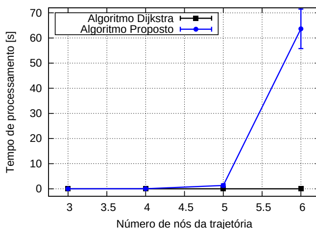
Figura 3.4: Comparativo para o tempo de processamento versus número de nós da trajetória com inicialização dos cromossomos utilizando critério aleatório
