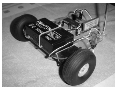
a)Robô móvel
