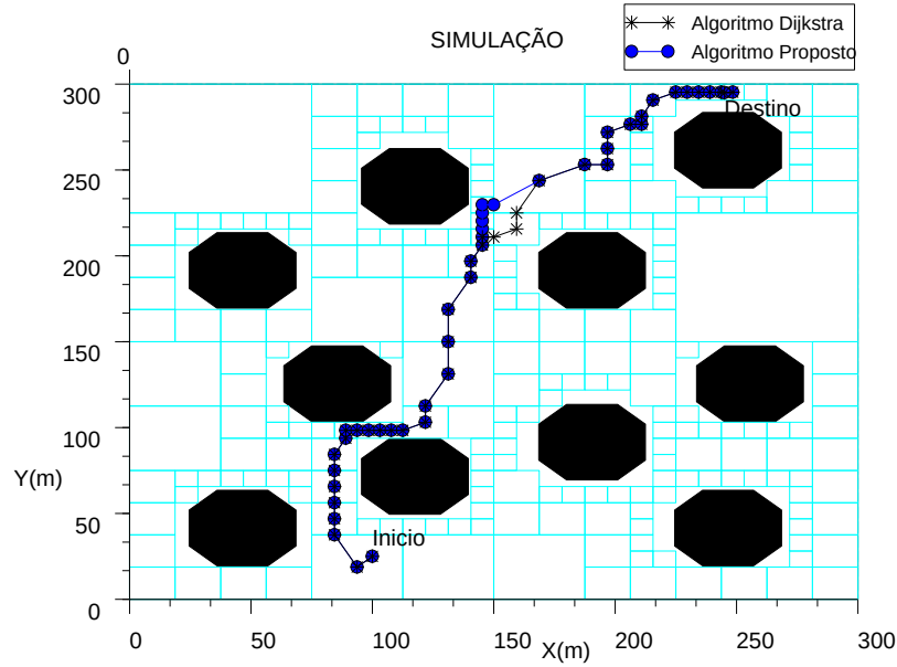
Figura 3.9: Trajetória obtida pelo algoritmo proposto com uma população de 200 indivíduos, 2,40 % maior em relação ao resultado do algoritmo Dijkstra Fonte: (Autor, 2012)
