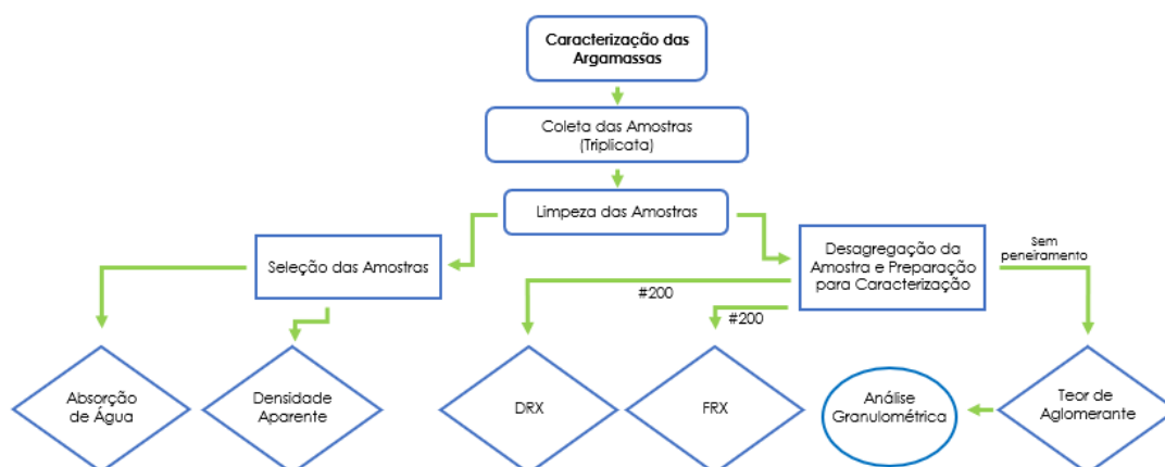
Figura 8. Sequência de processos para caracterização das argamassas. (Fonte: Autoria própria)
