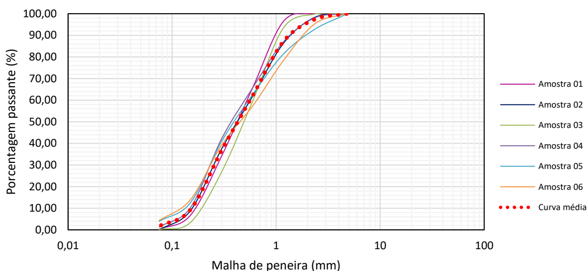
Figura 12. Gráfico das curvas granulométricas das amostras e curva média. (Fonte: Autoria própria)
