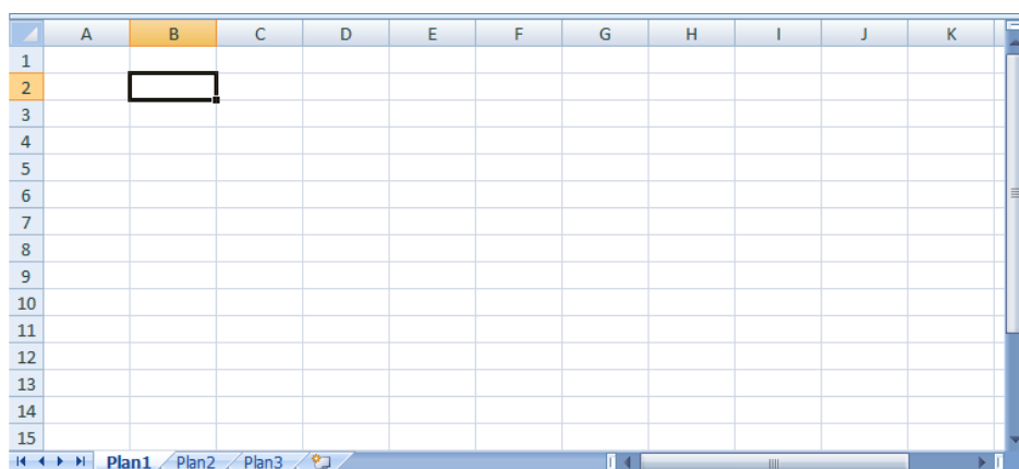
Figura 4 – Planilha Excel
