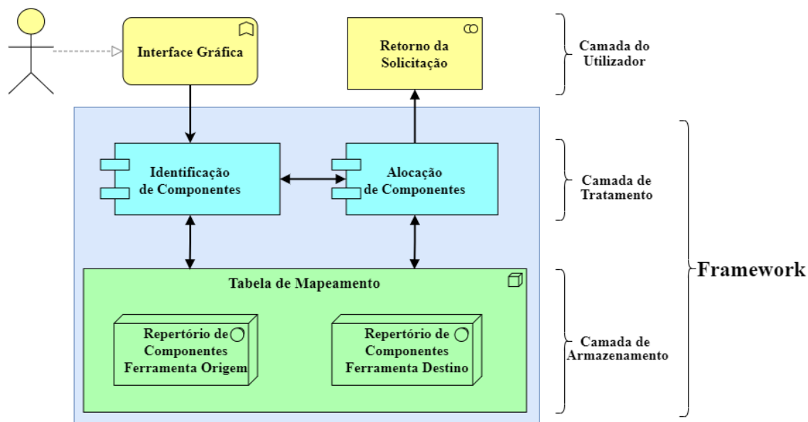
Figura 14 – Arquitetura do framework TADEM.
