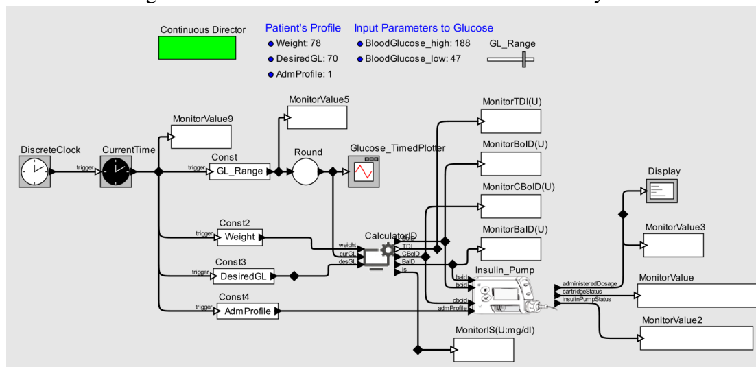
Figura 20 – Modelo da Bomba de Insulina no Ptolemy II®.
