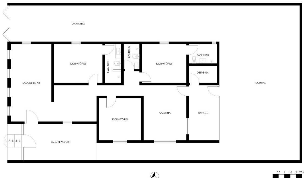
Figura 46 – Planta baixa da Residência 18, Rua Pedro Moura de Vasconcelos
