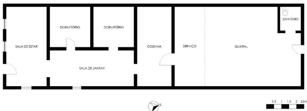
Figura 49 – Planta baixa da Residência 21, Rua Valdomiro Teonácio Bezerra
