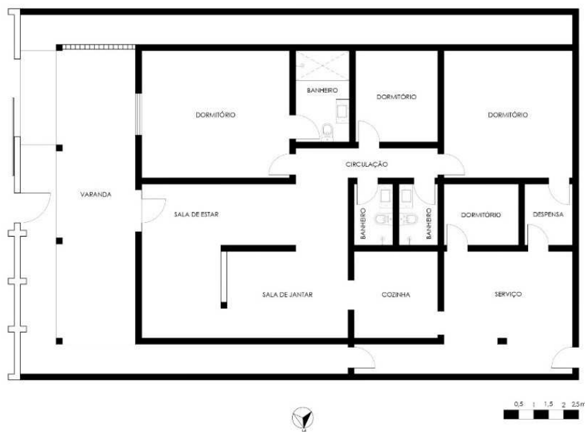
Figura 59 – Planta baixa da Residência 163, Avenida Pedro Matos
