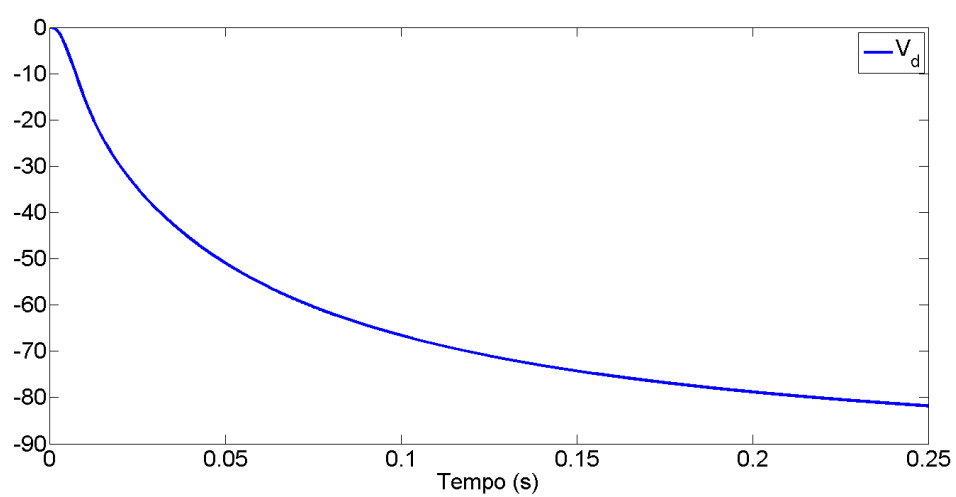
Figura 5.16: Sinal de controle V_d do controlador VS-MRAC.
