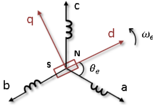
Figura 3.4: Eixos magnéticos do gerador síncrono.
