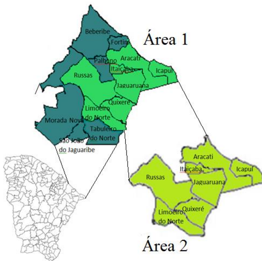
Figura 01- Posição geográfica da área 1 em estudo, compreendendo os municípios de Aracati, Fortim, Icapuí, Itaíçaba, Jaguaruana, Russas, Quixeré, Limoeiro do Norte, Morada Nova e São João do Jaguaribe, Região do Baixo Jaguaribe – CE. Posição geográfica da área 2 municípios de Aracati, Icapuí, Itaíçaba, Jaguaruana, Russas, Quixeré, Limoeiro do Norte, Região do Baixo Jaguaribe, estado do Ceará.
