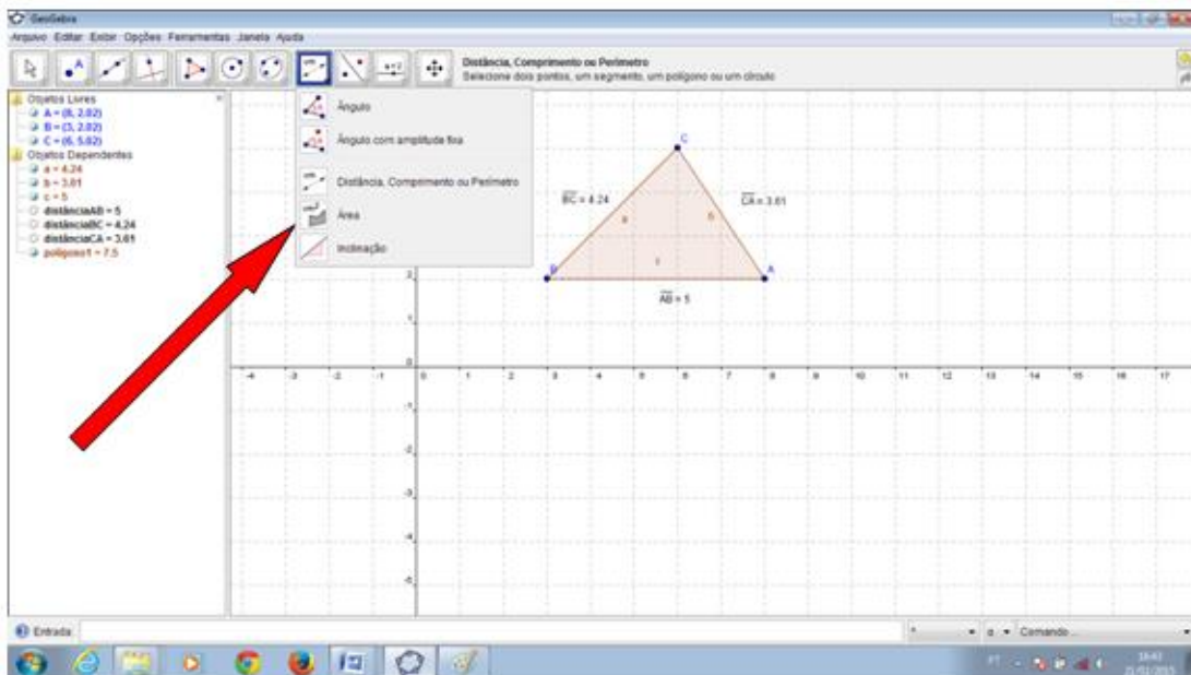
Figura 30 - Calculando a Área do Triângulo
