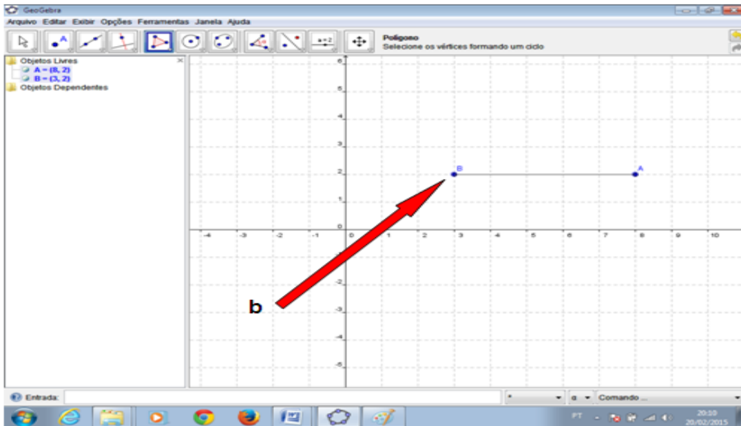
Figura 22 – Formando os lados do Triângulo Escaleno
