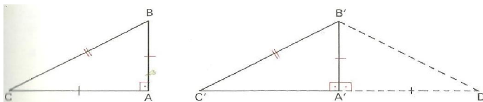
Figura 15 – Congruência no Triângulo Retângulo
