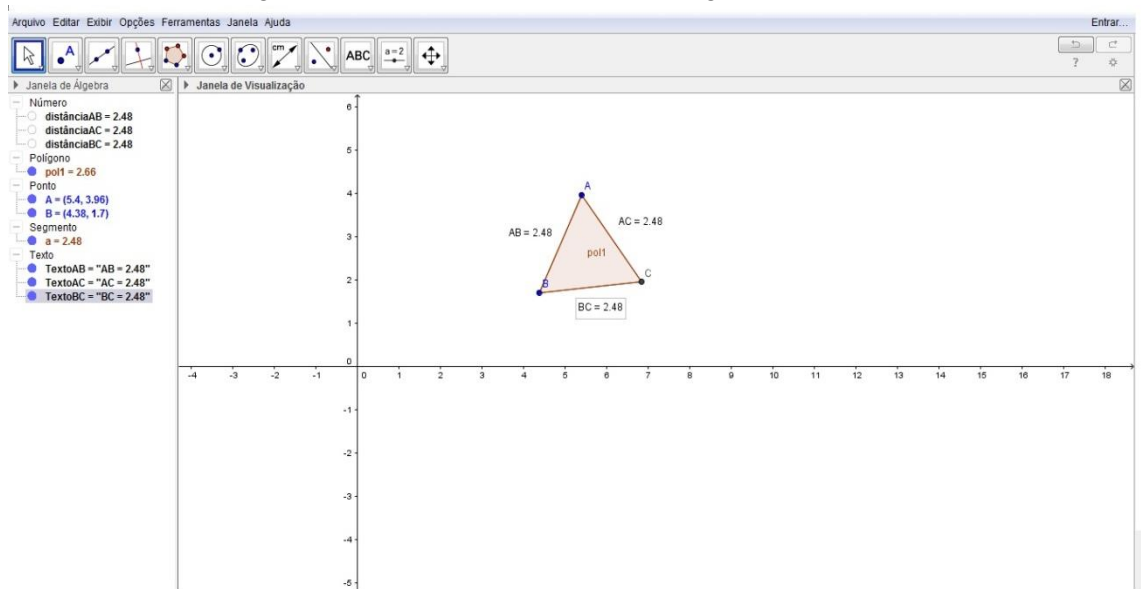
Figura 38 – Medidas dos lados no Triângulo Escaleno
