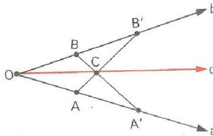
Figura 12 – Bissetriz Interna do Triângulo
