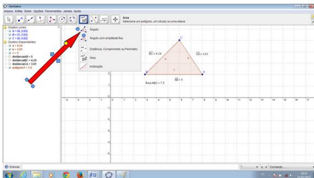
Figura 33 - Comando do GeoGebra: Construindo Ângulos
