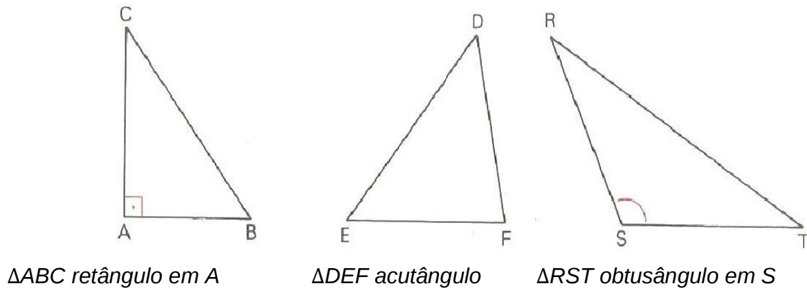
Figura 4 – Classificação dos Triângulos Quanto ao Ângulo
