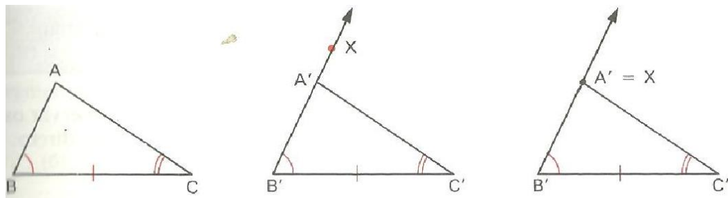
Figura 6 – Congruência de Triângulos Ângulo Lado Ângulo
