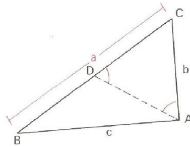
Figura 17 – Ângulo Opondo-se ao Maior lado do Triângulo
