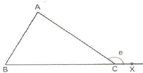
Figura 13 – Teorema Externo do Ângulo
