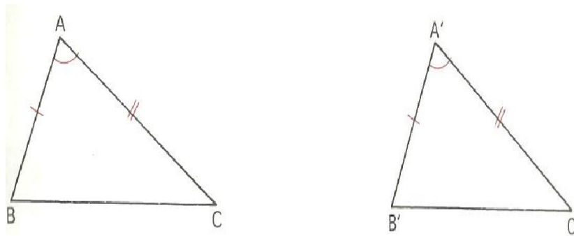
Figura 5 – Congruência de Triângulos Lado Ângulo Lado
