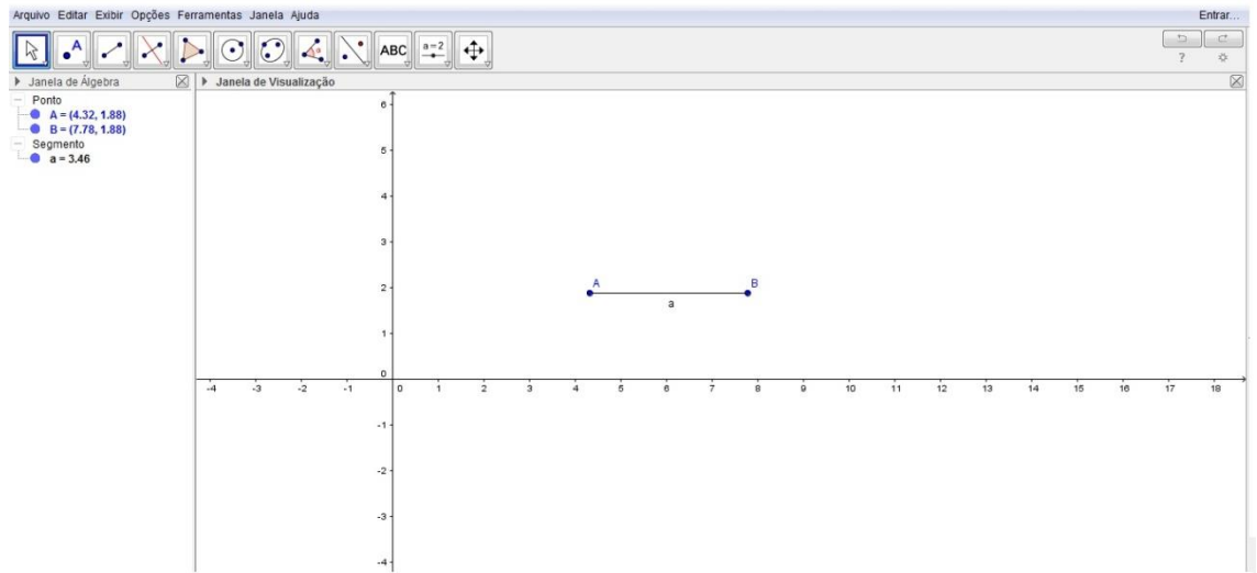
Figura 41- Construindo o Triângulo Isóscele Partindo do Segmento AB
