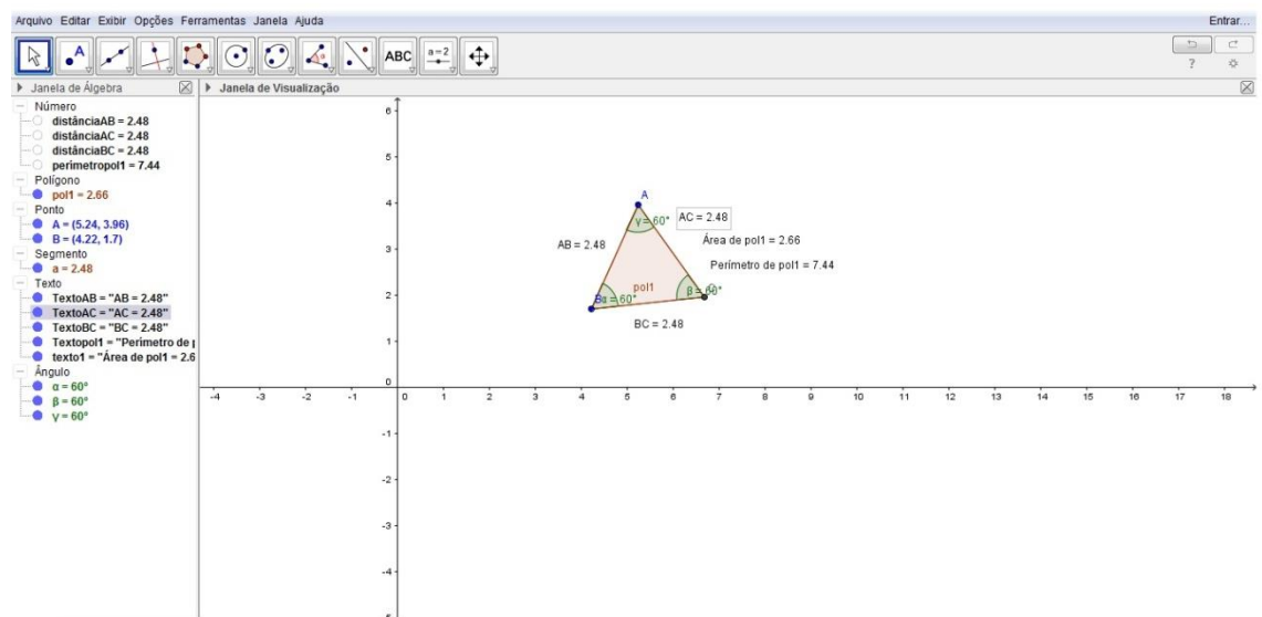
Figura 40 – Ângulos Internos no Triângulo Escaleno
