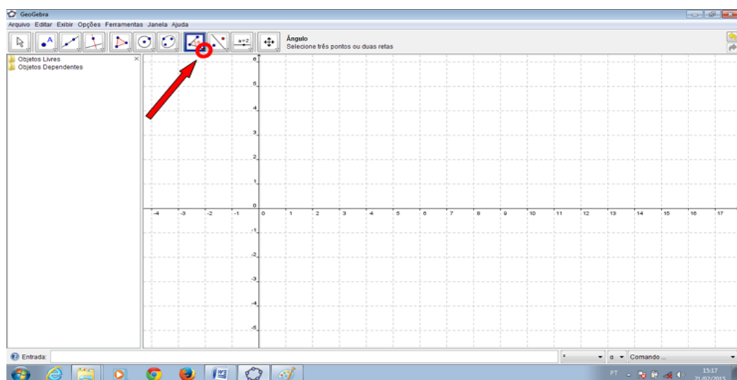
Figura 25 – Comando do GeoGebra
