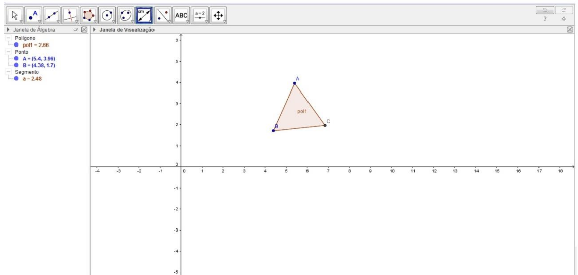
Figura 37 – Pontos Não colineares
