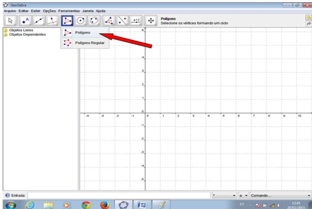
Figura 20 – Janela: Polígonos e Polígonos Regulares
