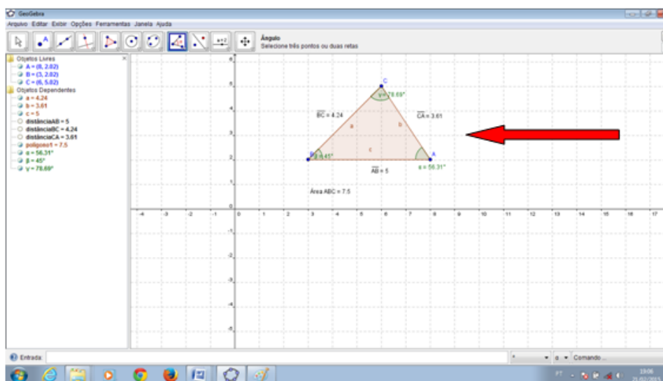
Figura 35 - Construindo Ângulo A\hat{C}B
