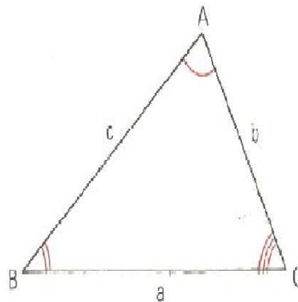
Figura 1 – Elementos do triângulo
