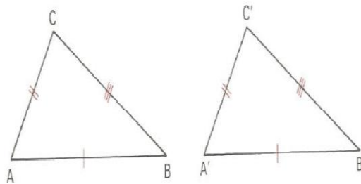
Figura 7 – Congruência de Triângulo Lado Lado Lado
