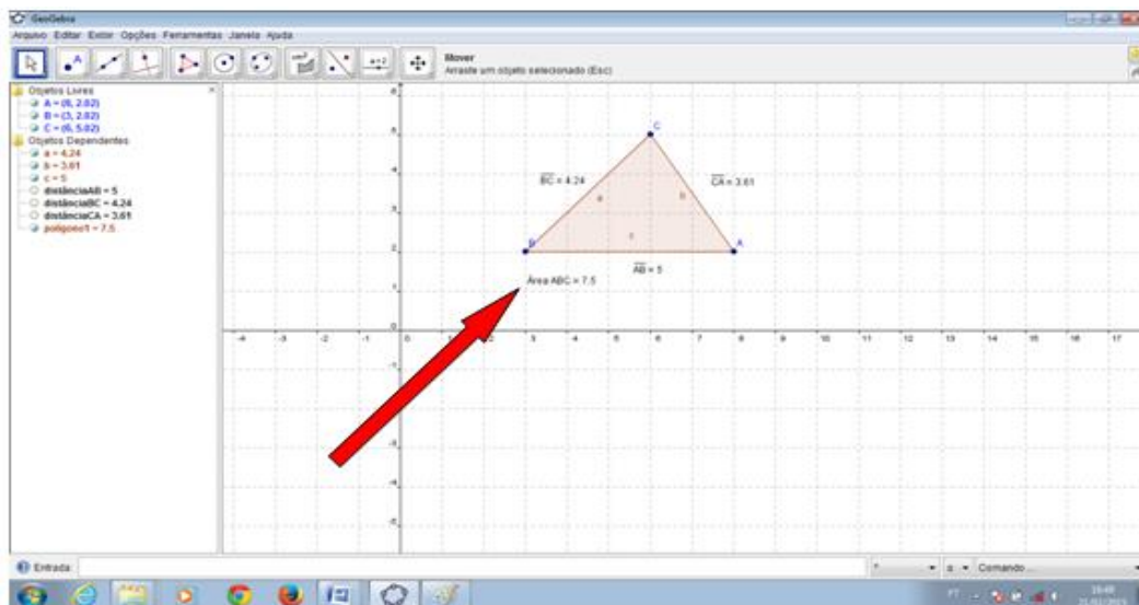
Figura 31 – Resultado da Área do Triângulo
