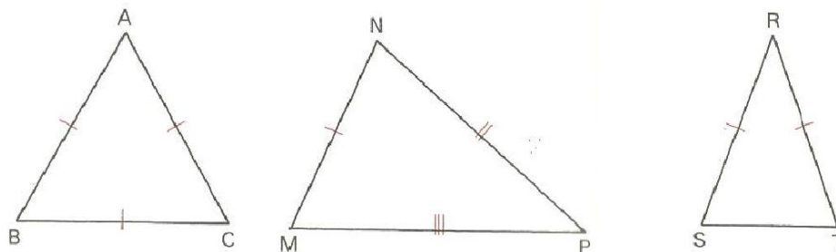
Figura 3 – Classificação dos Triângulos Quanto ao Lado
