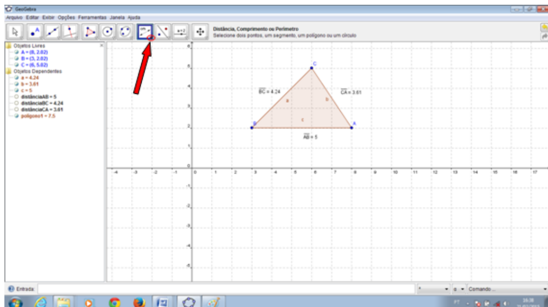
Figura 29 - soma dos lados de um polígono
