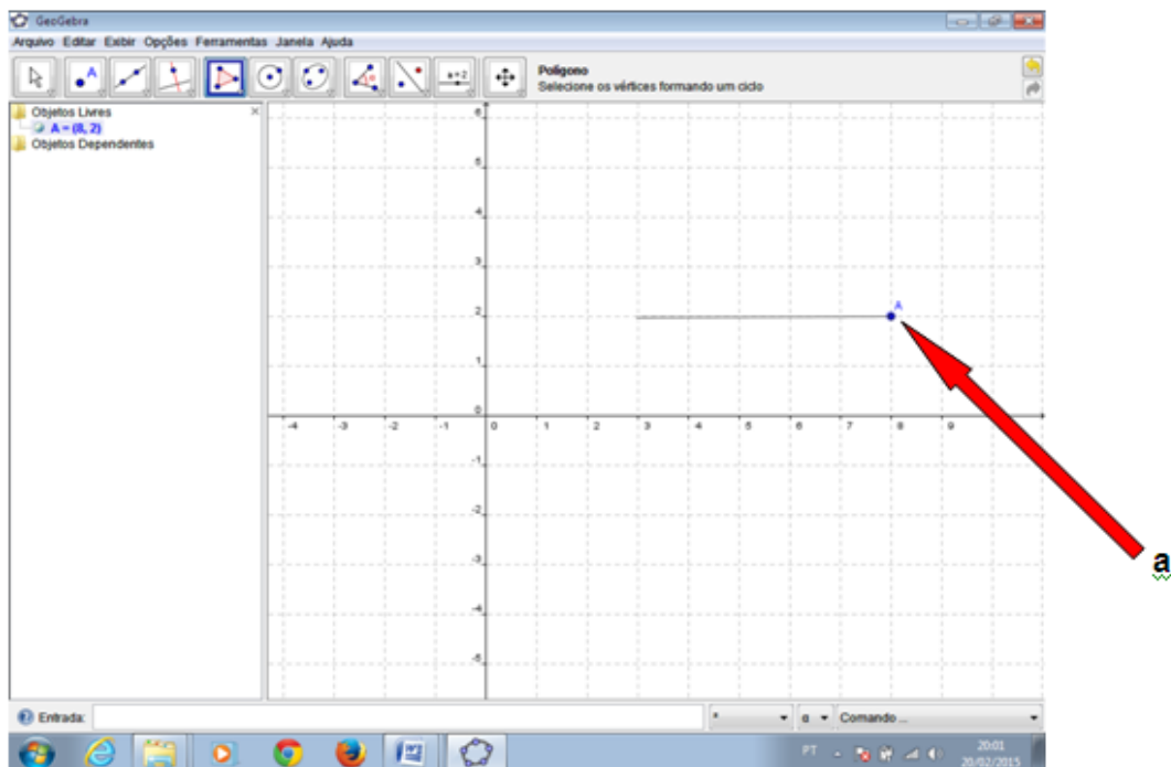
Figura 21 – Pontos Não colineares
