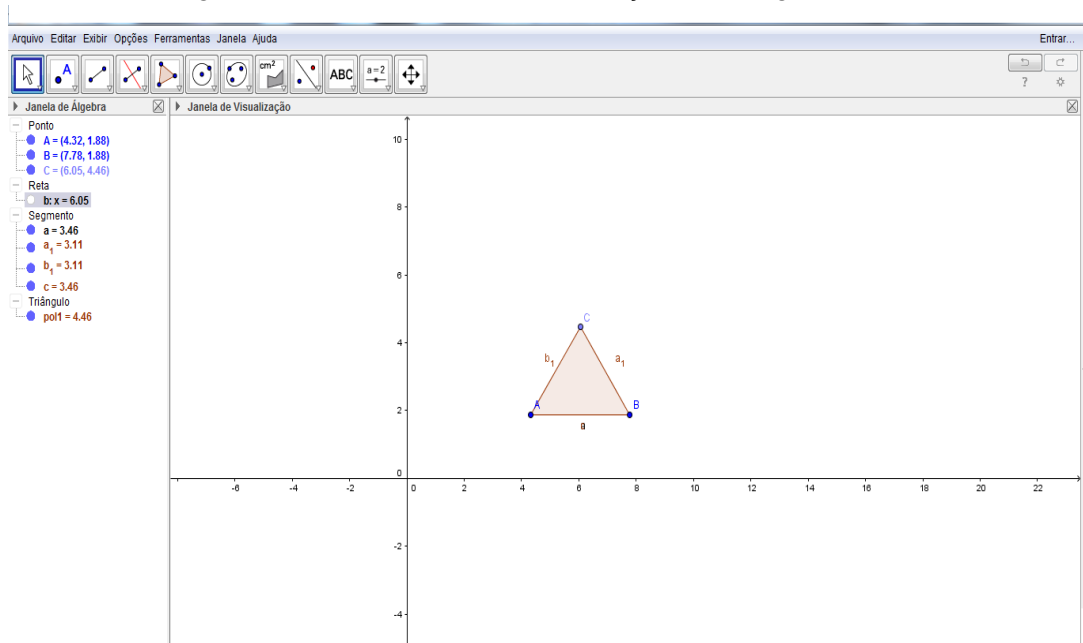
Figura 44 - Passo a Passo na Construção do Triângulo Isóscele
