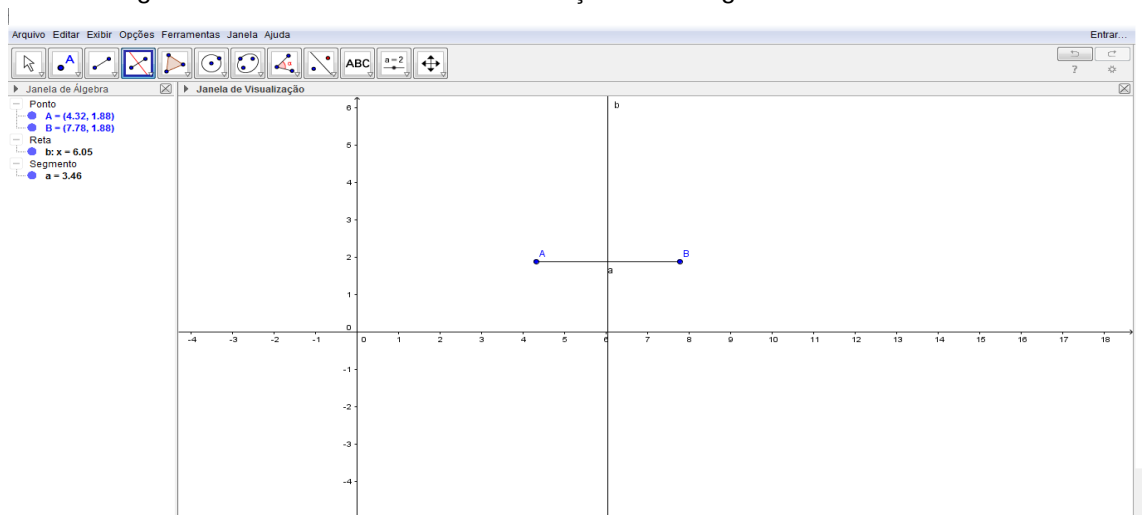
Figura 42 – Passo a Passo na Construção do Triângulo Isóscele
