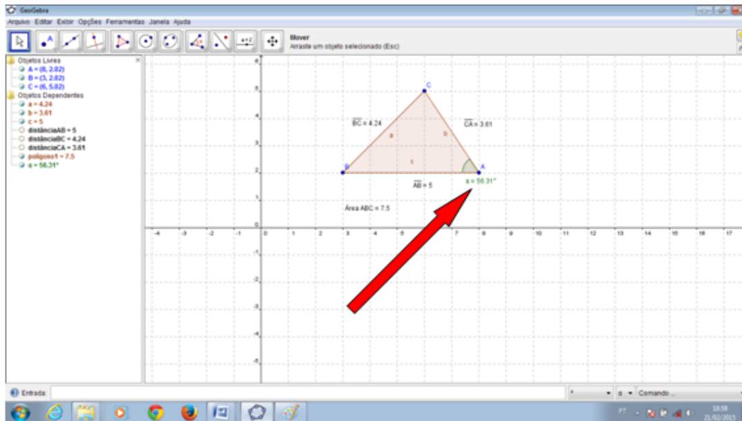
Figura 34 – Medindo o Ângulo B\hat{A}C no GeoGebra
