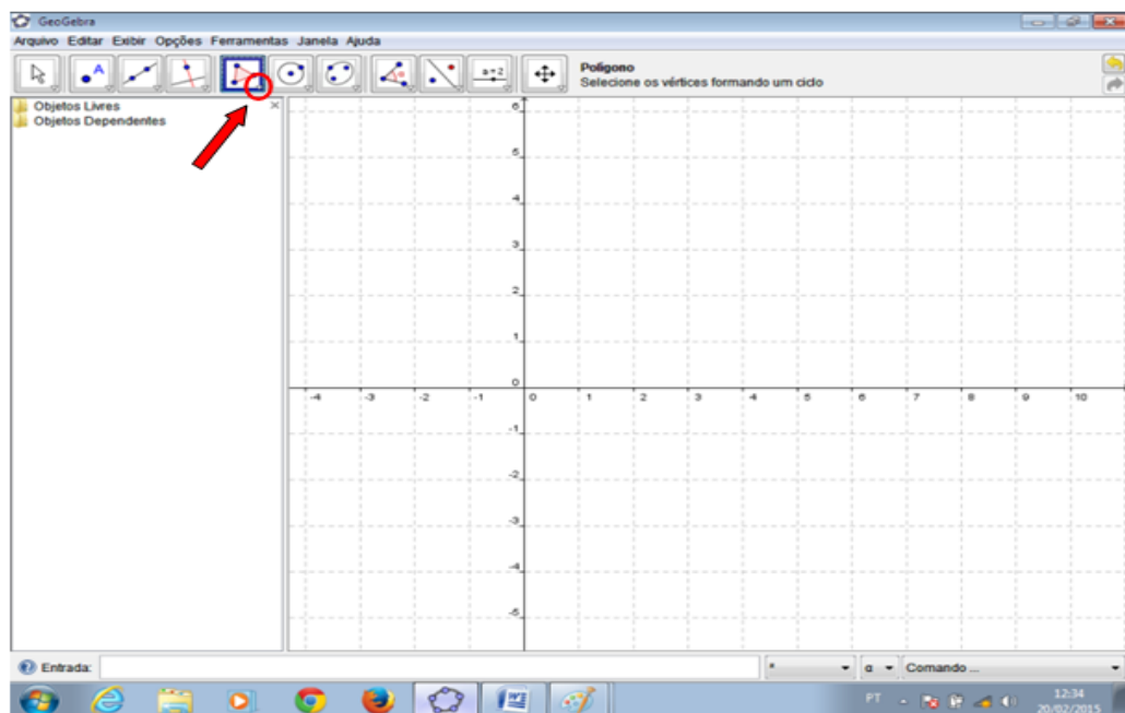
Figura 19 – Construção do Triângulo Escaleno
