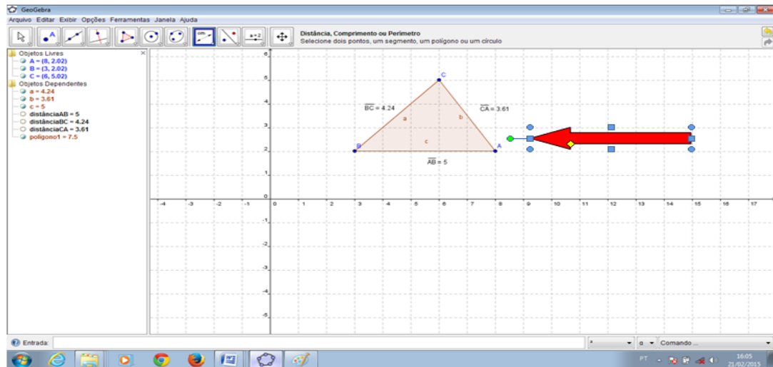
Figura 28 - Construindo os segmentos \overline{BC} e \overline{AC}
