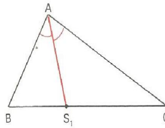
Figura 11 – Mediana do Triângulo
