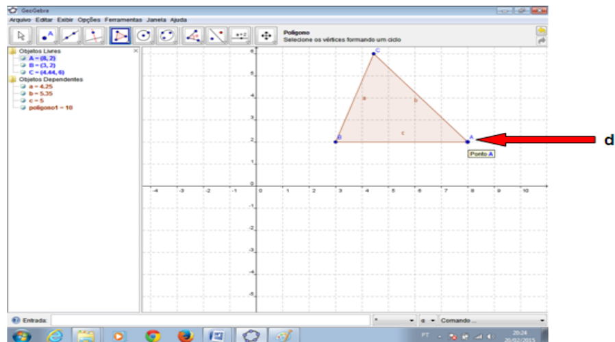
Figura 24 – Finalizado o Triângulo Escaleno
