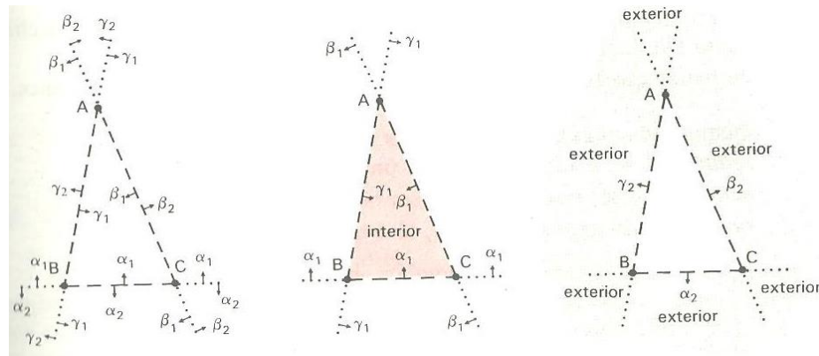
Figura 2 – Elementos Externos e Internos do Triângulo
