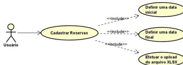
Figura 4: Diagrama de casos de uso da funcionalidade de reserva em lote
