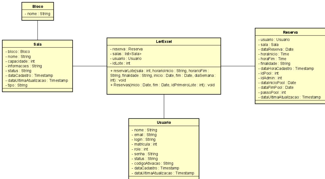
Figura 7: Diagrama de classes da funcionalidade de reserva em lote
