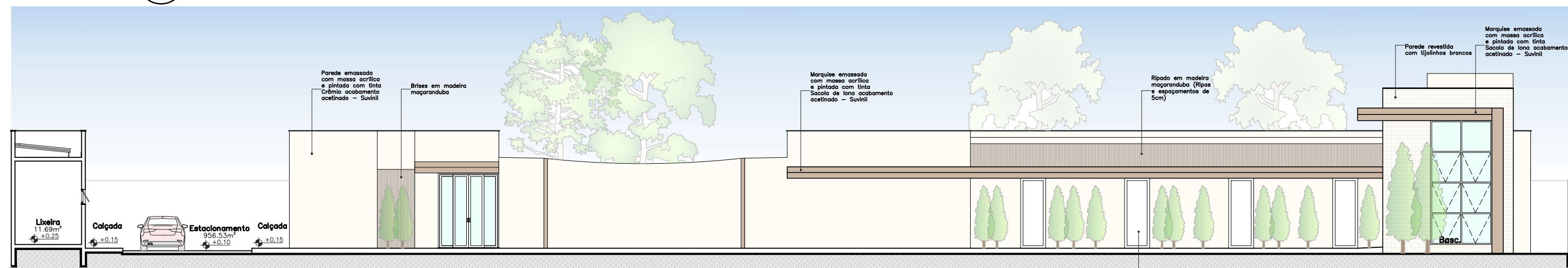
FACHADA 02 ESC. 1:155
