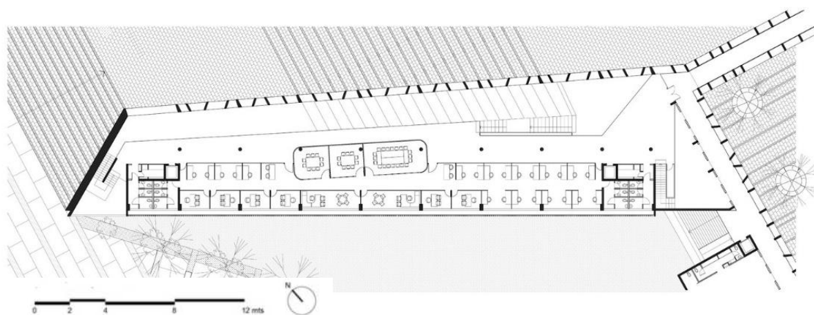
Figura 9: Planta baixa segundo pavimento - Centro Comunitário, Peñalolén, Chile.
