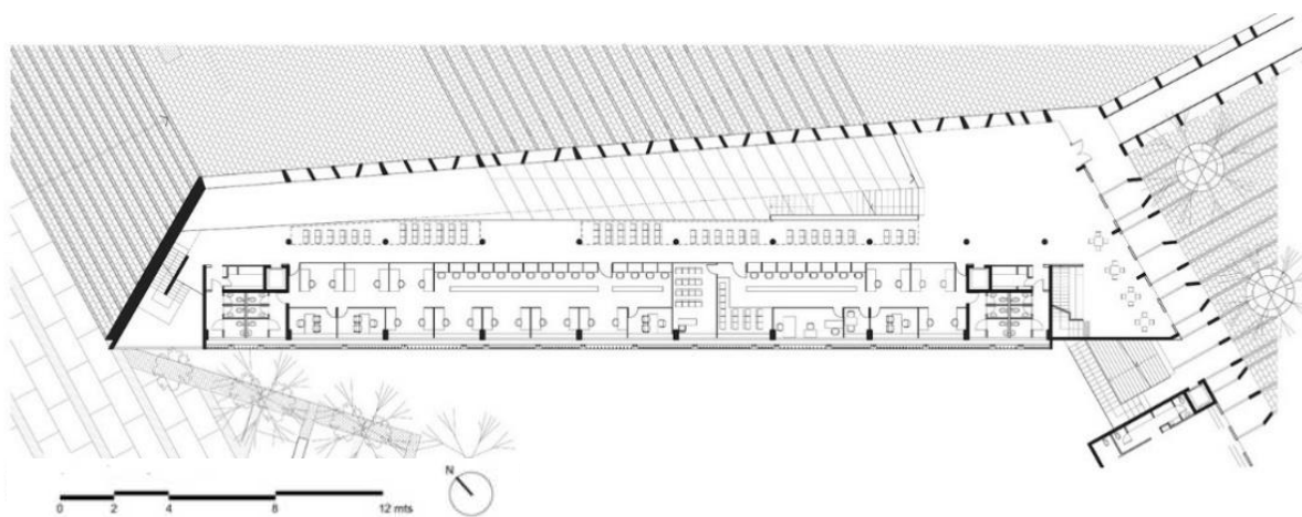
Figura 8: Planta baixa primeiro pavimento - Centro Comunitário, Peñalolén, Chile.
