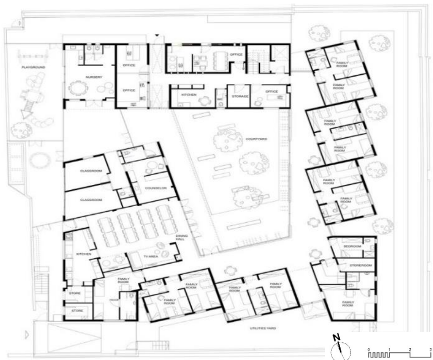
Figura 12: Planta baixa da edificação - The Ada and the Tamar De Shalit House
