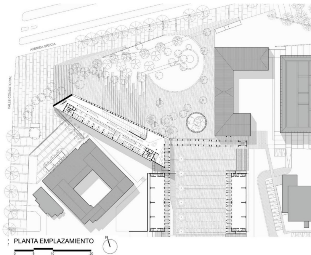
Figura 6: Planta de Implantação - Centro Comunitário, Peñalolén, Chile
