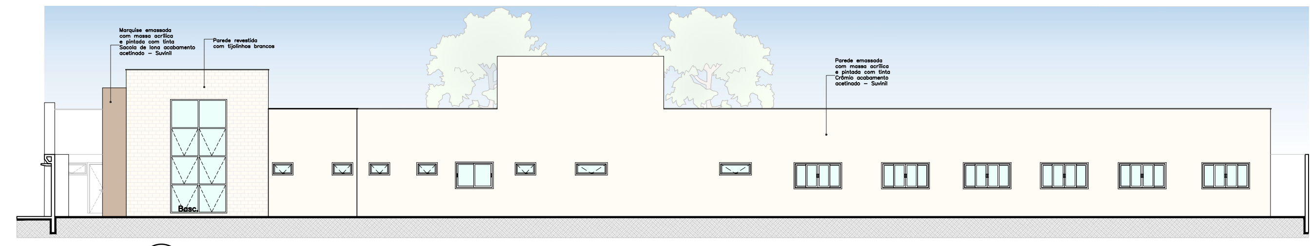
FACHADA 05 ESC. 1:155
