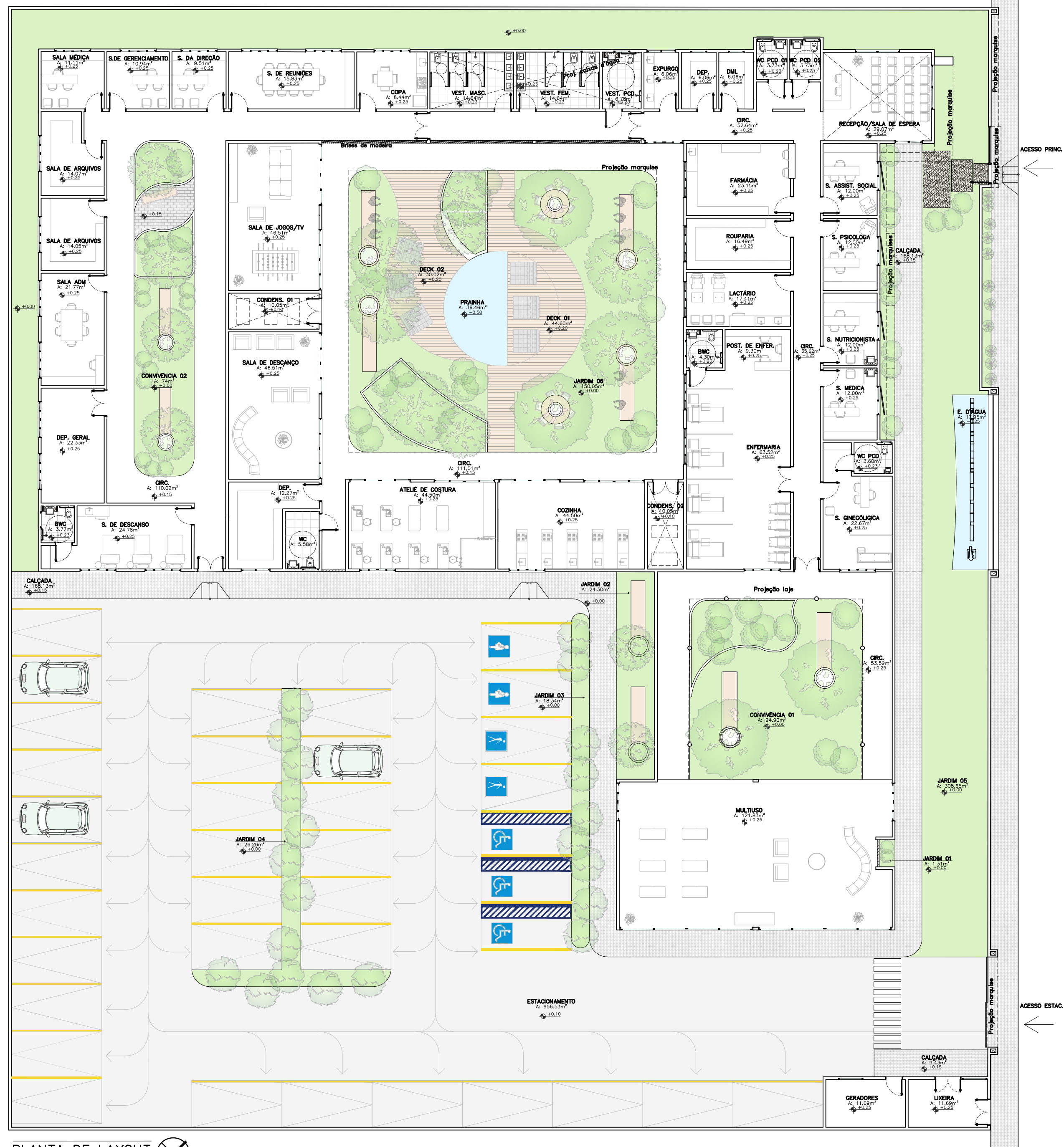
PLANTA DE LAYOUT ESC. 1:175
