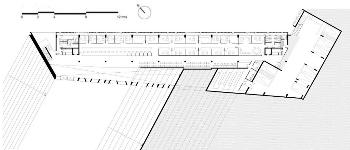
Figura 7: Planta baixa térreo - Centro Comunitário, Peñalolén, Chile
