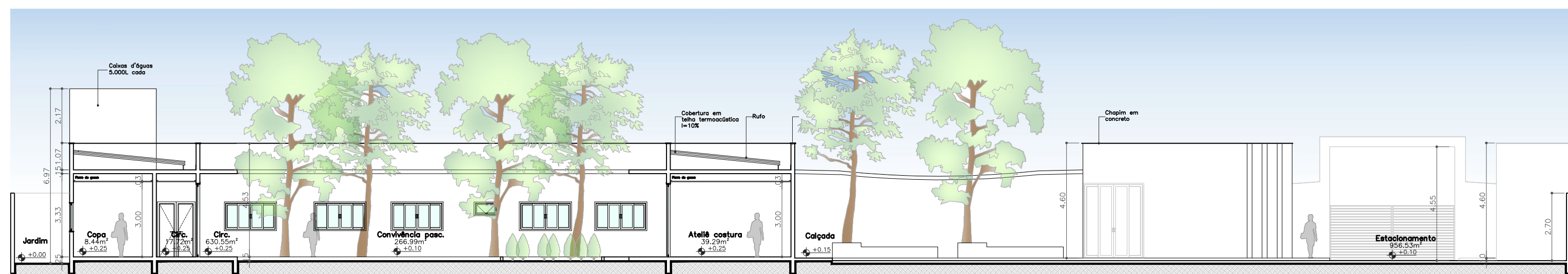
CORTE CC ESC. 1:155
