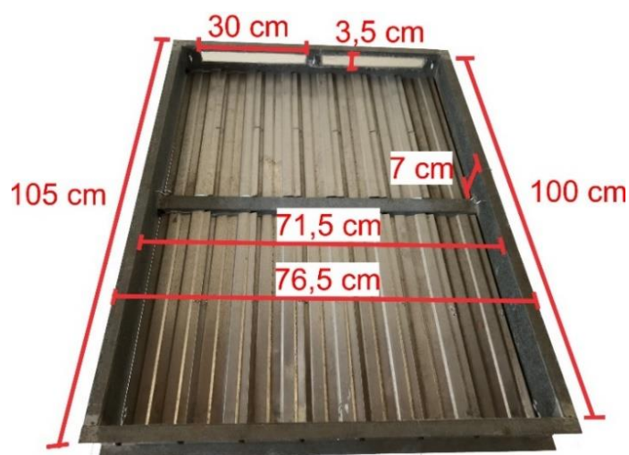
Figura 3. Dimensões da janela utilizada como estrutura para o secador solar reciclável. (Autoria própria)
