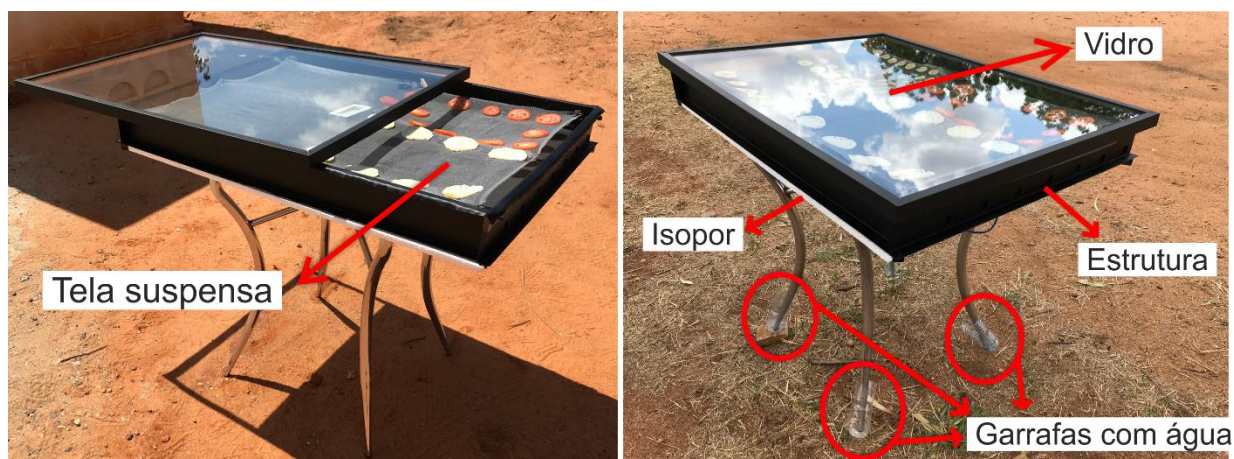
Figura 4. Montagem completa do secador solar proposto. (Autoria própria)
