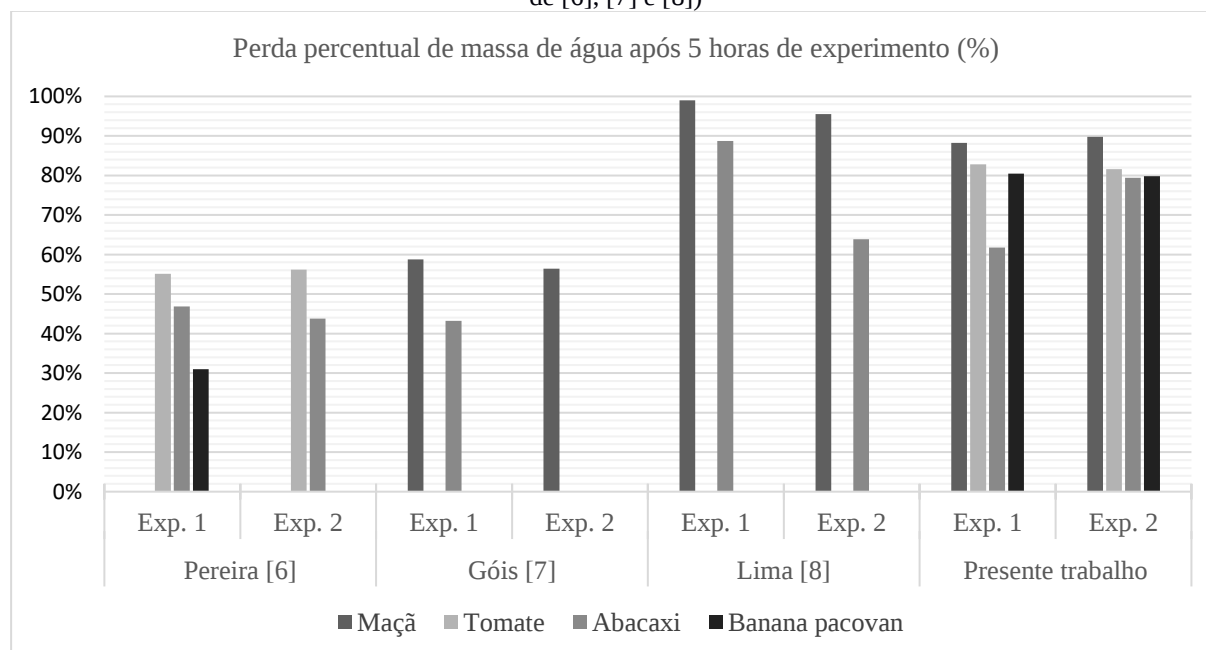
Gráfico 1 – Comparativo de perda de massa de água percentual das frutas após 5 h de experimento. (Adaptado de [6], [7] e [8])
