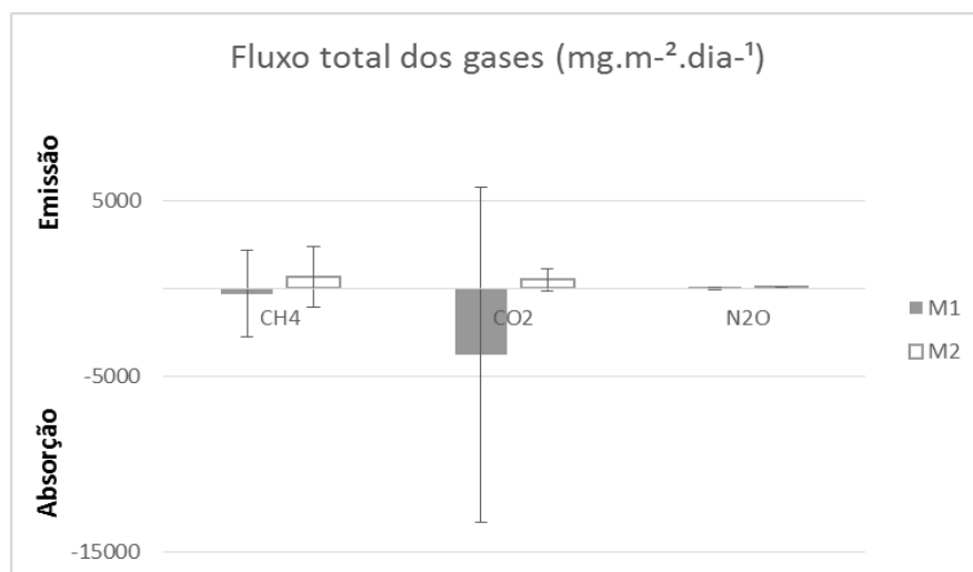
Figura 6: Fluxo total ( \text{mg.m}^{-2}.\text{dia}^{-1} ) nos viveiros de engorda de camarões marinhos para os dois tratamentos para todos os gases analisados. Legenda: M1: Manejo 1, M2: Manejo 2. Fluxo total: fluxo difusivo + fluxo ebulitivo. Absorção (valores negativos) indicam os gases que são absorvidos pelo sistema, Emissão (valores positivos) indicam os gases que são liberados pelo sistema.
