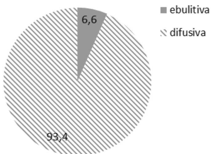
Figura 9: Comparação da contribuição percentual dos gases obtidos pelos dois métodos ebulitivo e difusivo para os dois tratamentos.
