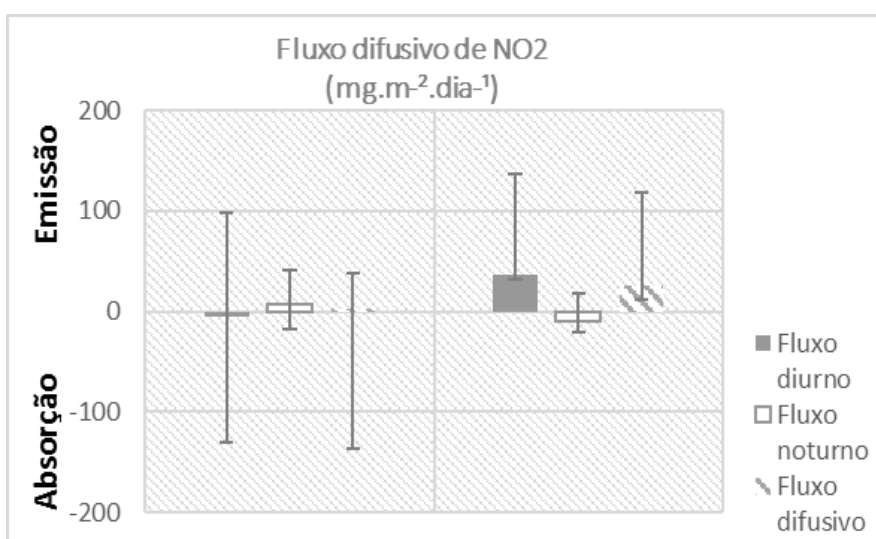
Figura 5: Valores médios e desvios padrão dos fluxos difusivos de N 2 O (mg.m -2 .dia -1 ) para cada tratamento. Legenda: N 2 O: óxido nitroso, M1: Manejo 1, M2: Manejo 2, Absorção (valores negativos): gases que são absorvidos pelo sistema. Emissão (valores positivos): gases que são liberados pelo sistema.
