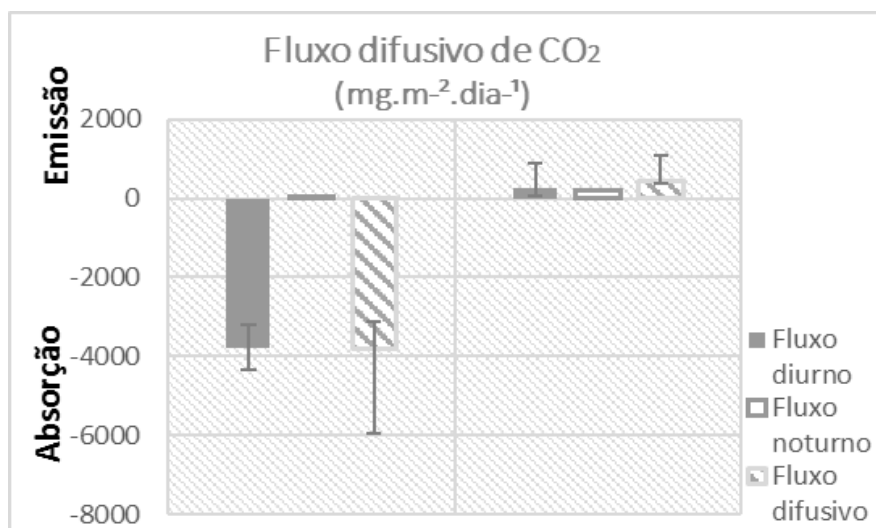
Figura 4: Valores médios e desvios padrão dos fluxos difusivos de CO 2 (mg.m -2 .dia -1 ) para cada tratamento. Legenda: CO 2 : dióxido de carbono, M1: Manejo 1, M2: Manejo 2, Absorção (valores negativos): gases que são absorvidos pelo sistema. Emissão (valores positivos): gases que são liberados pelo sistema.
