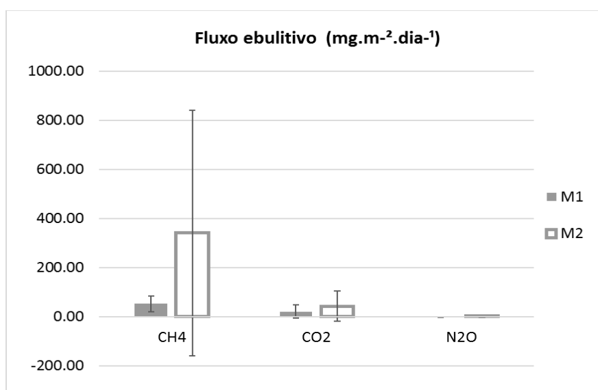
Figura 2: Valores médios e desvios padrão dos fluxos ebulitivos ( \text{mg.m}^{-2}.\text{dia}^{-1} ) para cada tratamento. Legenda: \text{CH}_4 – Metano, \text{CO}_2 – dióxido de carbono, \text{N}_2\text{O} – Óxido nitroso, M1: Manejo 1, M2: Manejo 2.
