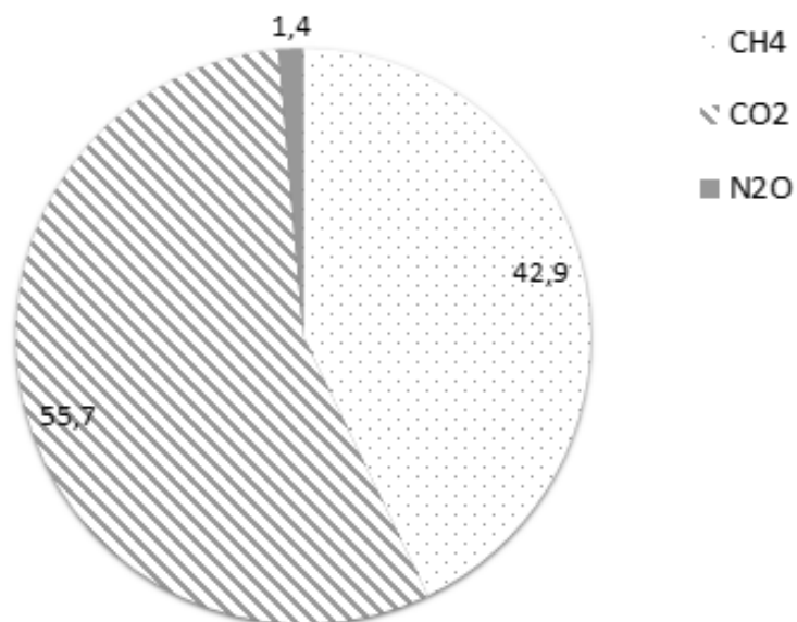
Figura 8: Distribuição quantitativa dos gases produzidos durante o período de estudo. Legenda: CH 4 –Metano, CO 2 – dióxido de carbono, N 2 O – Óxido nitroso. Fluxo total: emissão difusiva + emissão ebulitiva.
