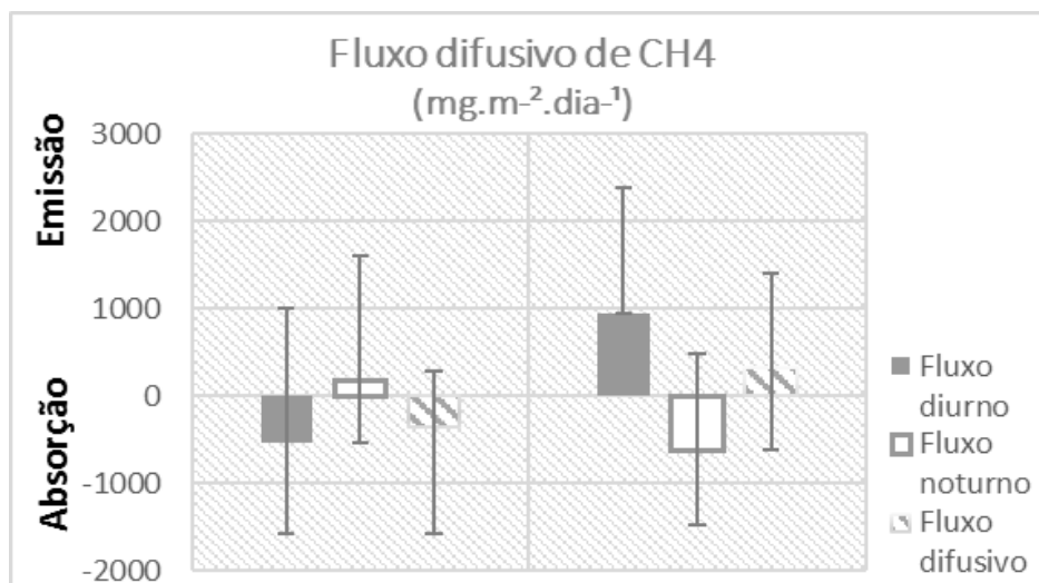
Figura 3: Valores médios e desvios padrão dos fluxos difusivos de \text{CH}_4 ( \text{mg.m}^{-2}.\text{dia}^{-1} ) para cada tratamento. Legenda: \text{CH}_4 , metano, M1: Manejo 1, M2: Manejo 2, Absorção (valores negativos): gases que são absorvidos pelo sistema. Emissão (valores positivos): gases que são liberados pelo sistema.
