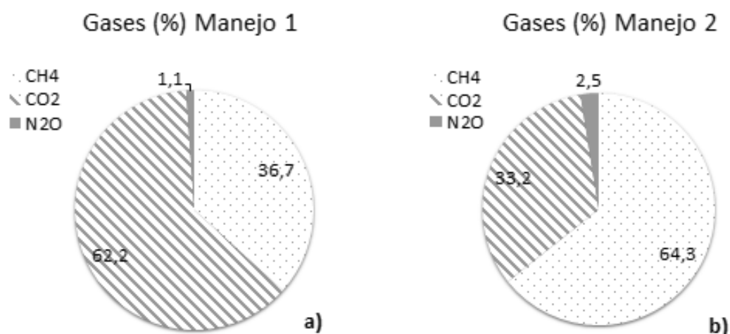
Figura 10: Comparação da contribuição percentual dos gases obtidos para os diferentes manejos realizados. a) Manejo 1, b) Manejo 2. Legenda: CH 4 : Metano, CO 2 : dióxido de carbono, N 2 O: Óxido nitroso.
