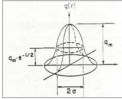
Figura 3. Fonte de calor Gaussiana. [12]
