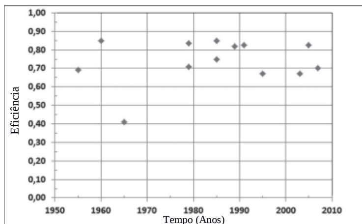
Figura 1. Valores médios de eficiência do processo TIG com o tempo. [9]
