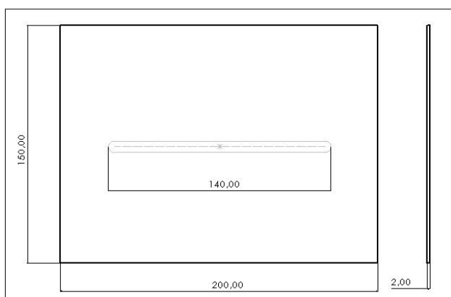
Figura 6. Ilustração do corpo de prova. (Autoria própria)
