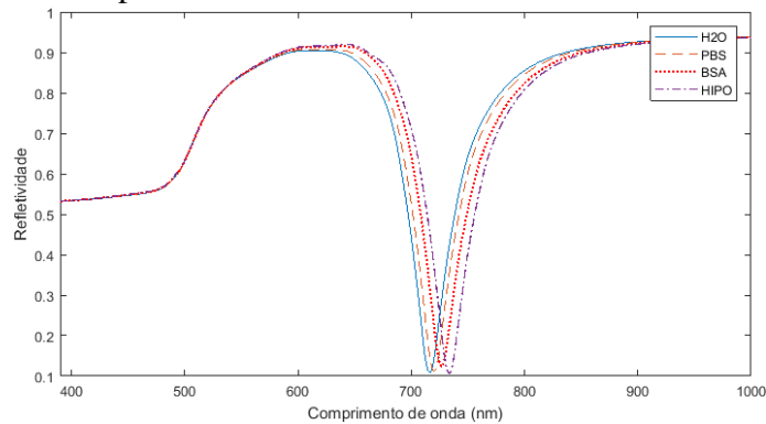
Figura 13 – Cuvas SPR teóricas WIM do sensor com prisma de BK7/Au (50 nm) para H_2O , PBS, BSA e Hipo.
