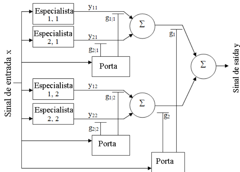
Figura 11 – Diagrama de blocos de uma máquina de comitê dinâmico com mistura hierárquica de especialistas. As saídas dos especialistas (1,1) e (2,1) são combinadas por g_{1|1} e g_{2|1} , produzindo uma saída g_1 que é combinada com a saída g_2 , produzindo uma saída y geral
