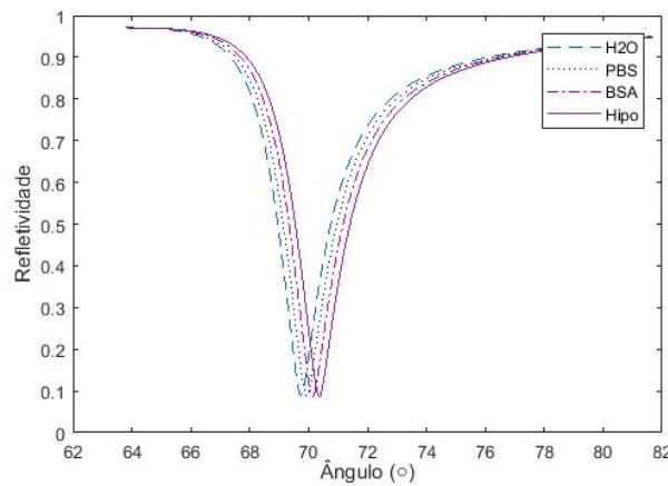
Figura 14 – Cuvas SPR teóricas AIM do sensor com prisma de BK7/Au (50 nm) para H_2O , PBS, BSA e Hipo.
