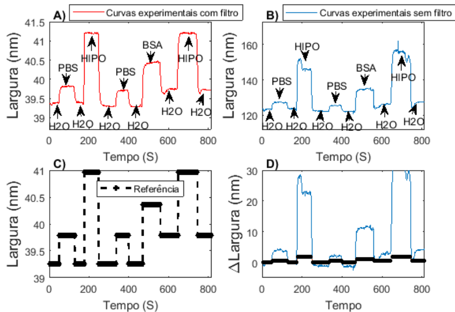
Figura 35 – Sensorgramas de largura, para o sistema multicamada composto por Ouro e BK7 em modo WIM.
