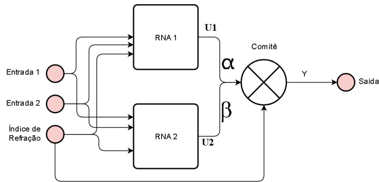
Figura 28 – Comitê dinâmico com dois especialistas, a saída do especialista RNA 1 é dada por U1 e a saída do especialista RNA 2 é dada por U2, de acordo com o índice de refração de cada substância o comitê julga a ponderação de cada especialista
