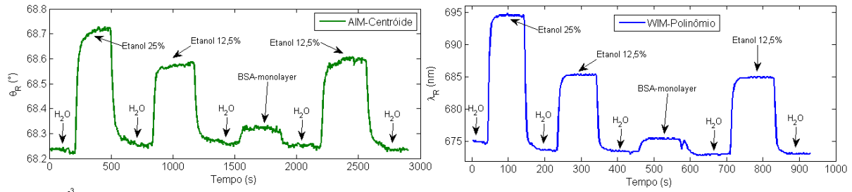
Figura 5 – Sensorgrama para o ciclo experimental H_2O \rightarrow \text{Etanol } 25\% \rightarrow H_2O \rightarrow \text{Etanol } 12,5\% \rightarrow H_2O \rightarrow \text{BSA} \rightarrow H_2O \rightarrow \text{Etanol } 12,5\% .
