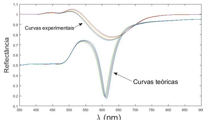
Figura 26 – Curvas experimentais e teóricas para para sistema multicamada composto por Ouro e Pc.
