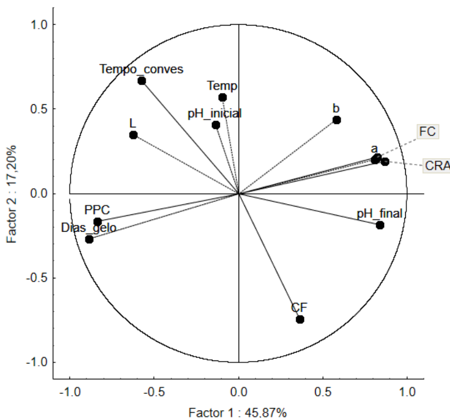
Gráfico 2- Gráfico bidimensional dos CP1 e CP2. Fonte: Arquivo pessoal.
