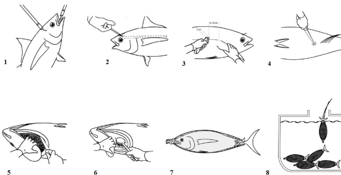
Figura 0-1 - Fluxograma pós-captura de manipulação do atum. (Adaptado de Blanc et al., 2005).
