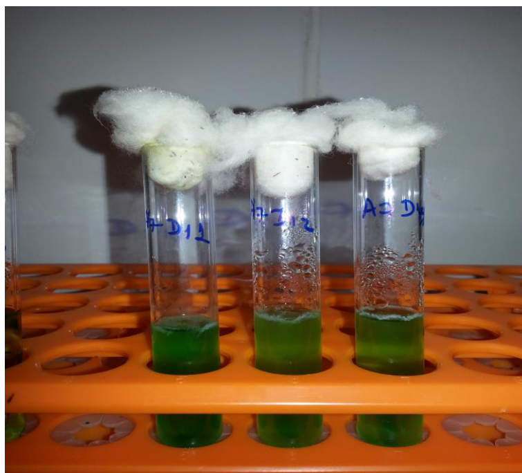
Figura 16 – Coliformes totais
