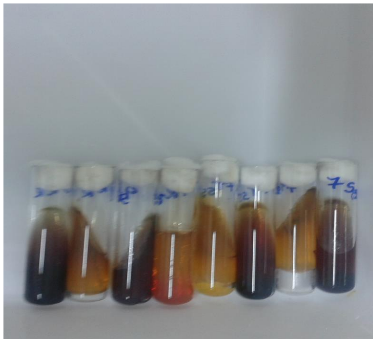
Figura 19 – Salmonella spp.
