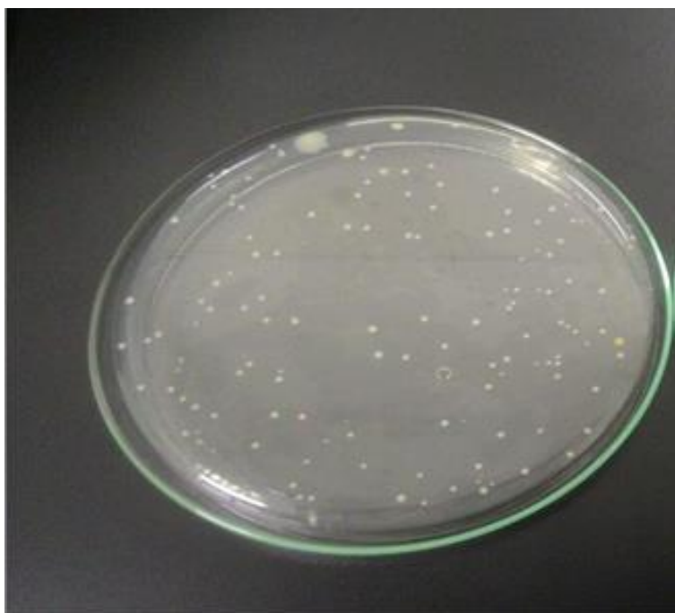
Figura 15 – Aeróbios mesófilos
