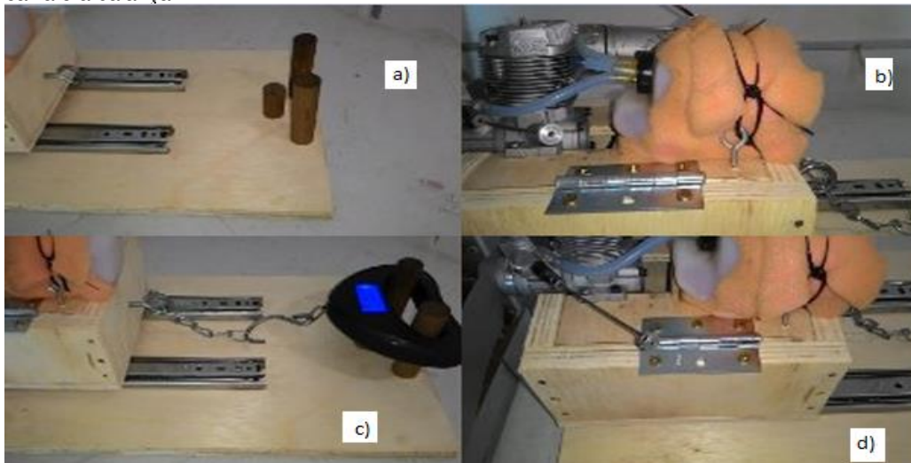
Figura 7: a) Toquinhos de madeira, b) Ganchos roscados de fixação do tanque, c) Gancho roscado para unir a caixa e a balança.
