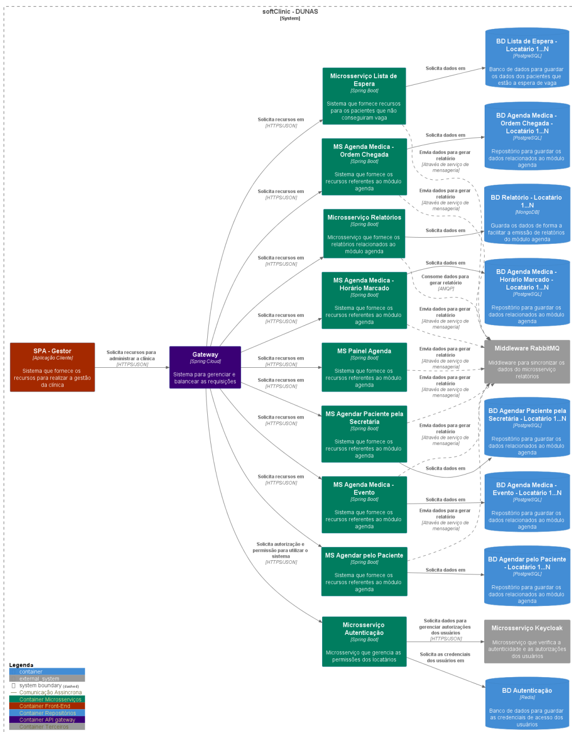
Figura 27 – Arquitetura de microserviços do subdomínio Agenda da LPS.
