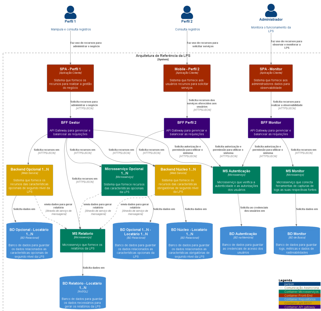
Figura 17 – Arquitetura de referência da LPS
