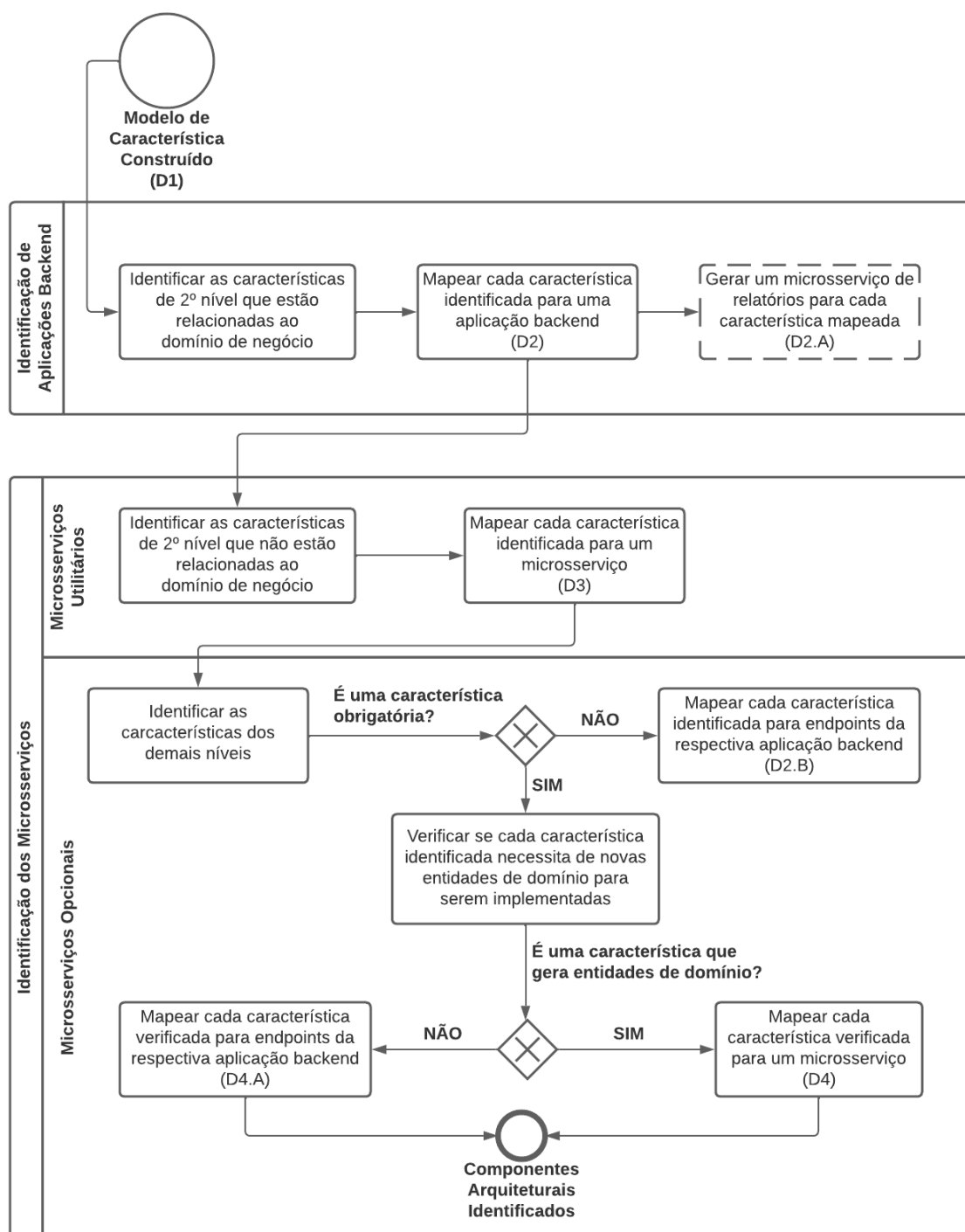
Figura 16 – Representação das diretrizes em fluxograma
