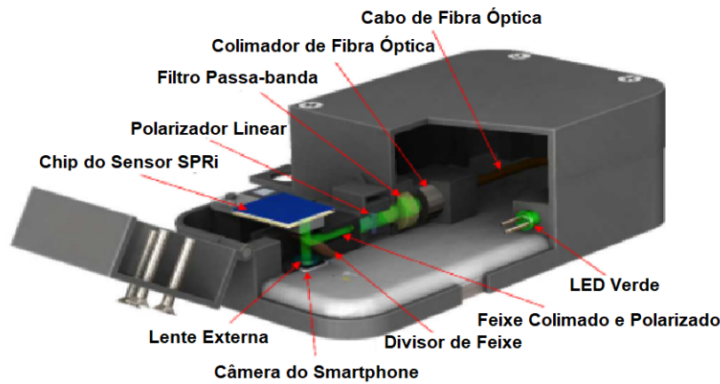
(a) Visão completa da arquitetura do projeto do sensor SPRI
