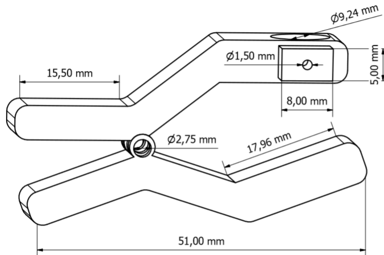
Figura 27 – Clip adaptador do MobileSPR App.
