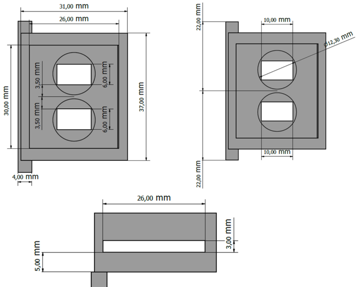
Figura 34 – MobileSPR Case 2.0 - Plataforma de Suporte.
