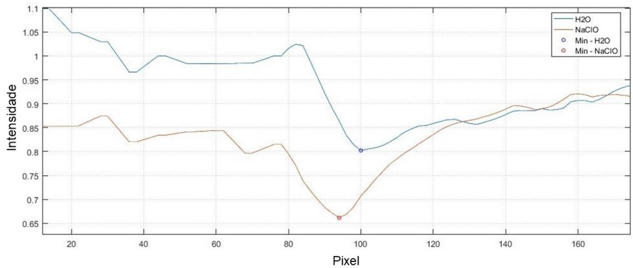
Figura 39 – Sinais de saída do experimento após o gotejamento das substâncias ( Wet Cell ) capturados pelo aplicativo.
