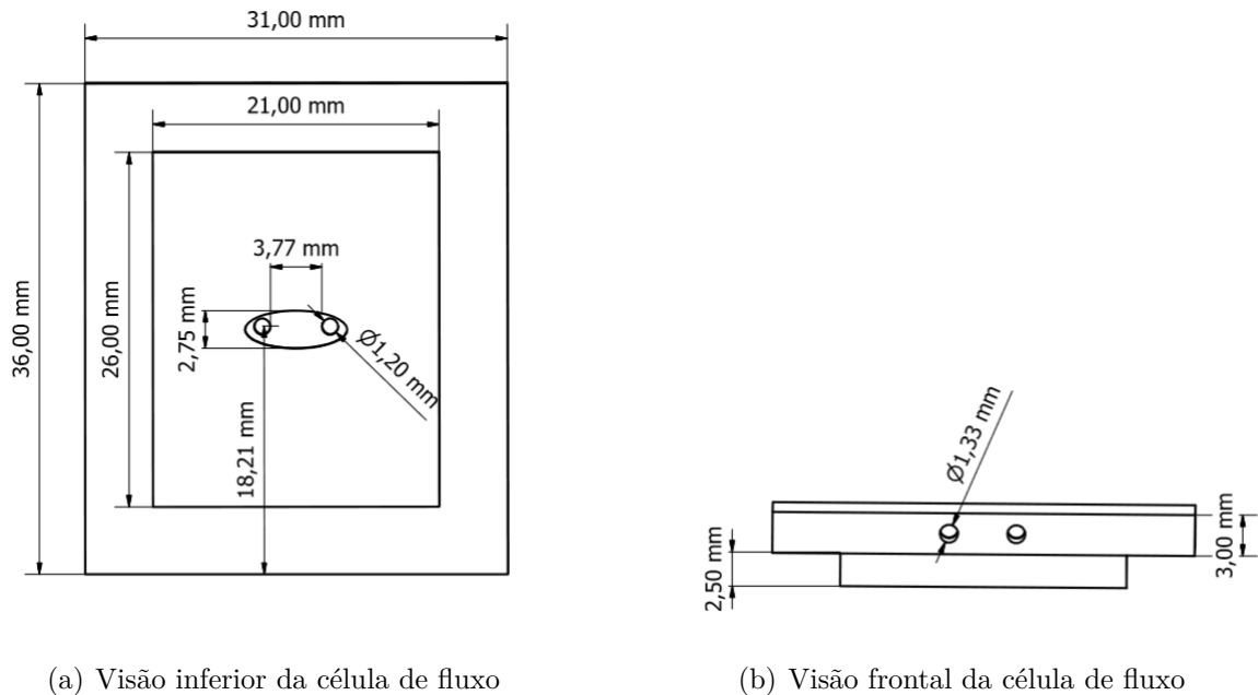
Figura 25 – Célula de Fluxo do MobileSpr Case.
