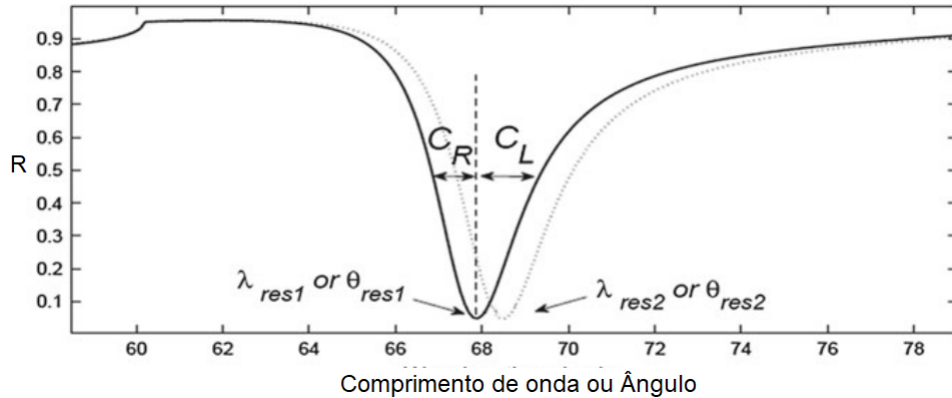
Figura 9 – Gráfico com a curva SPR formada e a obtenção dos valores de refletividade do meio.
