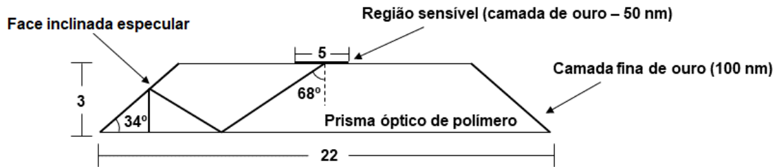
Figura 13 – Design do prisma polimérico PPBIO.
