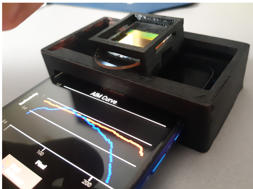
Figura 35 – MobileSPR Case - Montagem com o Virchip.
