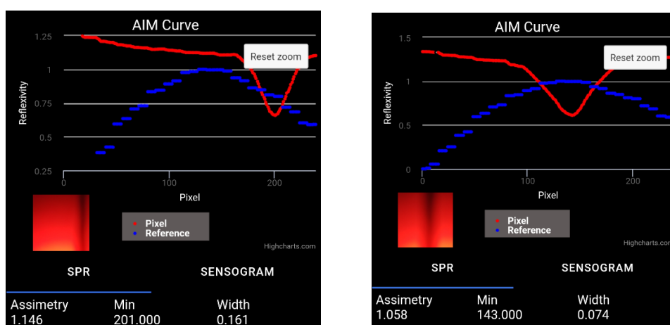
(a) Visualização da curva SPR simulando a inserção de H 2 O na superfície do biochip
