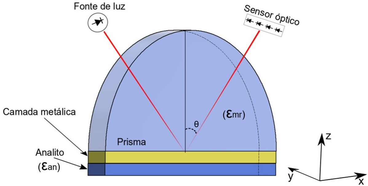
Figura 8 – Estrutura do sensor óptico multicamada SPR baseado em prisma proposto por Kretschmann e Raether (1968).
