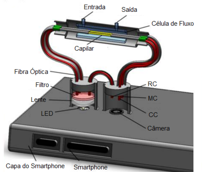
Figura 3 – Esquema do sensor SPR com estrutura de fibra óptica baseado em smartphone .
