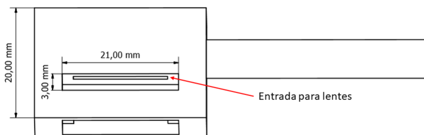
(b) Visão frontal do suporte
