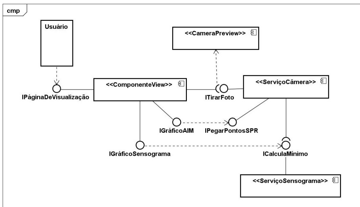
Figura 20 – MobileSPR App - Diagrama de Componentes.
