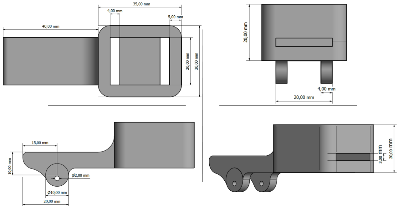
Figura 30 – MobileSPR Case 1.1 - visão geral superior.
