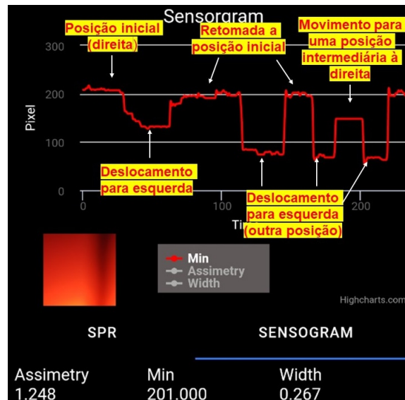
Figura 37 – MobileSPR App - Representação dos valores mínimos das curvas SPR simuladas no aplicativo.
