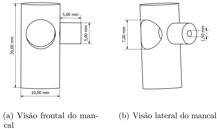
Figura 26 – Mancal do MobileSpr Case.
