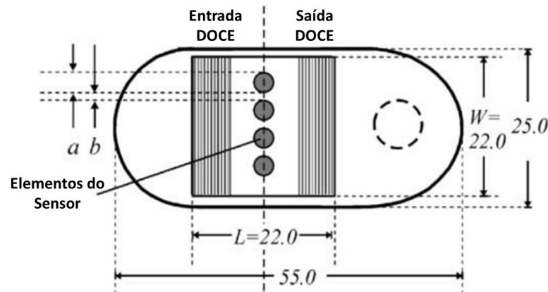
Figura 14 – Dseign do Virchip.
