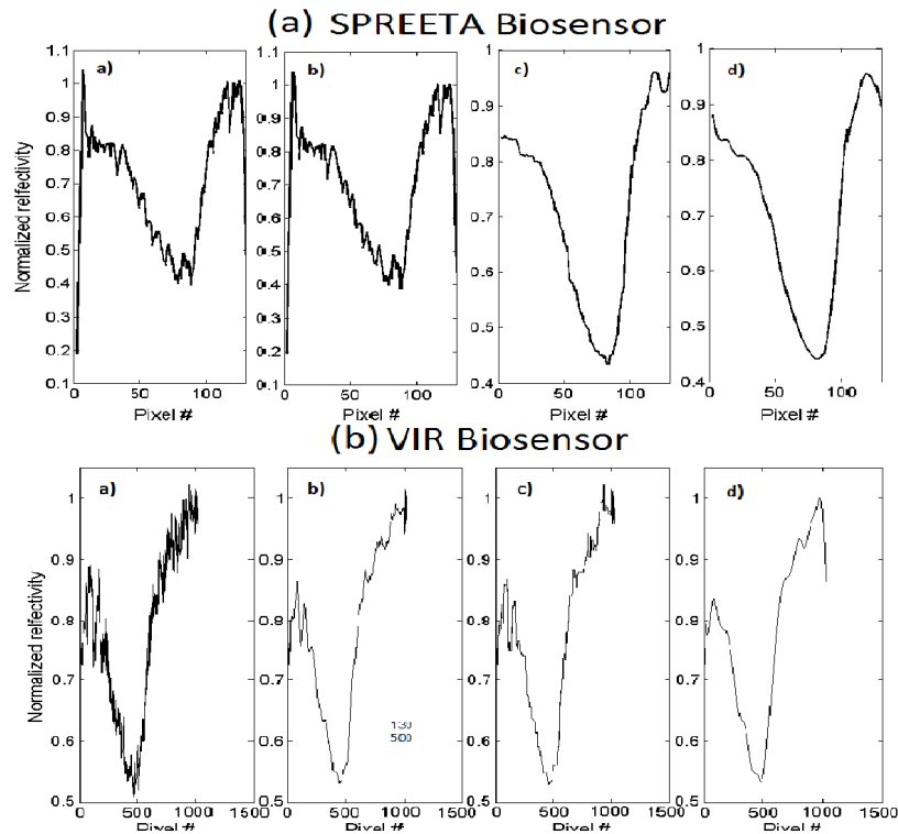
Figura 11 – Comparativo do sinal com diferentes aplicações de filtros. a) dados sem filtros, b) média temporal, c) mediana espacial e d) filtro passa-baixa
