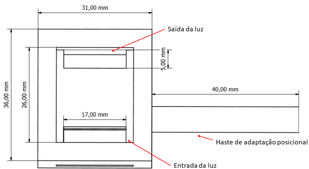
(a) Visão superior do suporte
