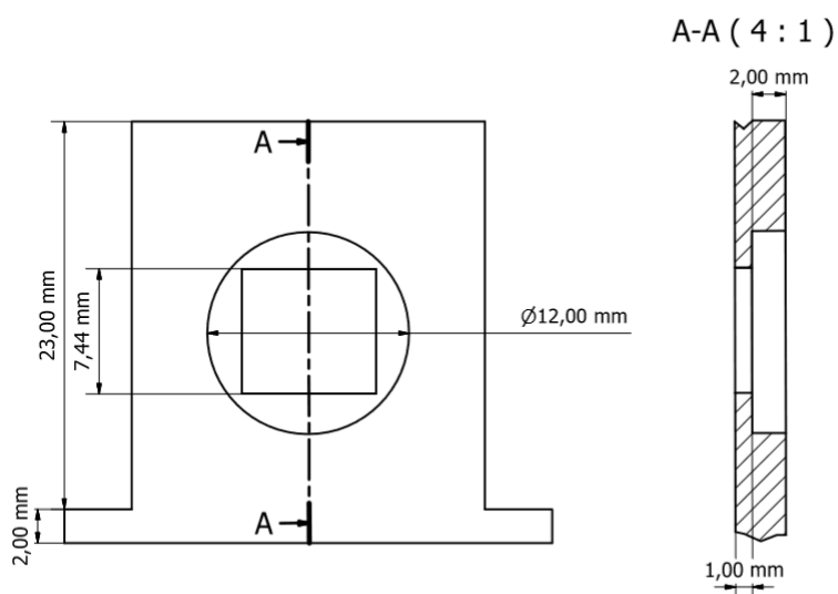
Figura 24 – Gaveta para lentes.
