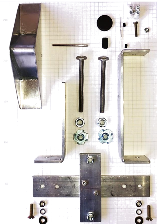
Figura 13: Principais componentes da estrutura interna do pluviômetro.
