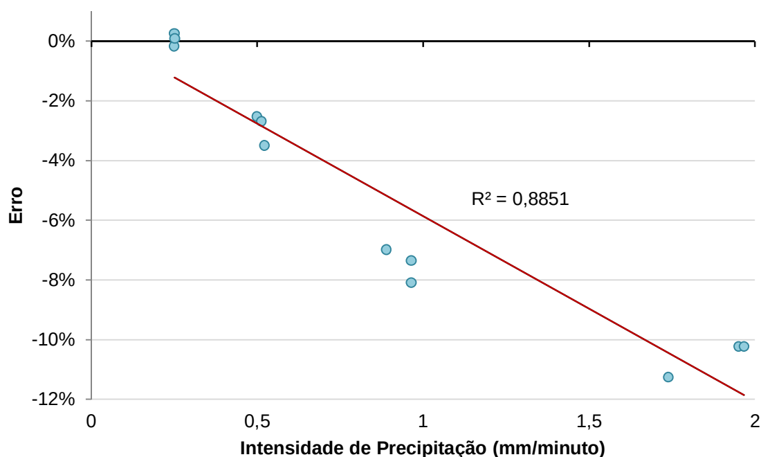
Figura 29: Erro percentual em função da intensidade de precipitação simulada.
