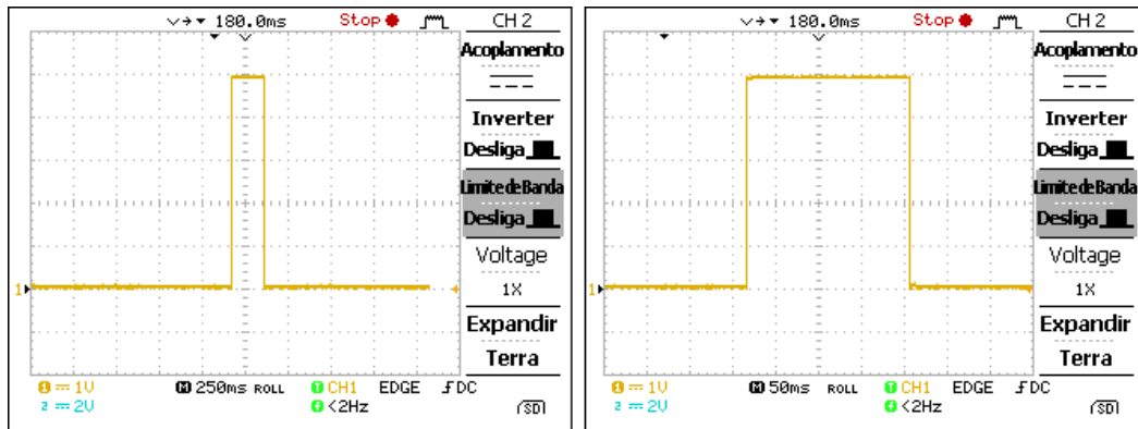
Figura 18: Observação da duração de um pulso rápido.
