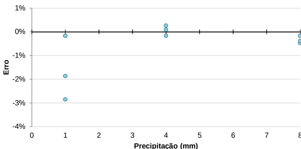
Figura 28: Erro percentual em função do volume precipitado simulado.
