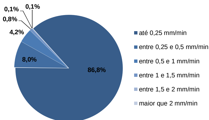
Figura 30: Percentual de ocorrências de determinadas intensidades de chuva em Mossoró.
