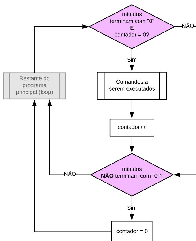
Figura 22: Fluxograma da lógica de execução de comandos por período de tempo.
