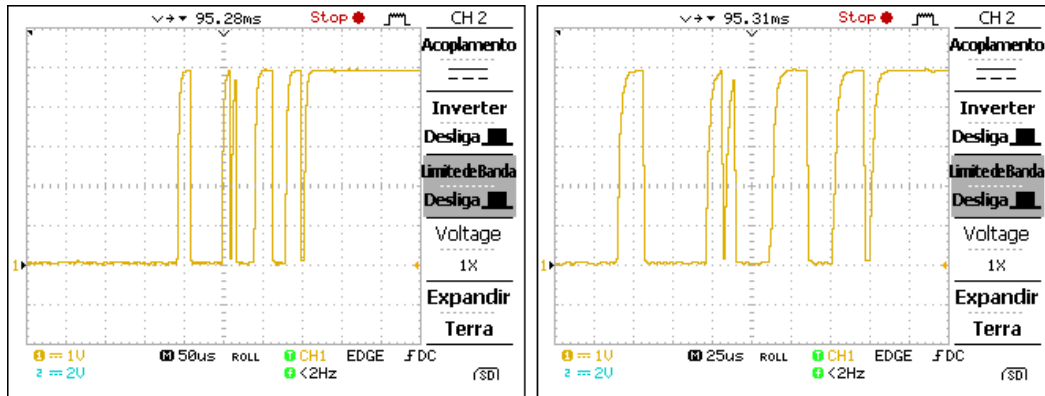
Figura 17: Observação do efeito bouncing no osciloscópio.
