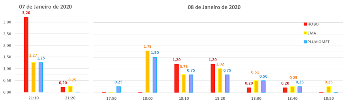
Figura 31: Precipitações registradas no teste em campo.
