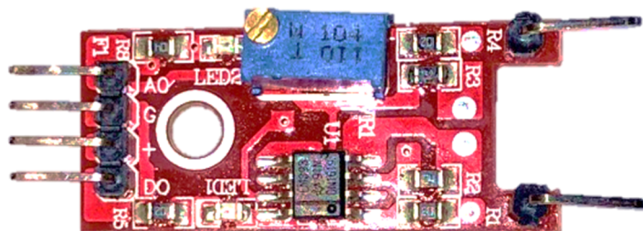
Figura 11: Módulo reed switch (adaptado).
