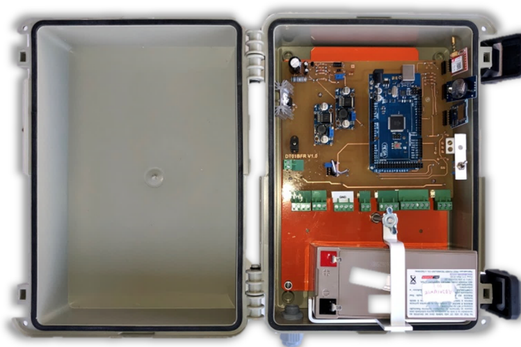
Figura 16: Equipamento de armazenamento e transmissão de dados ( datalogger ) desenvolvido.
