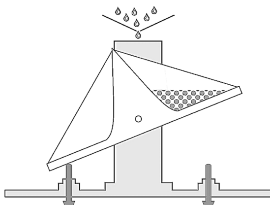
Figura 4: Estrutura interna de um pluviógrafo basculante.
