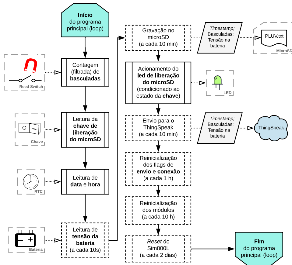
Figura 20: Fluxograma da função loop .
