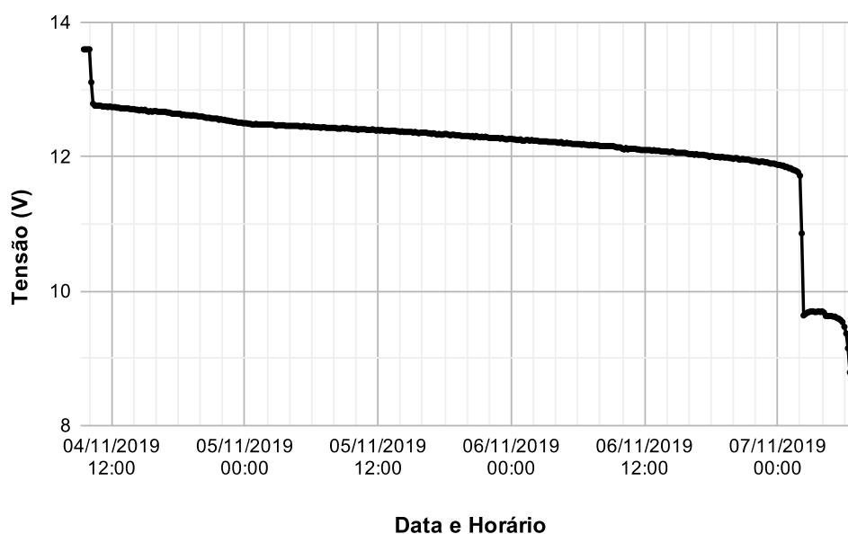
Figura 32: Curva de descarga da bateria estacionária testada.
