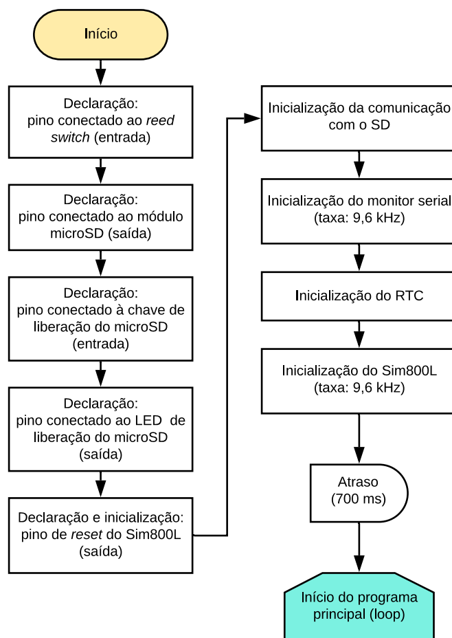
Figura 19: Fluxograma da função setup .
