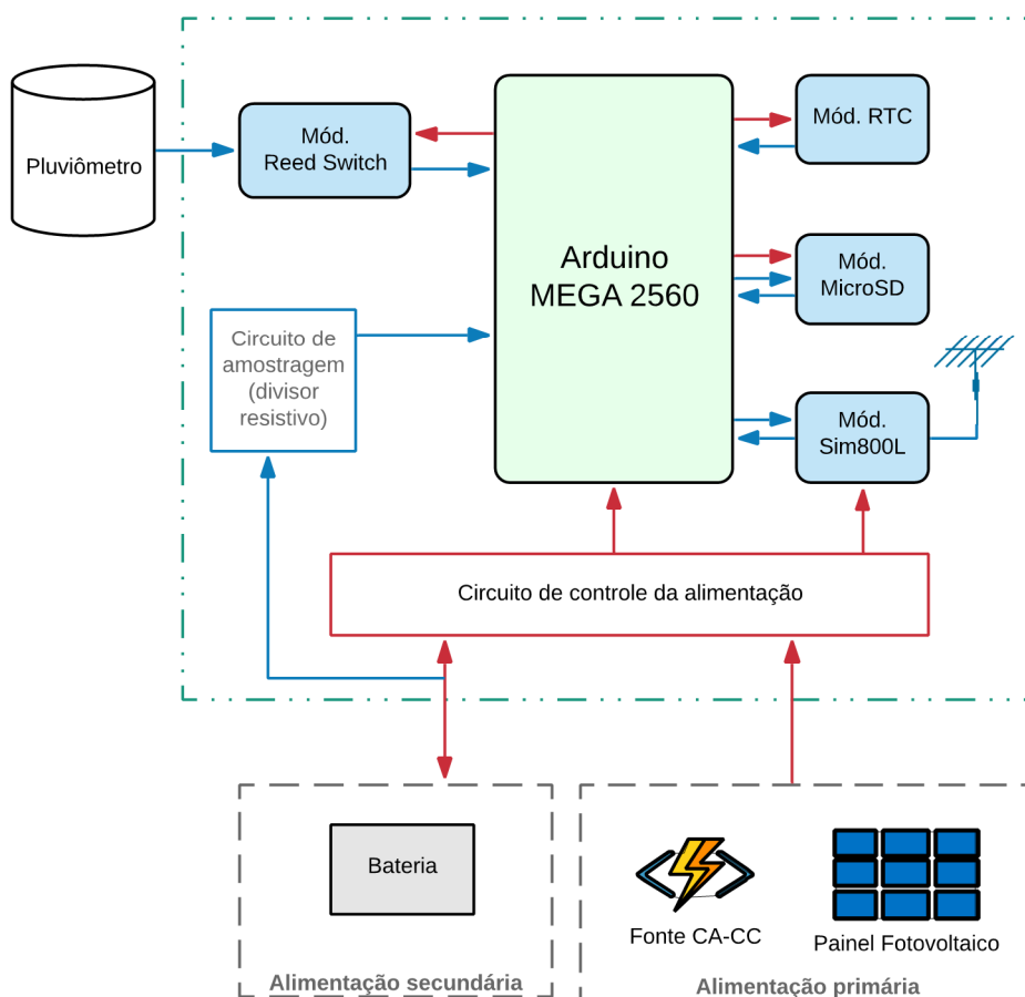
Figura 7: Diagrama de blocos do sistema (representação das partes de hardware).
