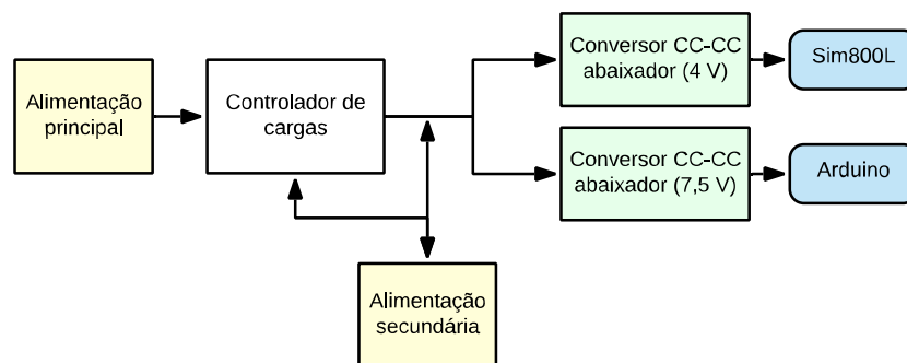
Figura 12: Diagrama de blocos das partes do circuito de alimentação.
