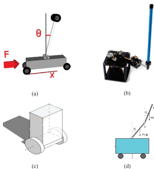
Figura 1: Representação dos diferentes tipos de pêndulos invertidos.
