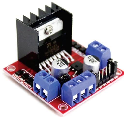
Figura 8: Ponte H L298n.
