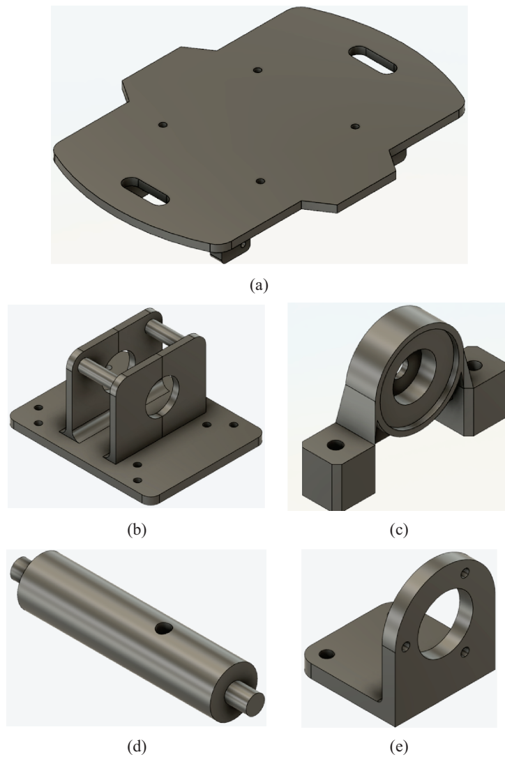
Figura 3: Partes do pendulo invertido: (a) chassi; (b) base superior; (c) suporte para os rolamentos; (d) eixo; (e) suporte para o encoder.
