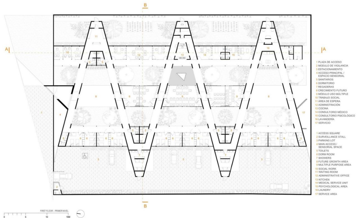
Figura 9 – Planta baixa da edificação.
