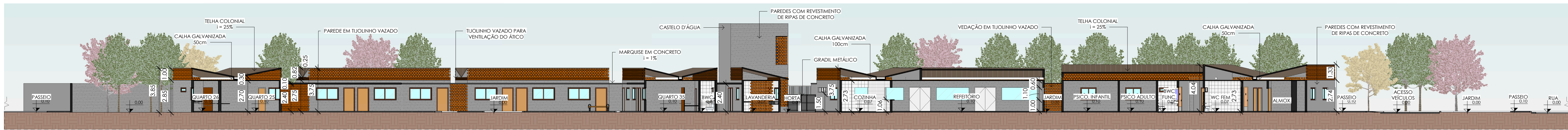
6 CORTE AA 1 : 150
