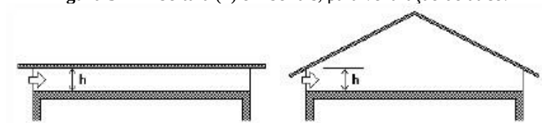
Figura 31 – Abertura (h) em beirais, para ventilação do ático.
