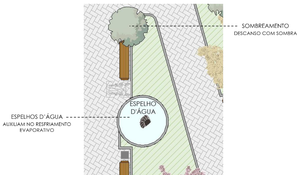
Figura 52 – Estratégias de conforto utilizadas no pátio central.
