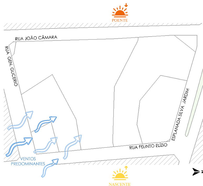
Figura 23 – Insolação e Ventilação no Terreno.
