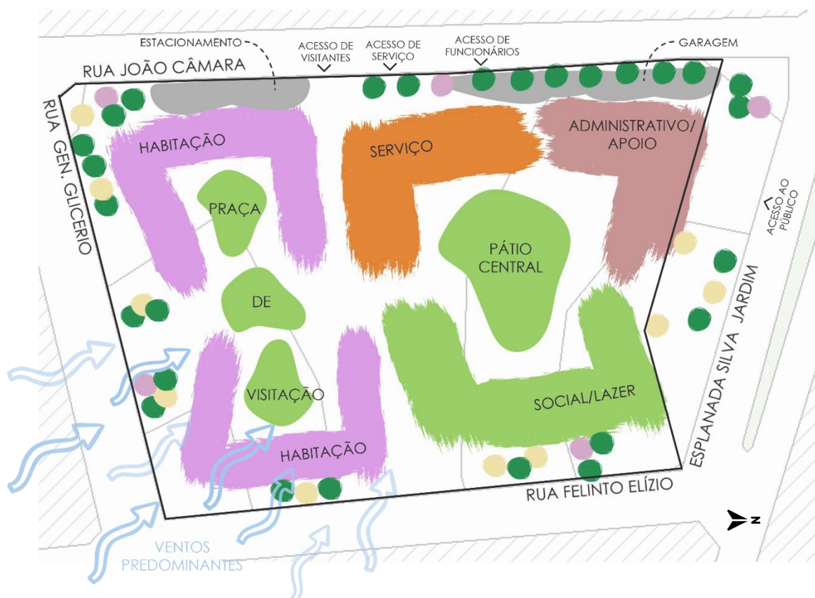
Figura 38 – Zoneamento dos setores do projeto.
