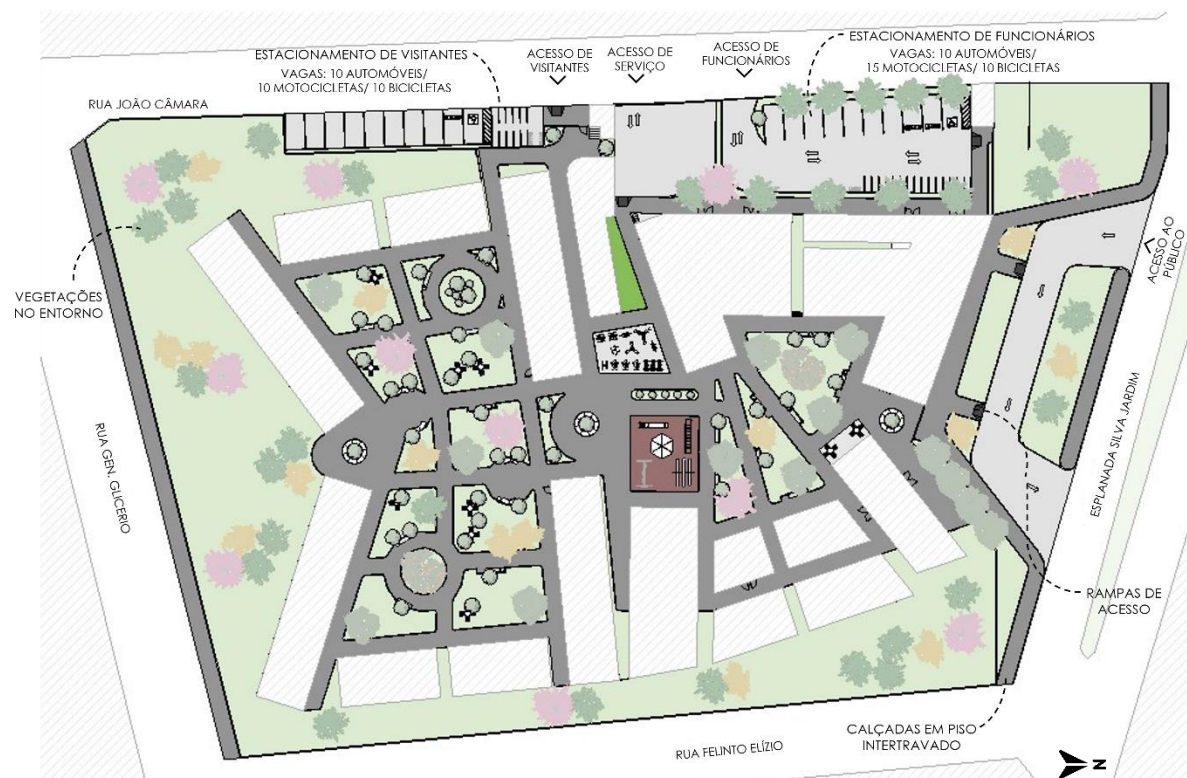
Figura 40 – Implantação destacando os acessos, rampas, calçadas, estacionamentos e vegetações circundantes aos blocos.
