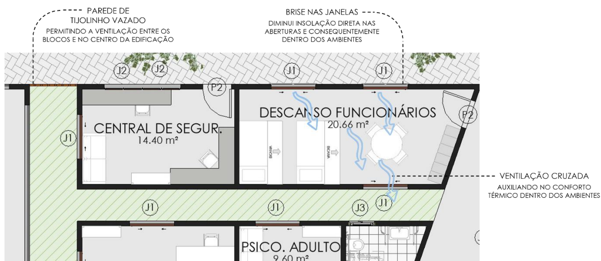
Figura 51 – Estratégias de conforto utilizadas na edificação.
