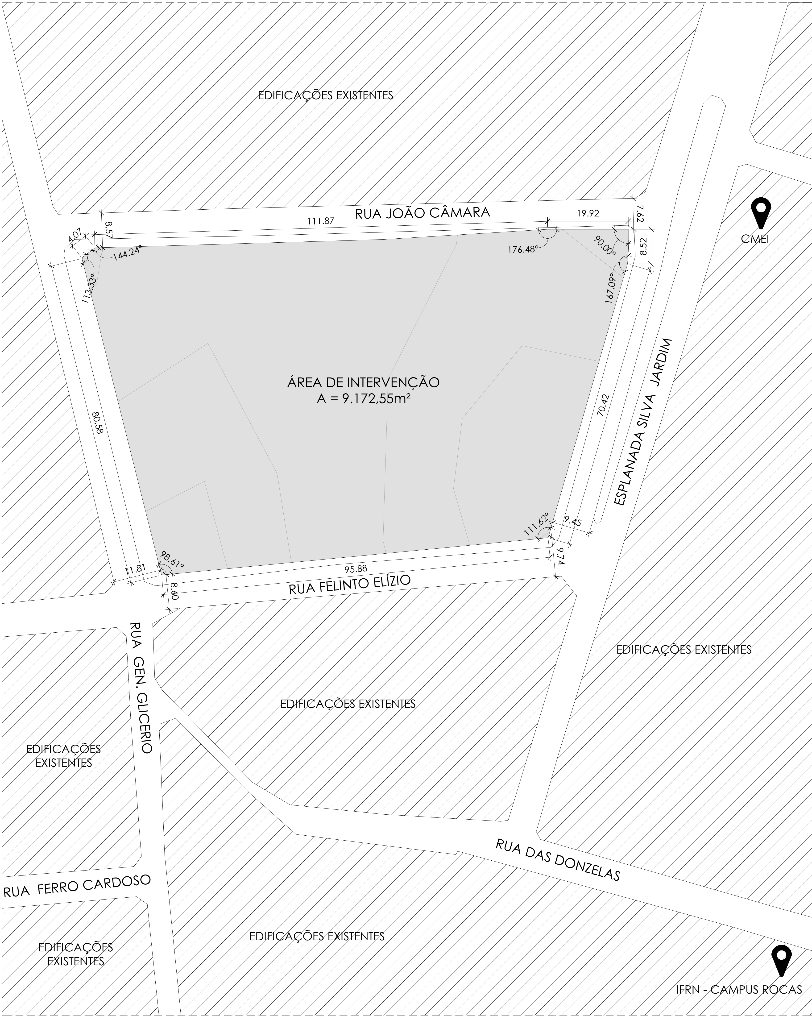
1 PLANTA DE SITUAÇÃO 1 : 400
