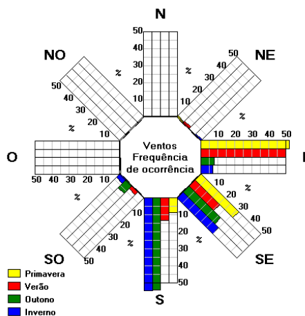
Figura 25 – Rosa dos Ventos de Natal/RN.
