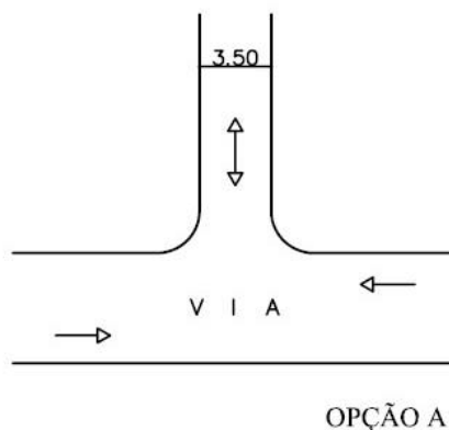
Figura 28 – Opção de acesso para via local.
