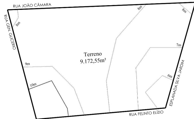
Figura 22 – Curvas de Nível do Terreno.
