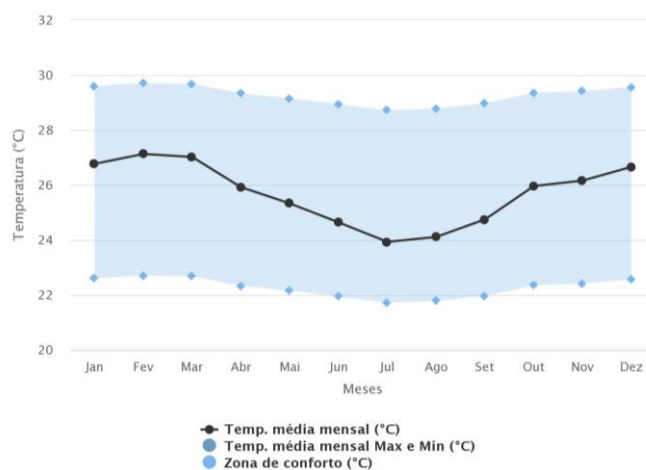
Figura 24 – Gráfico de Temperatura e Zona de Conforto.
