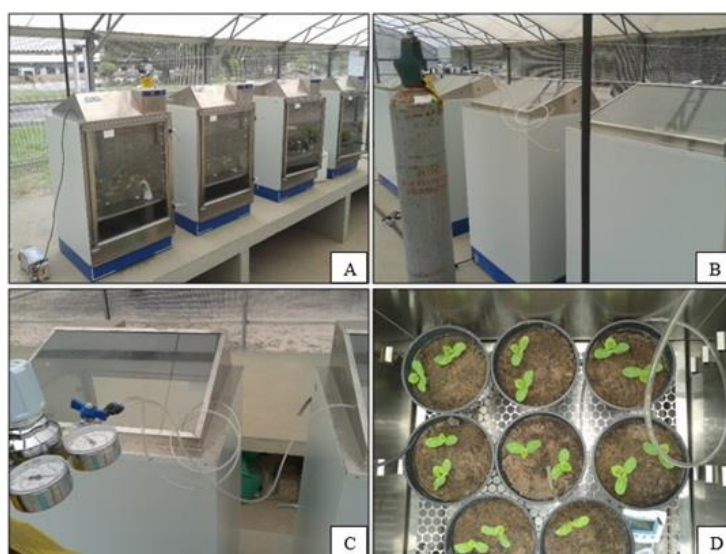
Figura 2 - Câmaras de germinação com sistema adaptado para temperatura e injeção de CO 2 (A; B; C e D).
