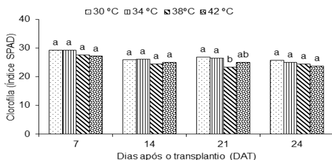
Figura 3 - Índice de clorofila em folhas de meloeiro em função das diferentes temperaturas aos 7; 14; 21 e 24 DAT.
