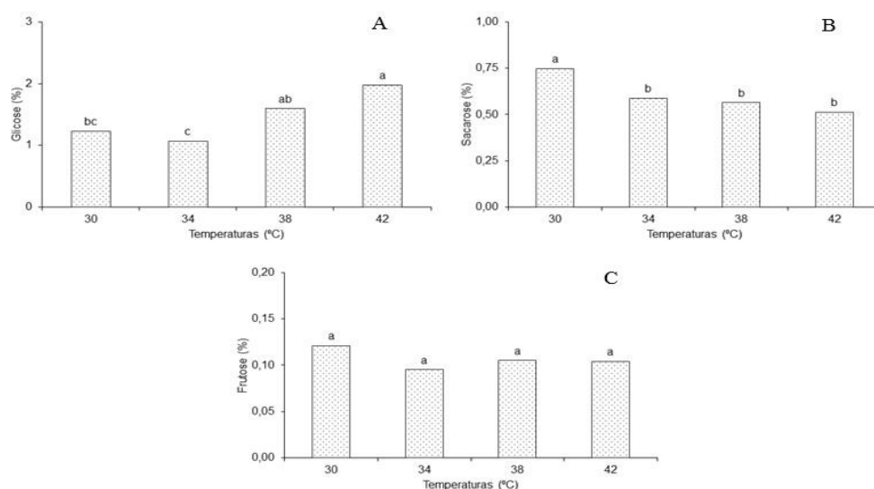
Figura 7 - (A) Porcentagem de glicose, (B) sacarose e (C) de frutose em função das diferentes temperaturas aos 24 DAT.
