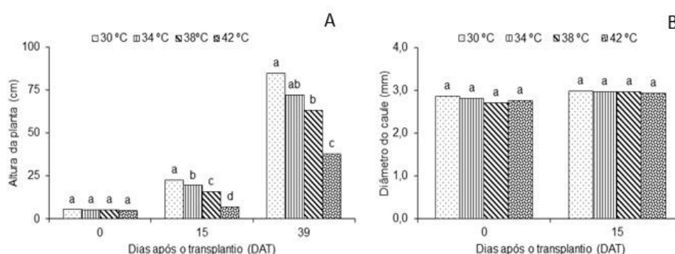
Figura 3 - (A) Altura da planta aos 0; 15 e 39 DAT e (B) diâmetro do caule do meloeiro aos 0 e 15 DAT em função das diferentes temperaturas.
