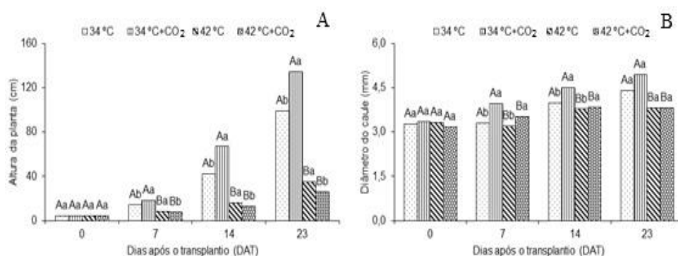
Figura 3- (A) Altura da planta e (B) diâmetro do caule do meloeiro aos 0; 7; 14 e 23 DAT em função das diferentes temperaturas e concentrações de CO 2 .
