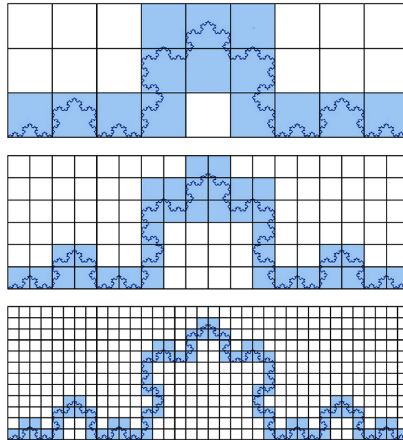
Figura 14 - Técnica da contagem de caixas em várias escalas.
