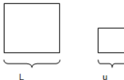
Figura 6 - Quadrado de lado medindo L e quadrado de lado medindo u .
