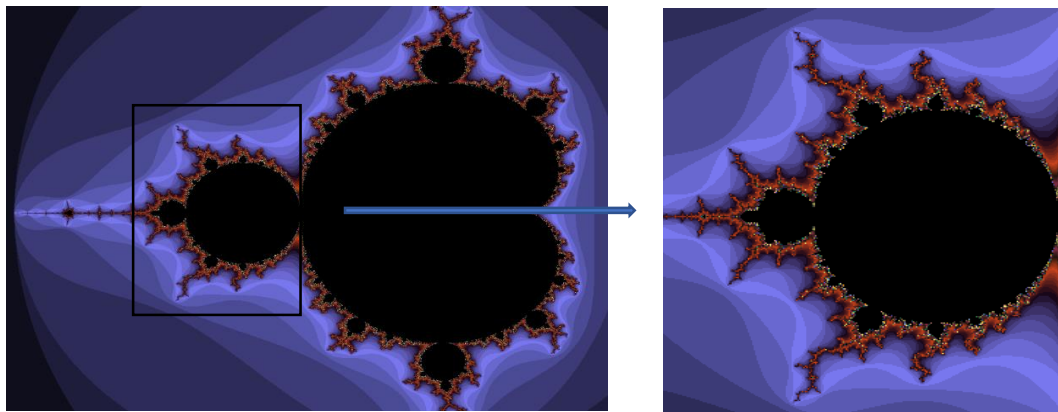
Figura 3 - Autossemelhança aproximada no Conjunto de Mandelbrot
