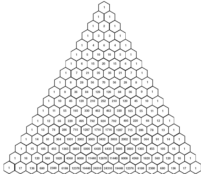
Figura 3: Triângulo de Pascal 2. 15
