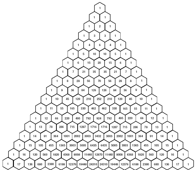
Figura 5: Triângulo de Pascal 2. 17
