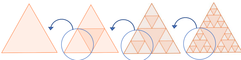
Figura 4 - Autosemelhança exata no Triângulo de Sierpinski
