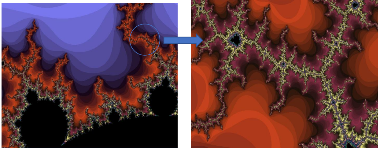
Figura 9 - Estrutura fina no Conjunto de Mandelbrot.
