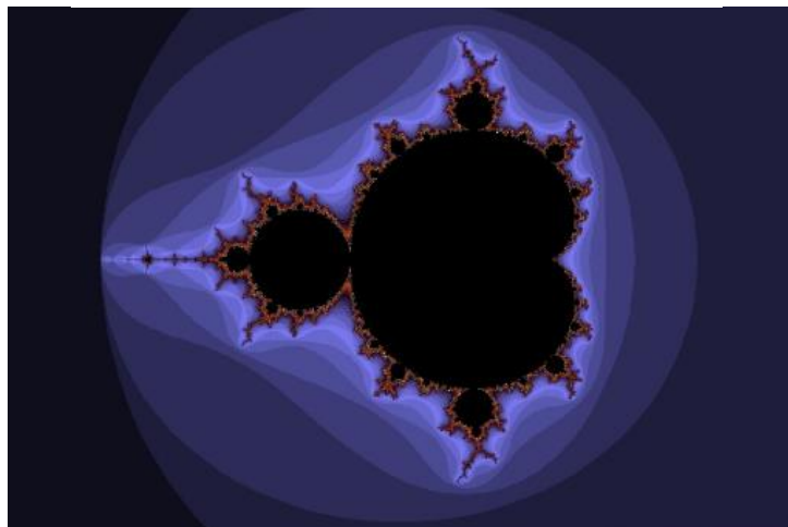
Figura 1 - O conjunto de Mandelbrot
