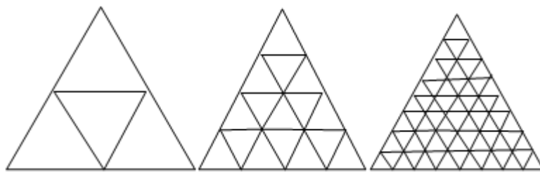
Figura 2: Triângulo de Sierpinski. 14
