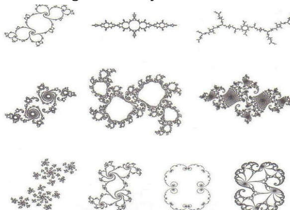
Figura 2 - Conjunto de Julia
