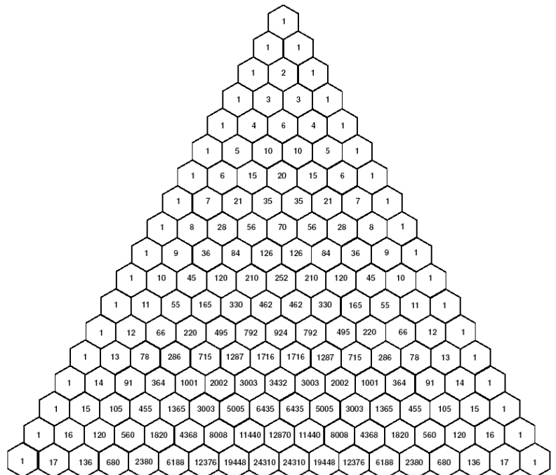
Figura 4: Triângulo de Pascal 2. 16
