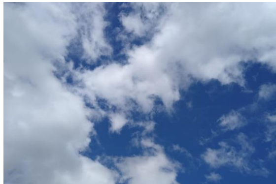
Figura 11 - Fractais na natureza - Nuvens.
