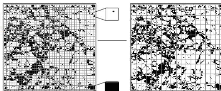
Figura 15 - Técnica Box-counting aplicada à análise do solo.
