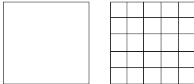
Figura 8 - Quadrado inicial a ser dimensionado e uma cópia com lado dividido em cinco pedaços iguais.
