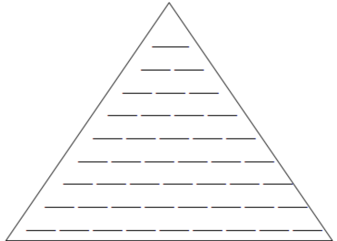
Figura 17: Construção do Triângulo de Pascal. 13
