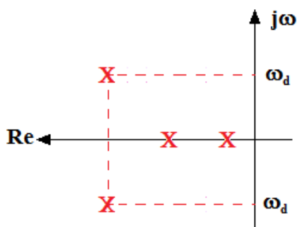
Figura 3.11 – Caso III.c: diagrama de pólos de um sistema de quarta ordem com um par complexo conjugado próximo a origem.
