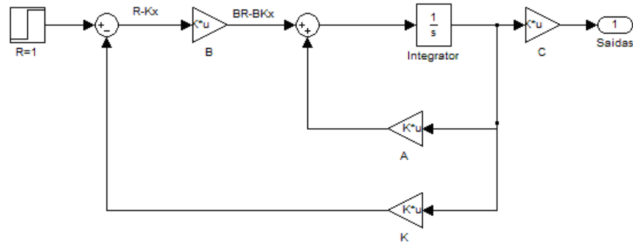
Figura 3.6 – Diagrama de blocos de um sistema em espaço de estados em malha fechada.
