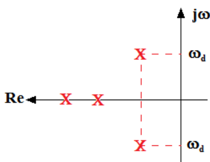
Figura 3.9 – Caso III.a: diagrama de pólos de um sistema de quarta ordem com um par complexo conjugado próximo a origem.
