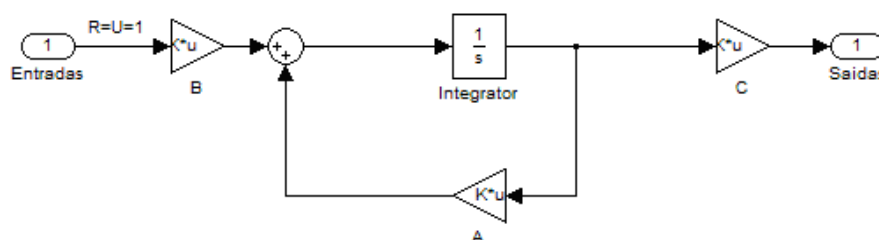
Figura 3.5 – Diagrama de blocos de um sistema em espaço de estados em malha aberta.
