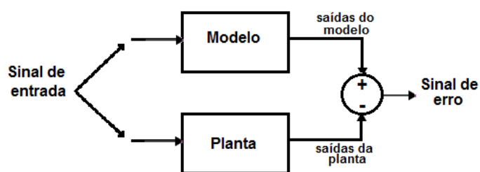
Figura 3.3 - Monitoramento das saídas e cálculo de erro.
