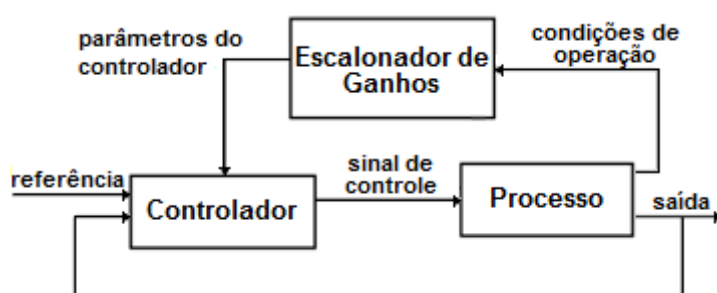
Figura 2.4 – Diagrama de blocos de um sistema de controle por escalonamento de ganhos.
