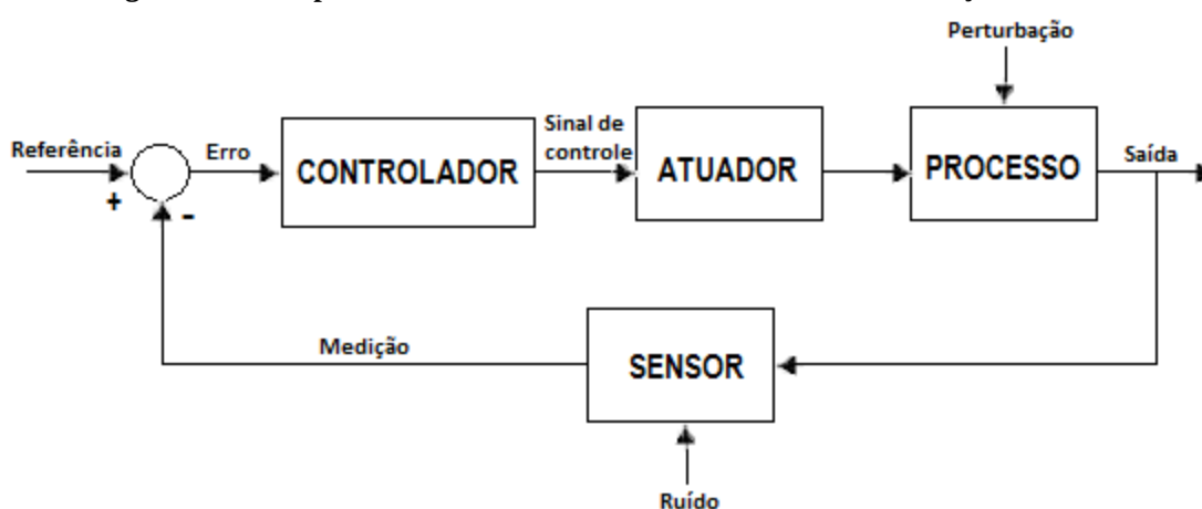
Figura 1.1 - Componentes de um sistema de controle com realimentação de saída.
