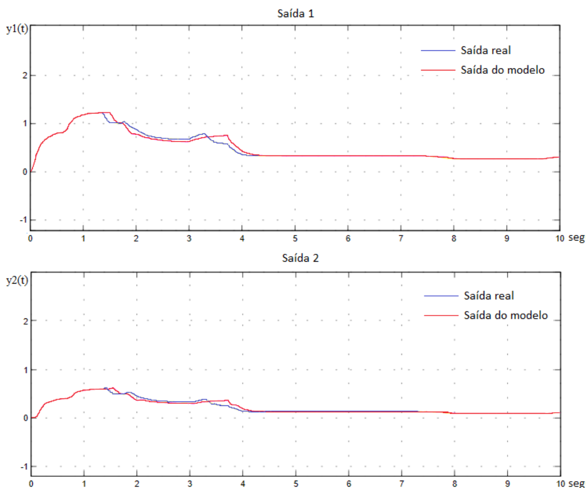
Figura 4.1.a – Saídas do sistema real e saídas do modelo estimado.
