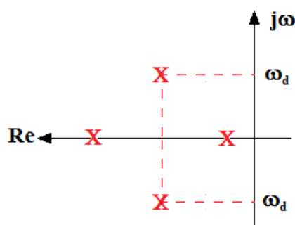
Figura 3.10 – Caso III.b: diagrama de pólos de um sistema de quarta ordem com um par complexo conjugado situado entre os pólos reais.
