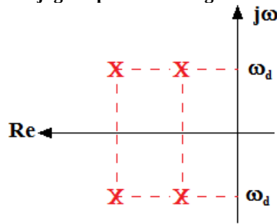
Figura 3.8 – Caso II.a: diagrama de pólos de um sistema de quarta ordem com um par complexo conjugado próximo a origem.
