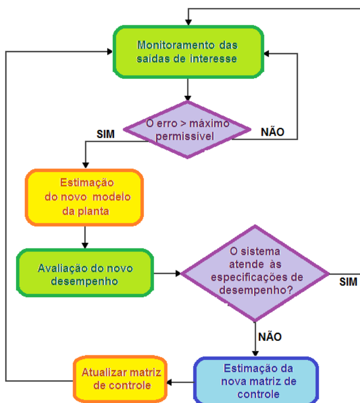
Figura 3.2 - Etapas do controle adaptativo proposto.
