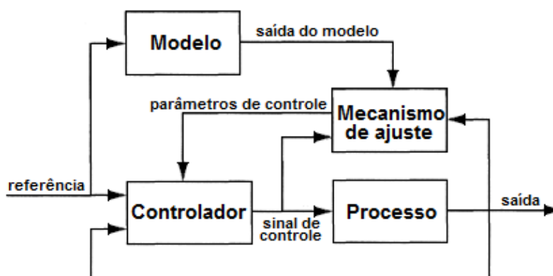
Figura 2.5 – Diagrama de blocos de um controlador adaptativo por modelo de referência.
