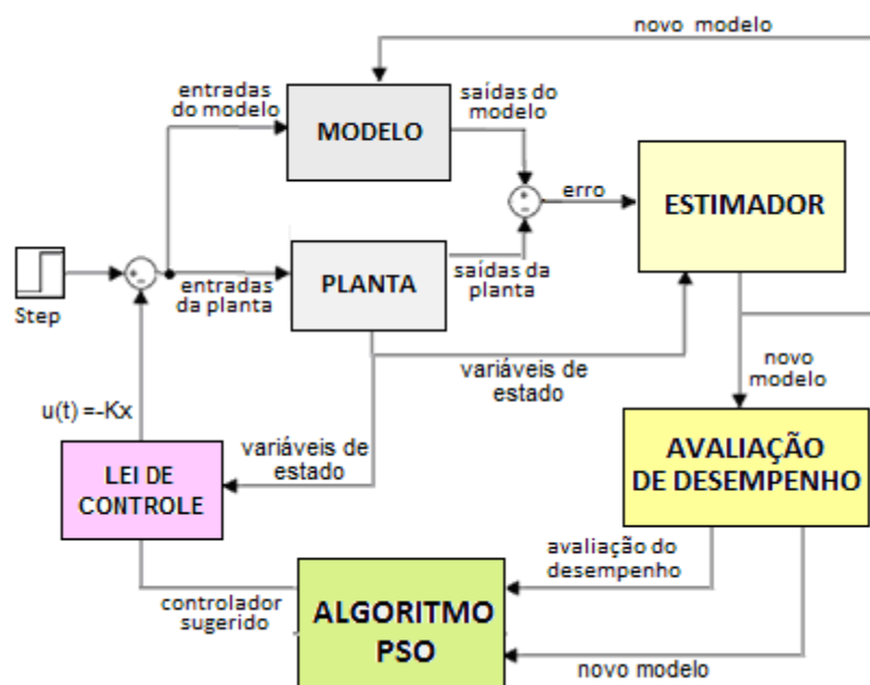
Figura 3.1 – Diagrama de blocos para o sistema de controle adaptativo proposto.
