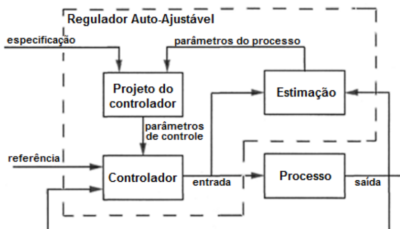
Figura 2.6 – Diagrama de blocos de um Regulador auto-ajustável.
