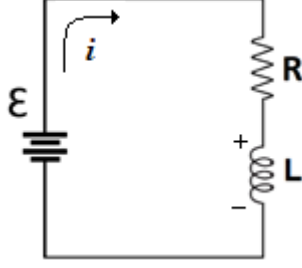
Figura 7 – Circuito RL e fonte ( \mathcal{E} ).
