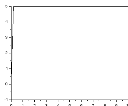
Figura 6 – Solução com séries de potências para Eq. 26.
