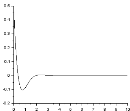
Figura 13 – Solução analítica para Eq. 43.
