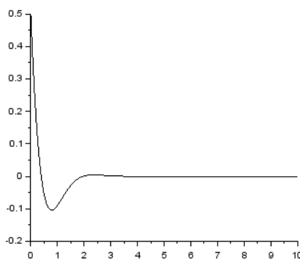
Figura 14 – Solução com Runge-kutta para Eq. 43.
