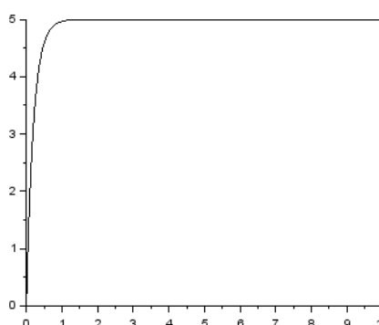
Figura 5 – Solução com Runge-Kutta para Eq. 26.
