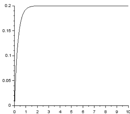
Figura 10– Solução com Runge-Kutta para Eq. 34.
