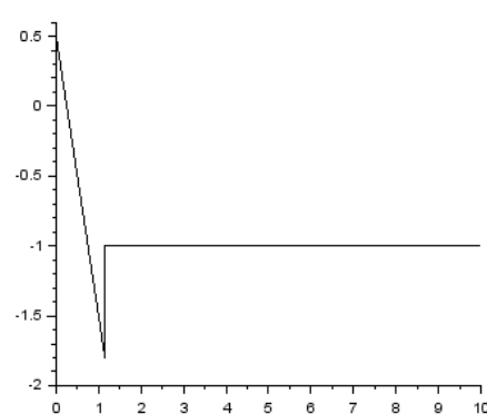
Figura 15 – Solução com série de potências para Eq. 43.
