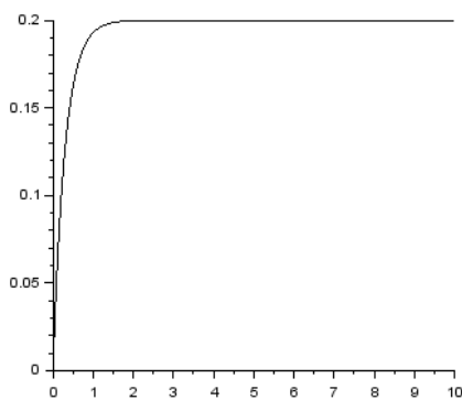
Figura 9 – Solução analítica para Eq. 34.
