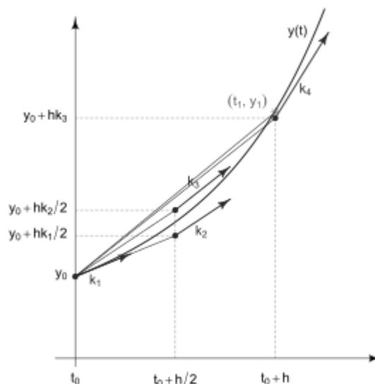
Figura 1 – Visão Geométrica do Método de Runge Kutta de 4ª Ordem.
