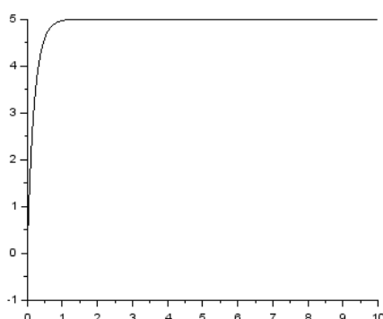
Figura 4 – Solução analítica para Eq. 26.
