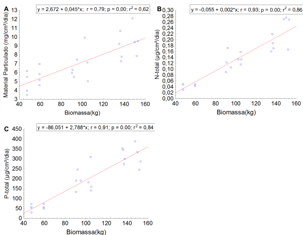
Figura 3. Correlação entre a biomassa de tilápia e as taxas de sedimentação de material particulado (A); nitrogênio total (N-total) (B); fósforo total (P-total) (C).
