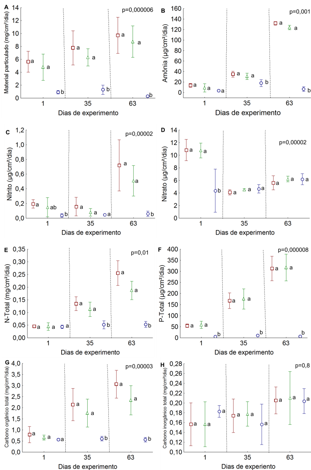
Figura 2. Valores médios e desvios padrão das taxas de sedimentação de: A) material particulado; B) amônia; C) nitrito; D) nitrato; E) nitrogênio total; F) fósforo total; G)
