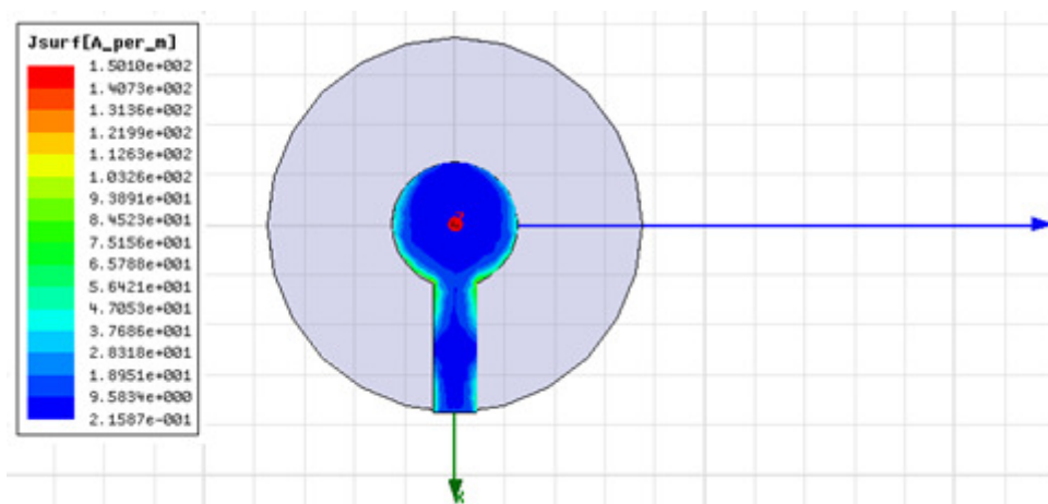
Figura 30 – Densidades de correntes e campos radiados da antenna simulada.
