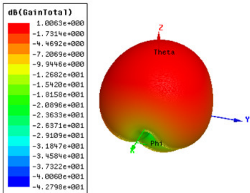
Figura 29 – Diagrama de radiação em 3D da antenna simulada
