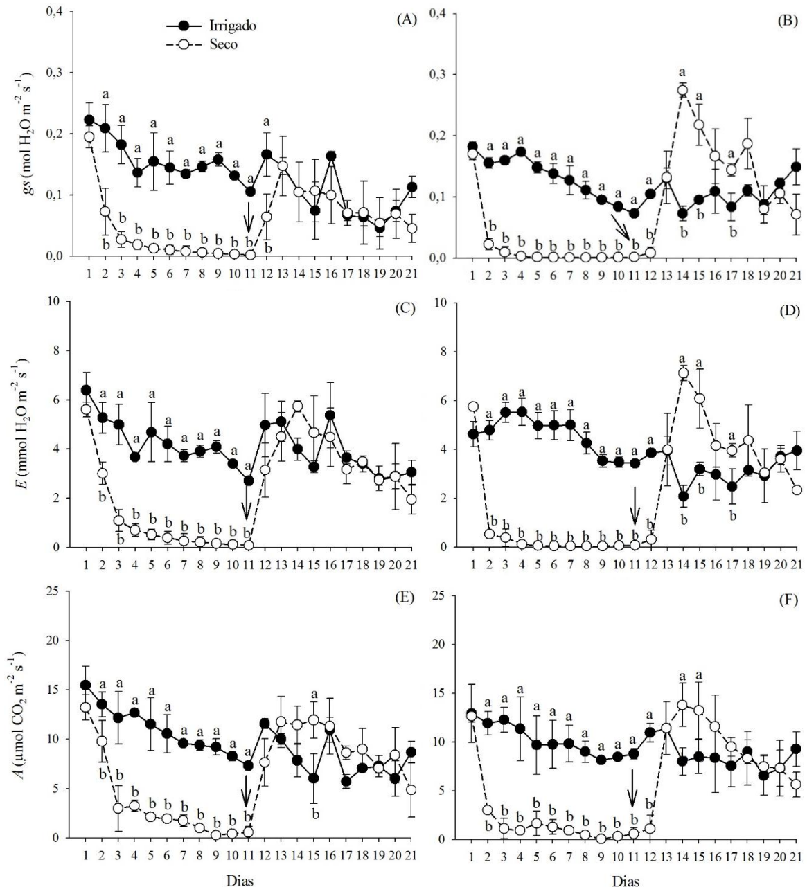
Gráfico 13. Condutância estomática ( g_s ), transpiração ( E ) e taxa fotossintética líquida ( A ) de Commelina benghalensis em monocultivo (A; C; E) e em interação (B; D; F) com feijão-caupi, submetida ao déficit hídrico (Seco) ou não (Irigado). As setas indicam o momento da retomada da irrigação. As barras de erro indicam intervalo de confiança da média a 95%. Mossoró/RN, 2017.
