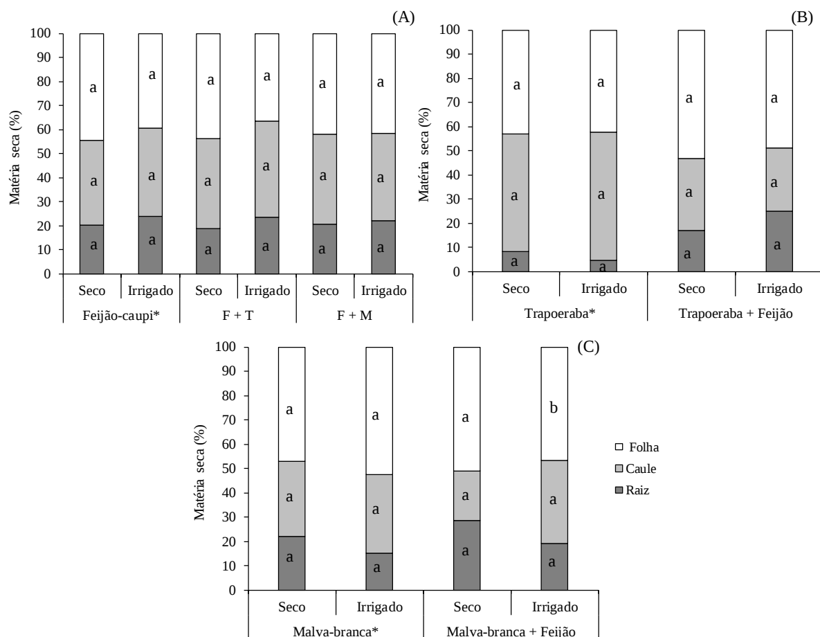
Gráfico 1. Partição de matéria seca de feijão-caupi (A), Commelina benghalensi (B) e Waltheria indica (C), em situação de competição, submetidos ao déficit hídrico (Seco) ou não (Irigado). Médias seguidas pela mesma letra, em cada variável (órgão da planta), não diferem entre si pelo teste t a 5% de probabilidade; *=Plantas cultivadas sem interação. Mossoró/RN, 2017.
