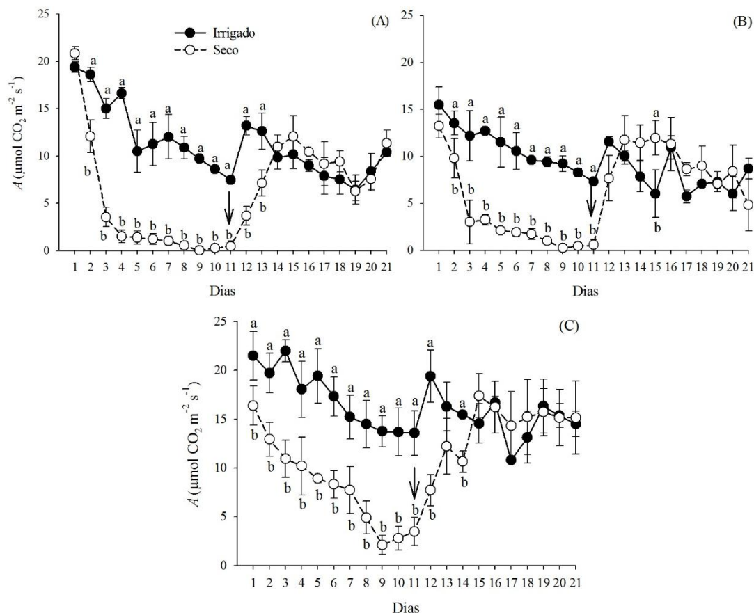
Gráfico 5. Taxa fotossintética líquida (A) de feijão-caupi (A) Commelina benghalensis (B) e Waltheria indica (C), cultivados sem interação, submetidos ao déficit hídrico (Seco) ou não (Irigado). As setas indicam o momento da retomada da irrigação. As barras de erro indicam intervalo de confiança da média a 95%. Mossoró/RN, 2017.
