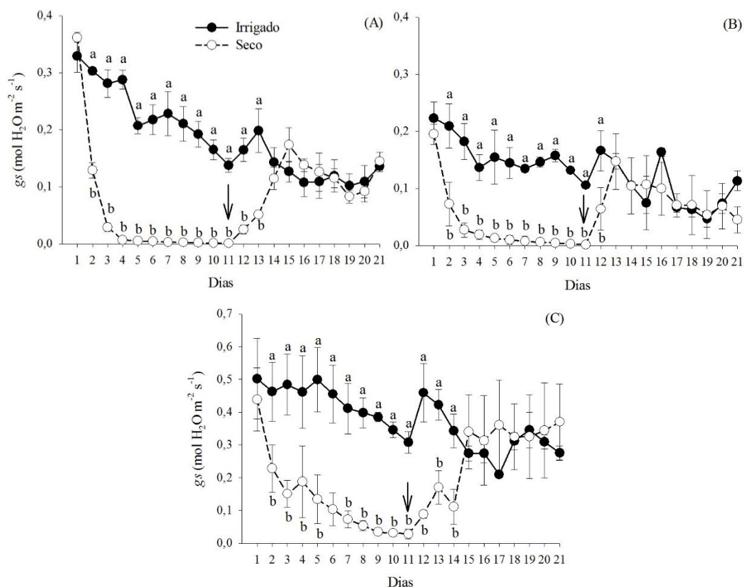
Gráfico 3. Condutância estomática ( gs ) de feijão-caupi em (A) Commelina benghalensis (B) e Waltheria indica (C), cultivados sem interação, submetidos ao déficit hídrico (Seco) ou não (Irigado). As setas indicam o momento da retomada da irrigação. As barras de erro indicam intervalo de confiança da média a 95%. Mossoró/RN, 2017.
