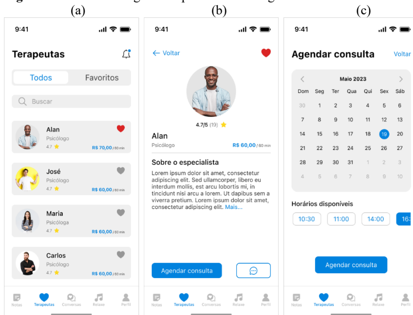
Figura 3 - Telas de listagem dos profissionais e agendamento de consulta.
