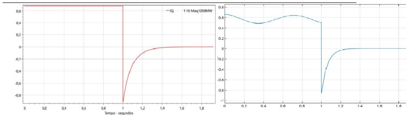
Figura 7 - Corrente de eixo de quadratura. (Autoria própria)
