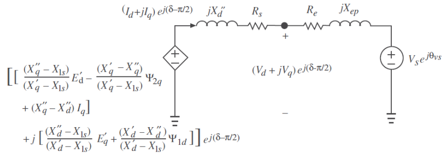
Figura 3. Circuito sub-trânsitório da máquina síncrona. [7]
