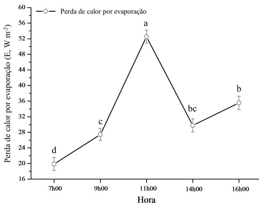
Figura 7. Perda de calor por evaporação em cutias ( Dasyprocta leporina ). Médias seguidas por letras iguais não diferem entre si pelo teste de Tukey-Krammer ( P > 0,05 ).
