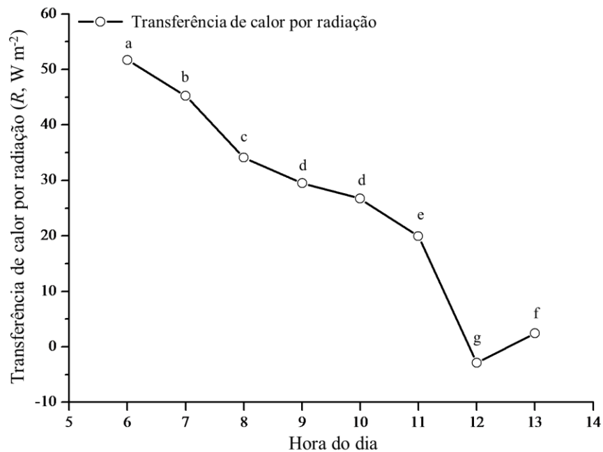
Figura 15. Perda de calor por radiação ( R , W m^{-2} ) em preás ( Galea spixii ). Médias seguidas pela mesma letra não diferem entre si pelo teste de Tukey-Krammer ( P > 0,05 ).
