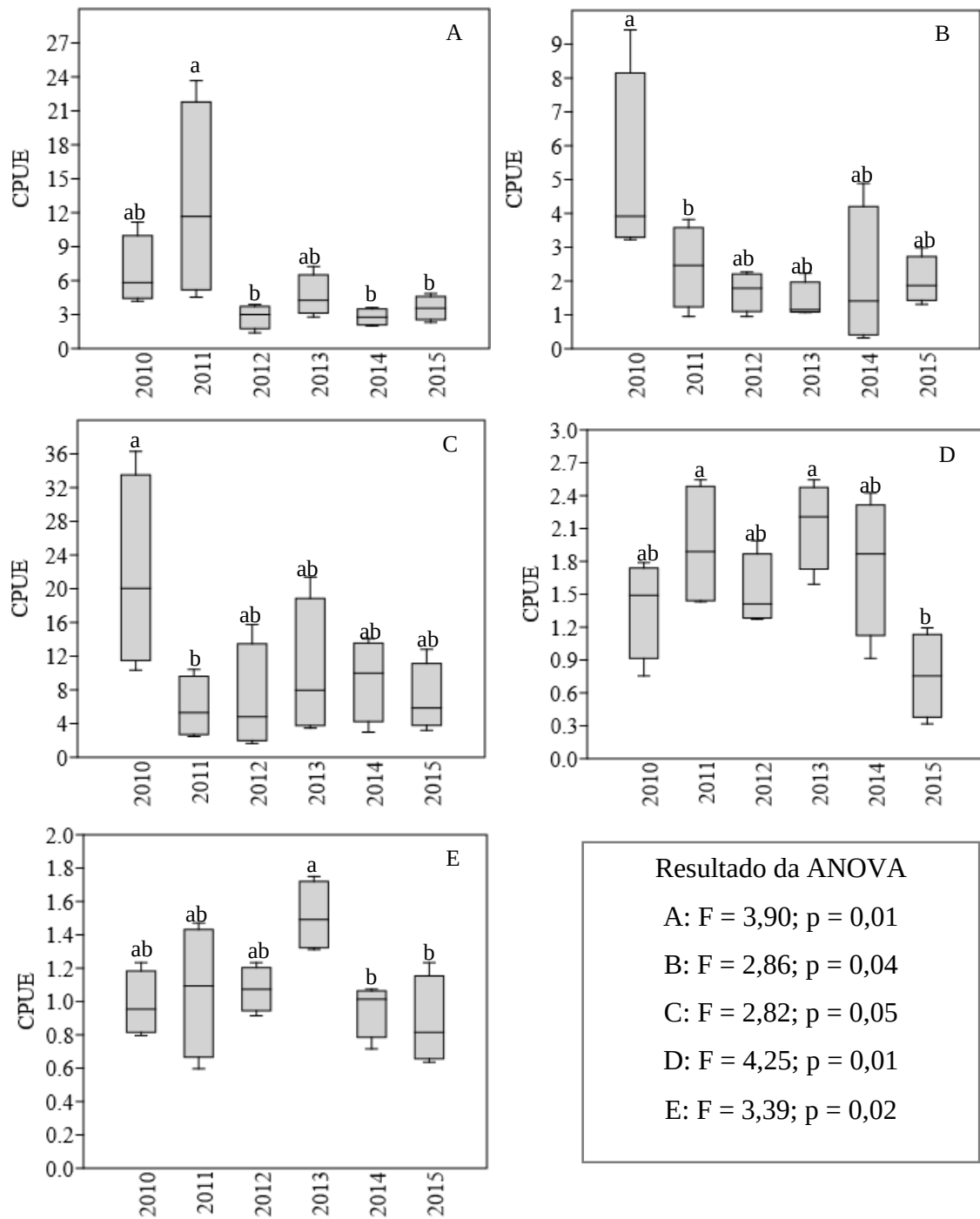
Figura 4 – Variação anual da CPUE das guildas tróficas de peixes entre período de 2010 e 2015, no reservatório de Santa Cruz, Brasil. A – Detritívora, B – Carcinófaga, C – Insetívora, D – Onívora, E - Piscívora. A mediana é mostrada com uma linha horizontal dentro da caixa. Os valores mínimos e máximos são mostrados com linhas horizontais curtas. Letras diferentes indicam diferenças estatísticas (Tukey, p < 0,05 ).
