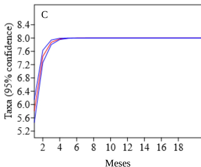
Figura 2 – Curva de acumulação de espécies (linha vermelha), intervalos de confiança de 95% (linha azul) para os reservatórios de Santa Cruz (A); Umari (B); Pau dos Ferros (C), da bacia hidrográfica do rio Apodi/Mossoró, Rio Grande do Norte, Brasil.
